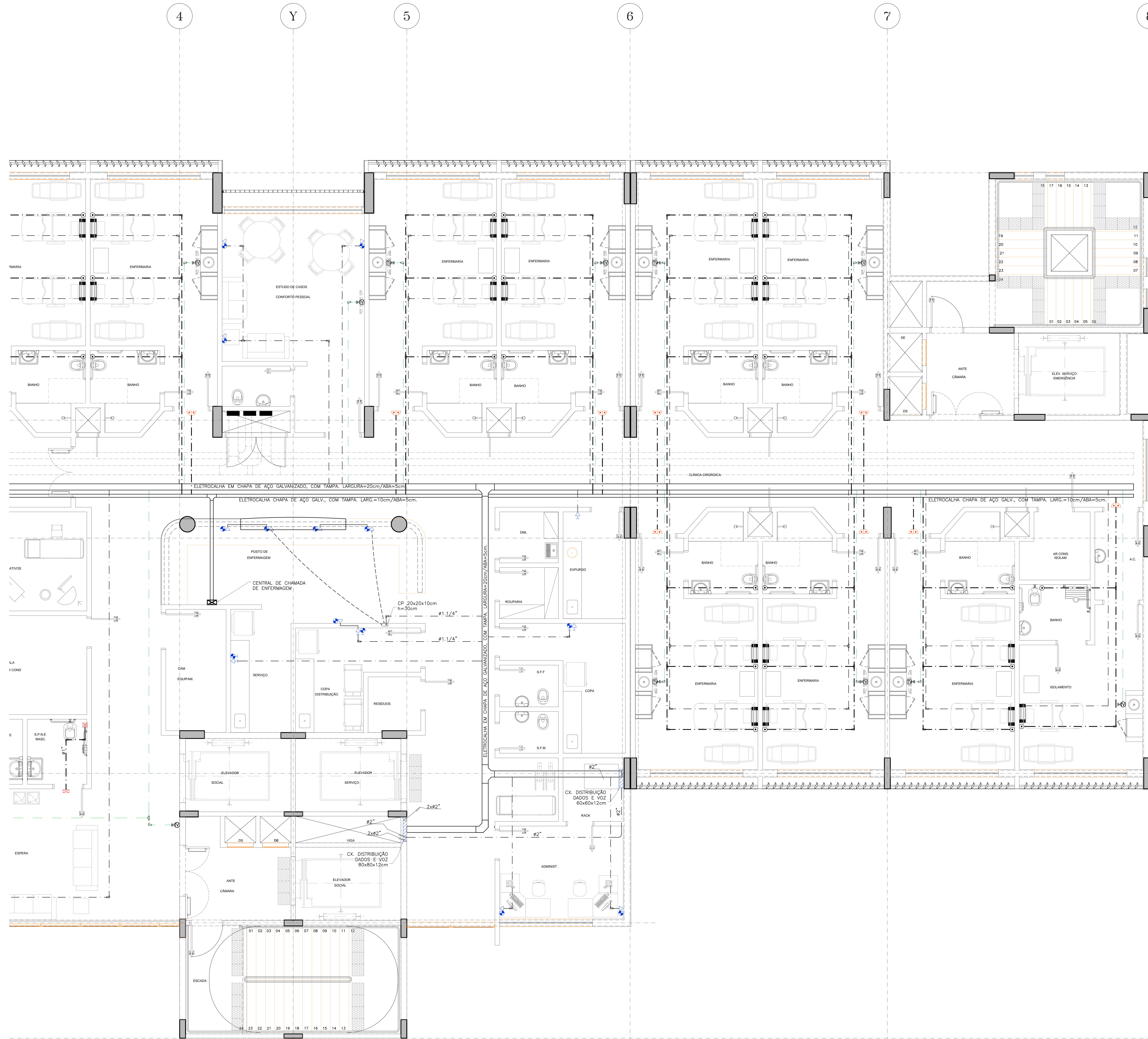
PLANTA 4º PAVTº - PARTE 2 ESC. 1:50
