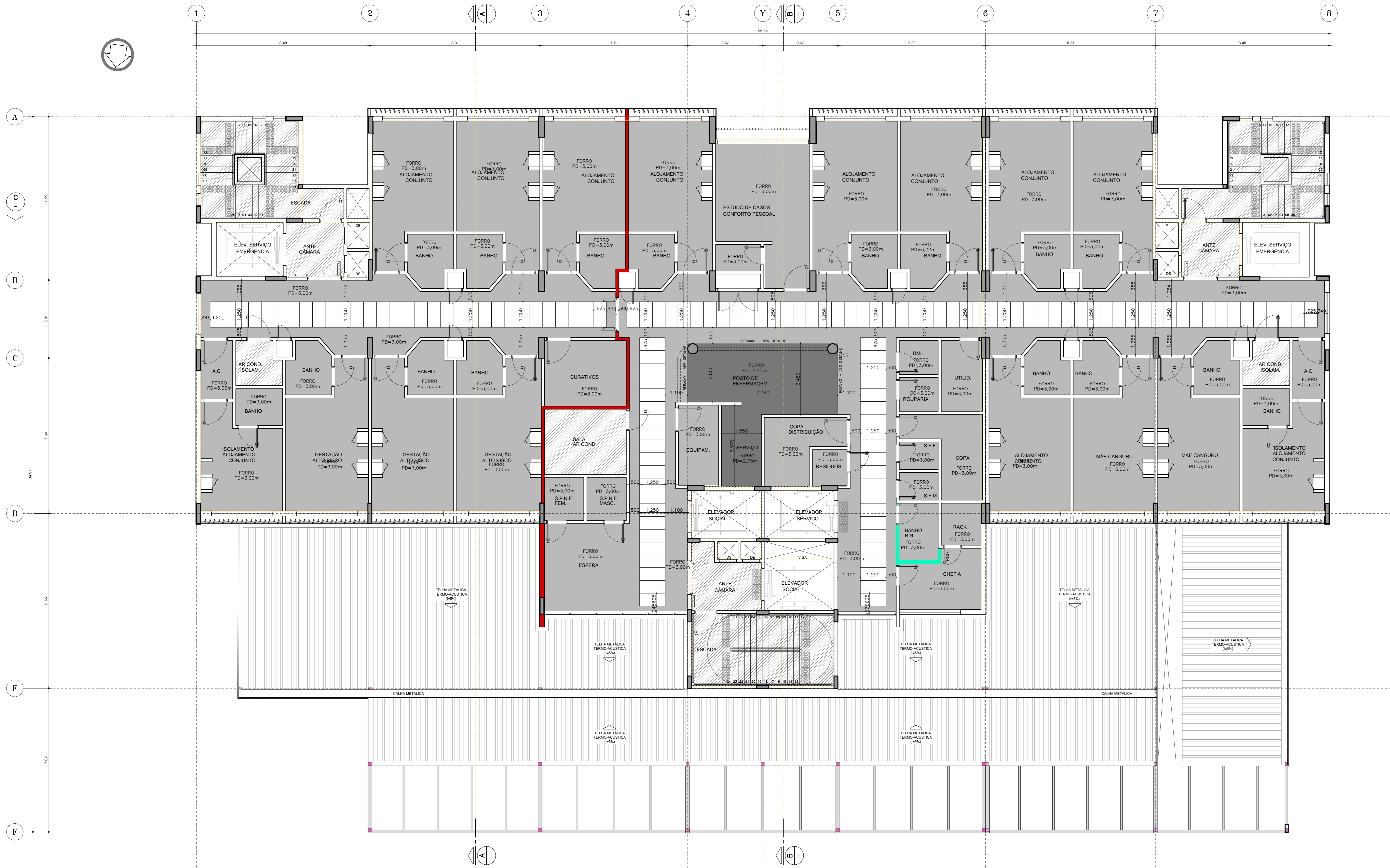
PAGINAÇÃO DE FORRO - 3º PAVIMENTO ESC. 1:75
