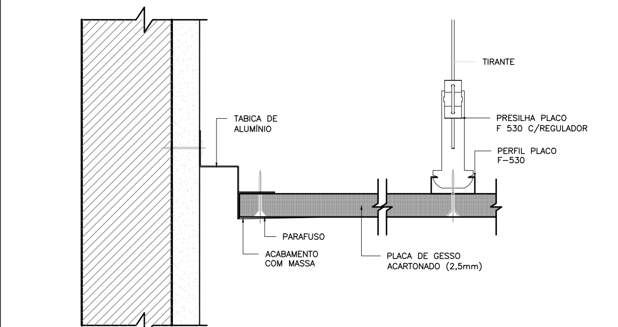
DETALHE TABICA FORRO DE GESSO ESC. 1:2 MEDIDAS CM
