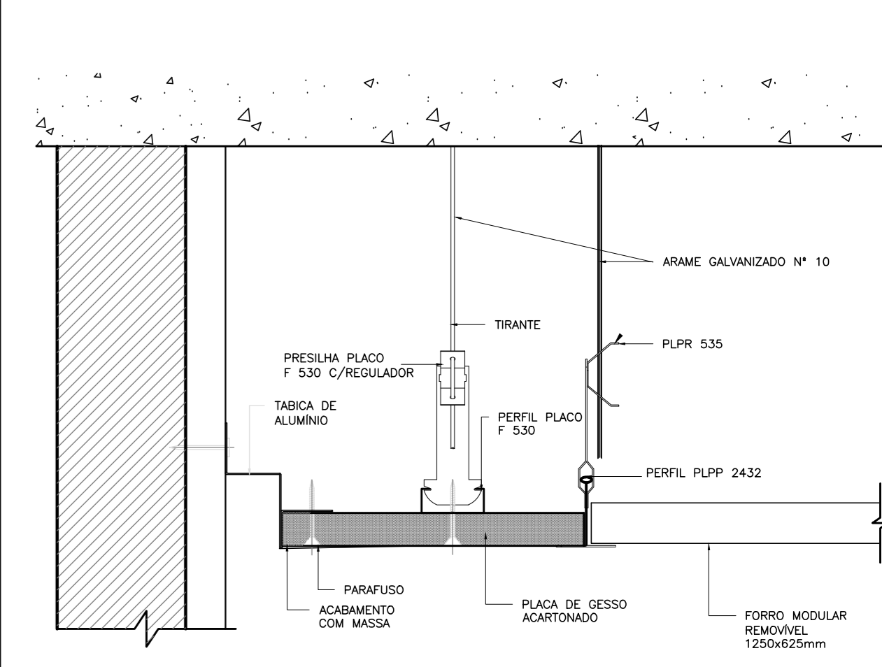
DETALHE ARREIMATE FORRO DE GESSO / FORRO REMOVIVEL ESC. 1:2 MEDIDAS CM
