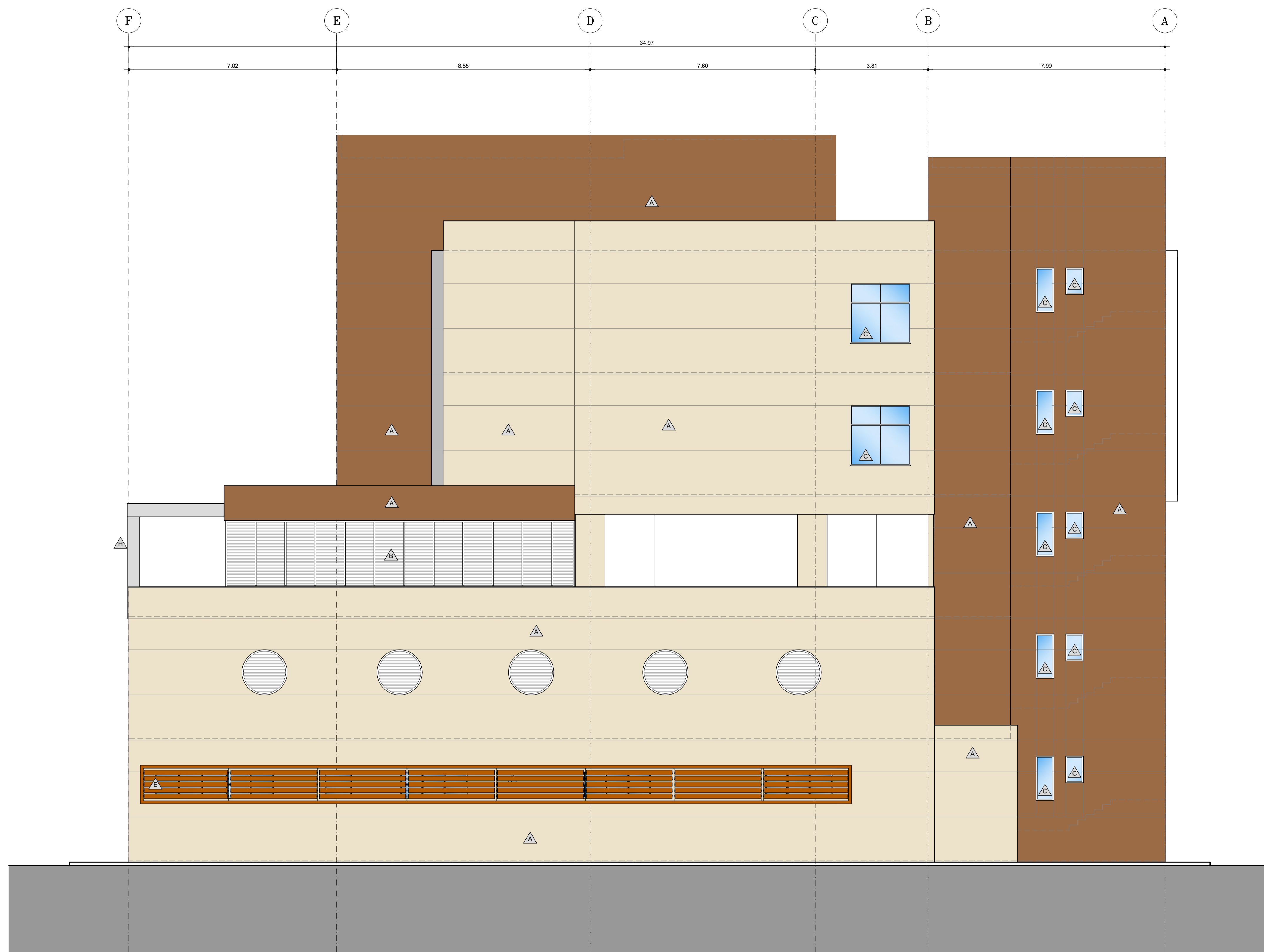
ELEVAÇÃO 04 ESC. 1:75
