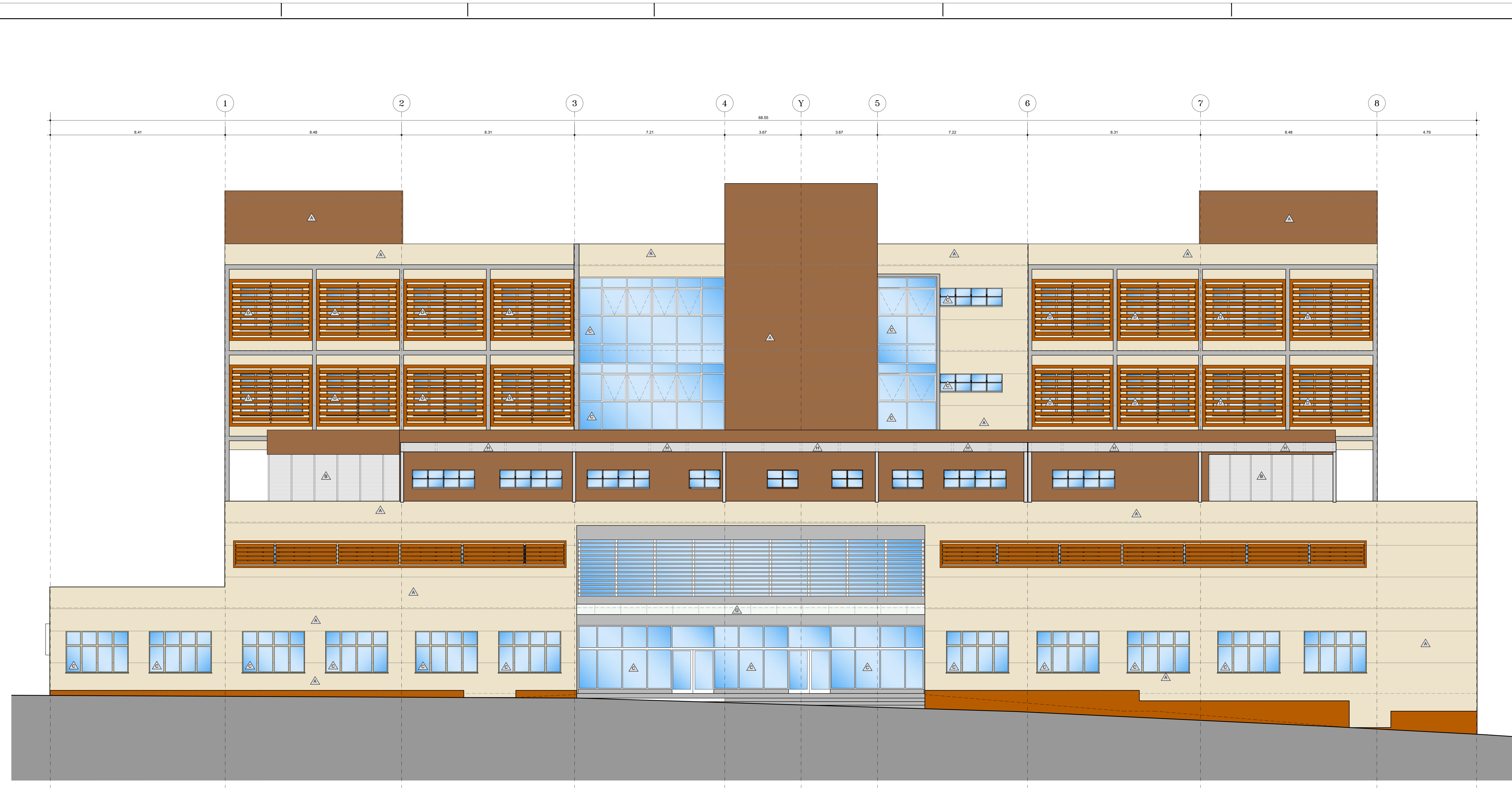
ELEVAÇÃO 01 ESC. 1:75
