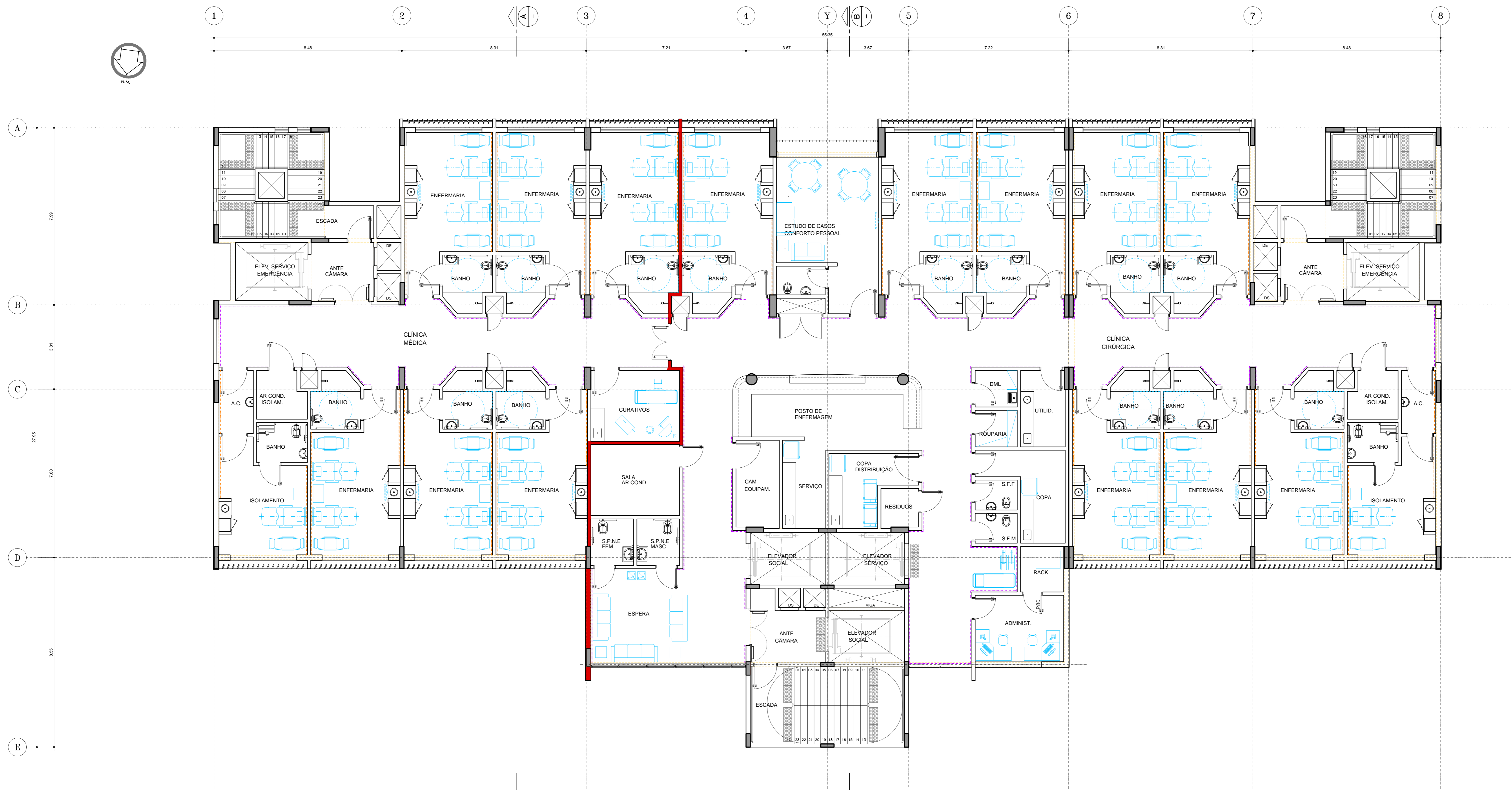
PLANTA DE LAYOUT - 4º PAVIMENTO ESC. 1:75
