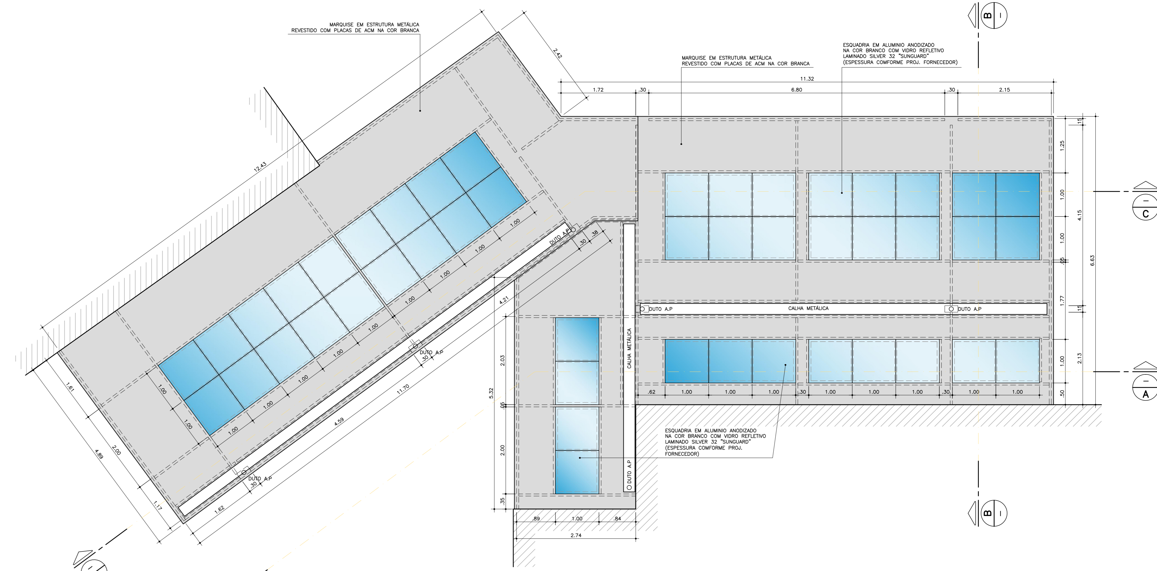
PLANTA COBERTURA - INTERLIGAÇÃO ESC. 1:50
