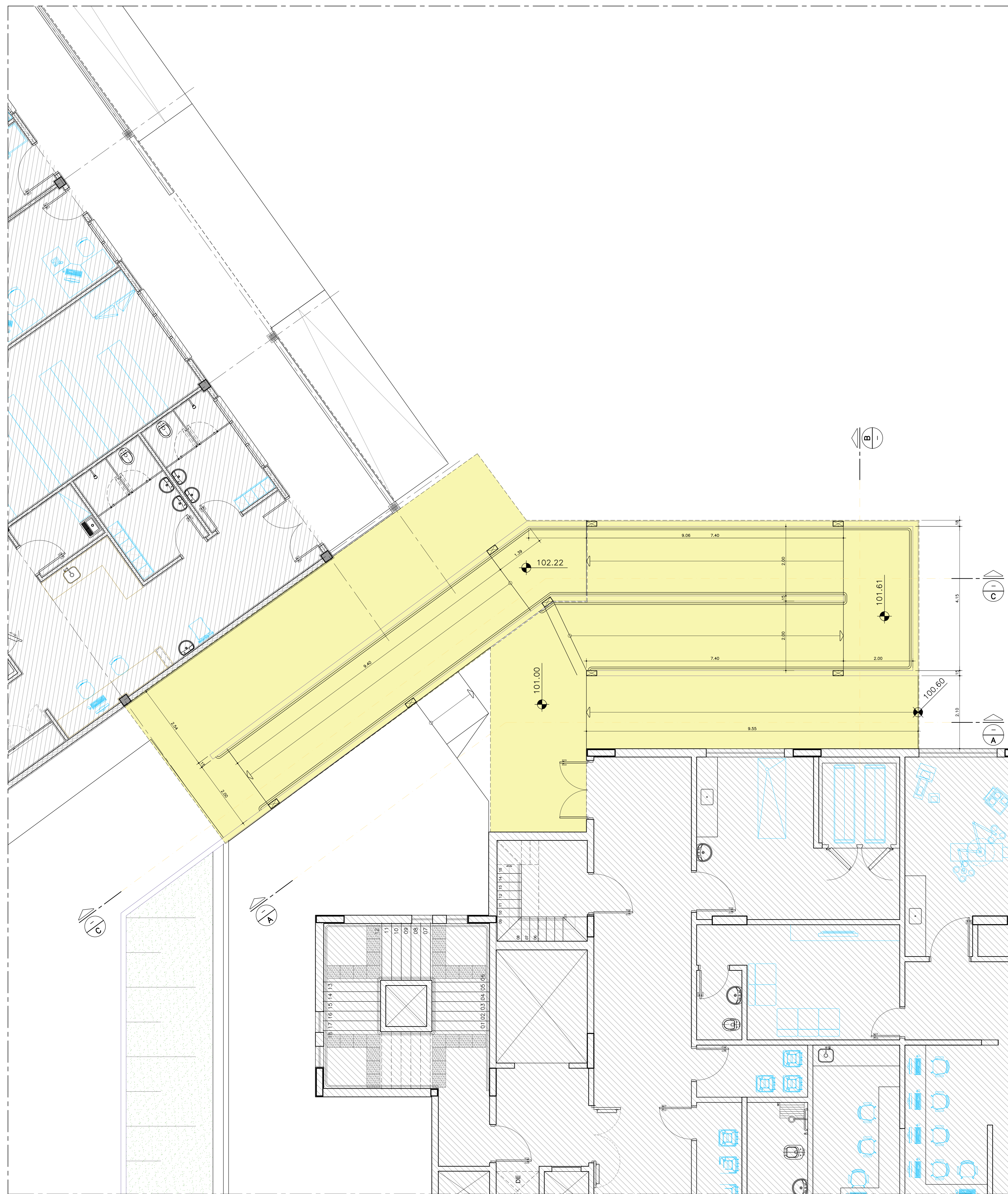
PLANTA BAIXA - INTERLIGAÇÃO ESC. 1:50
