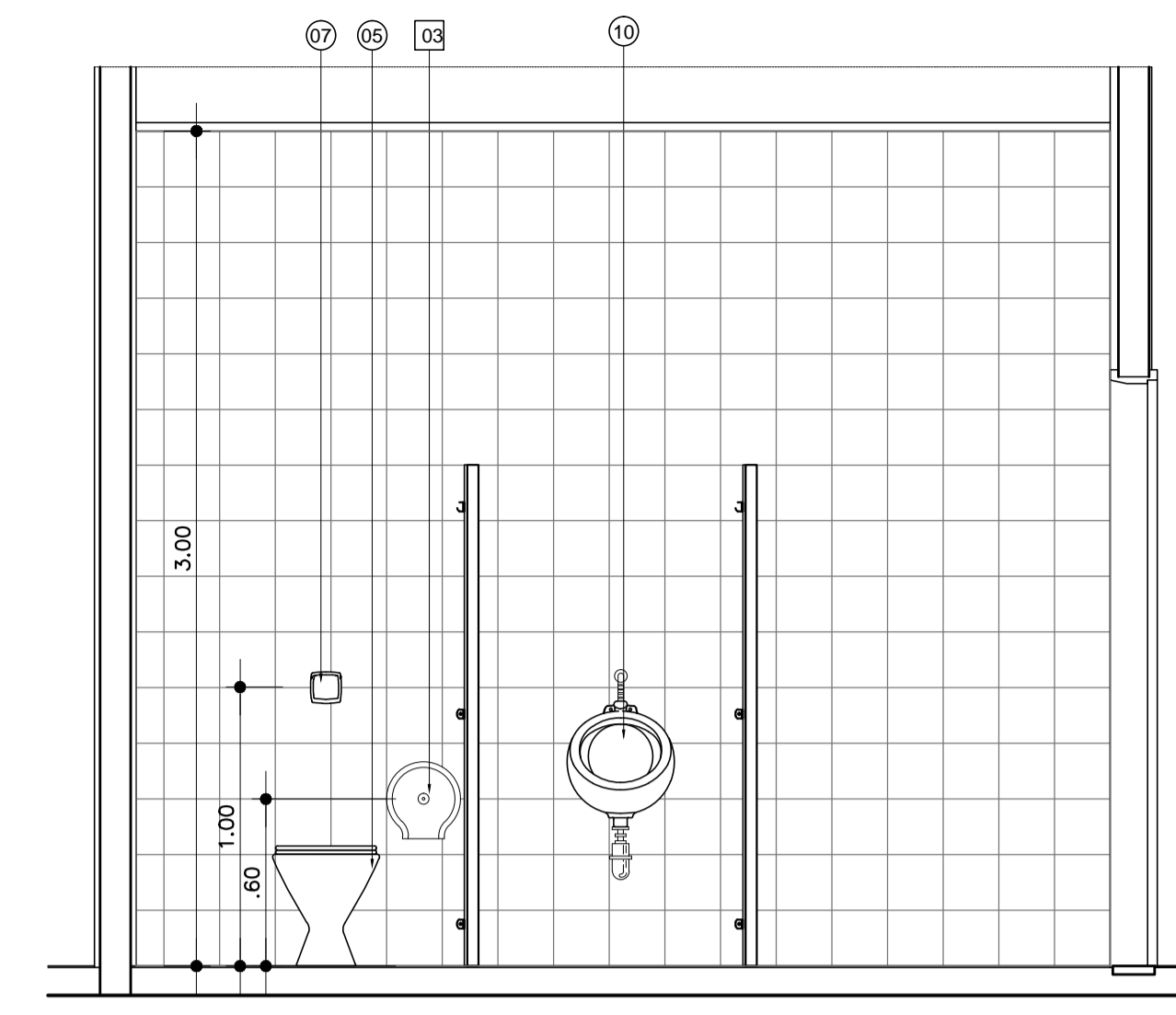
VISTA 13 ESC.: 1:25
