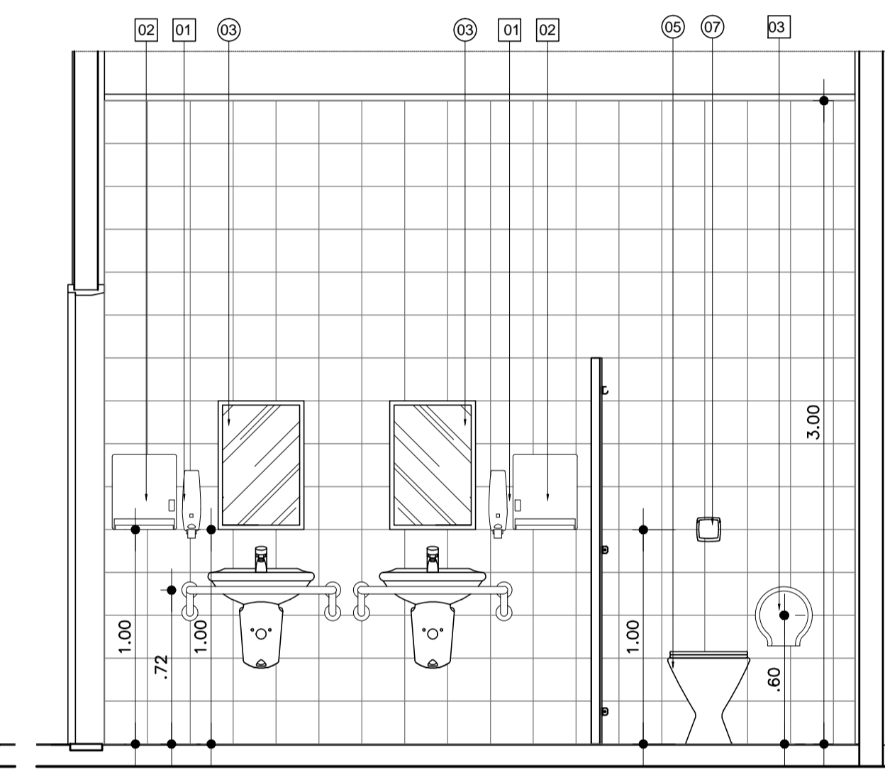
VISTA 15 ESC.: 1:25
