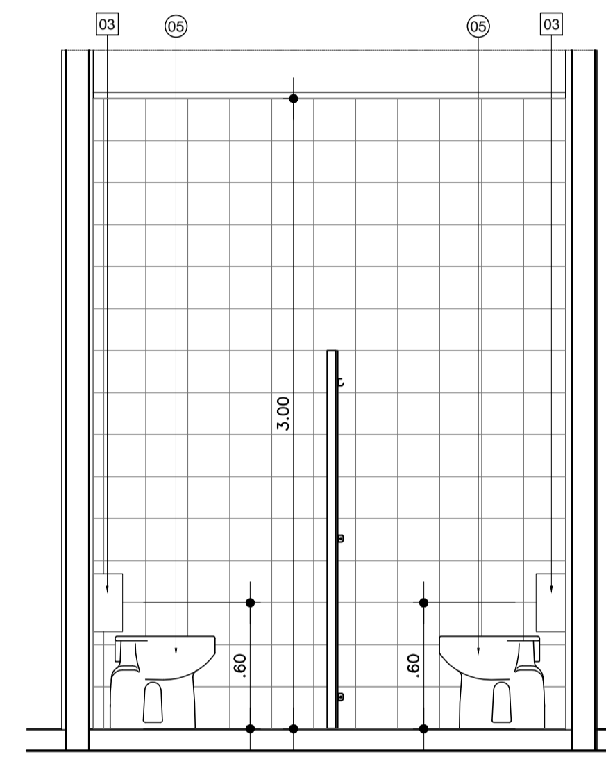
VISTA 16 ESC.: 1:25
