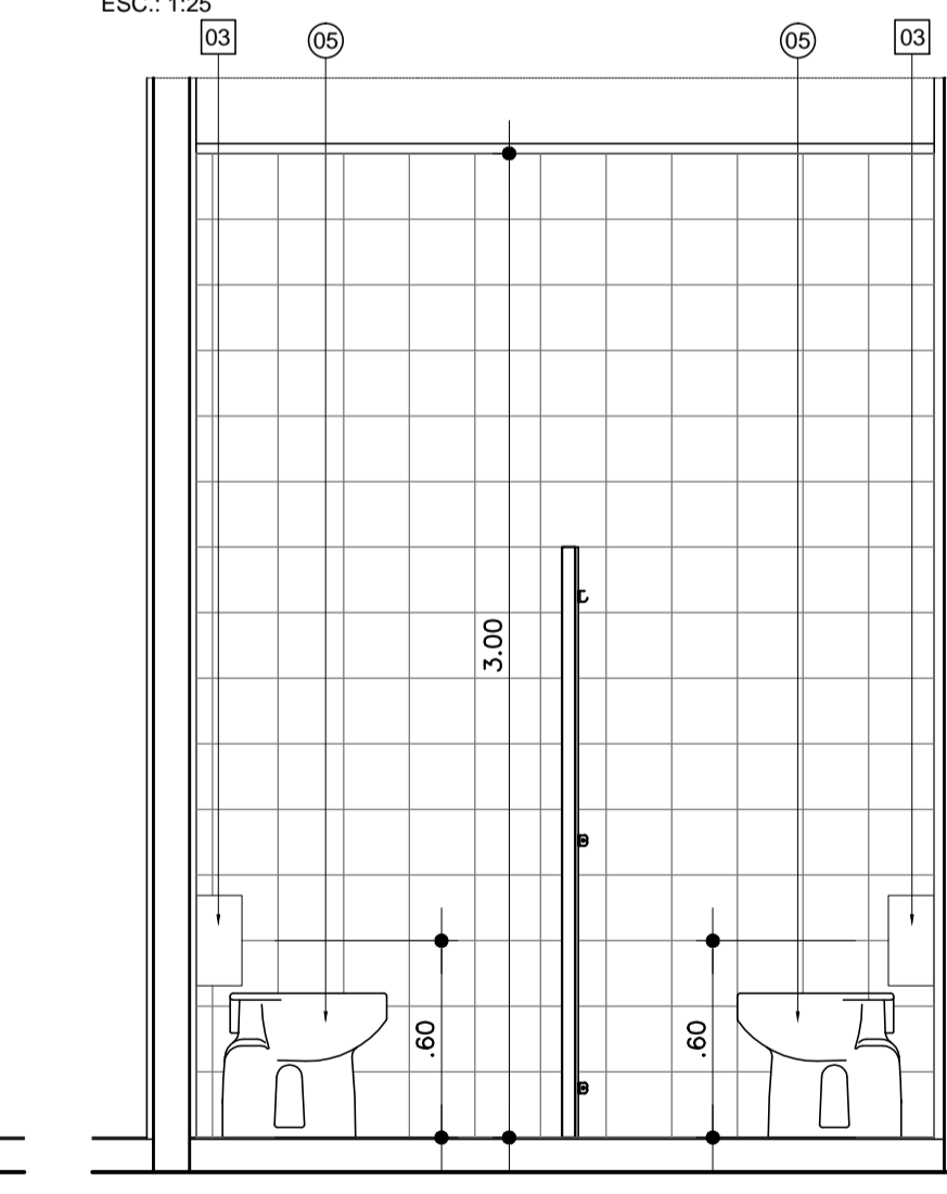
VISTA 20 ESC.: 1:25
