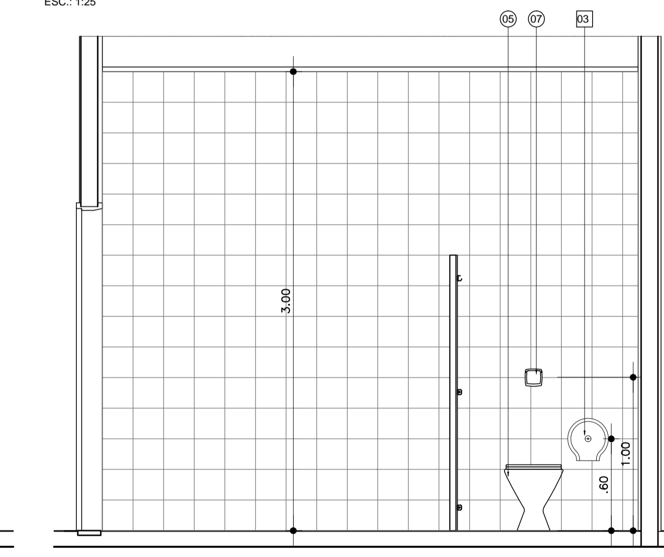
VISTA 19 ESC.: 1:25
