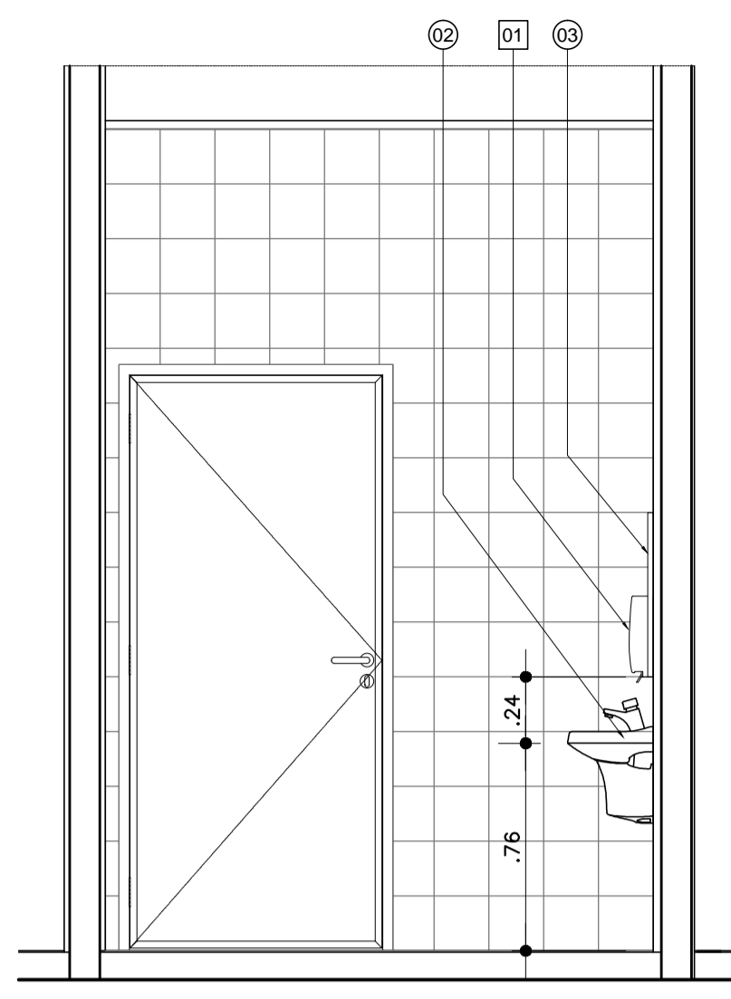
VISTA 10 ESC.: 1:25
