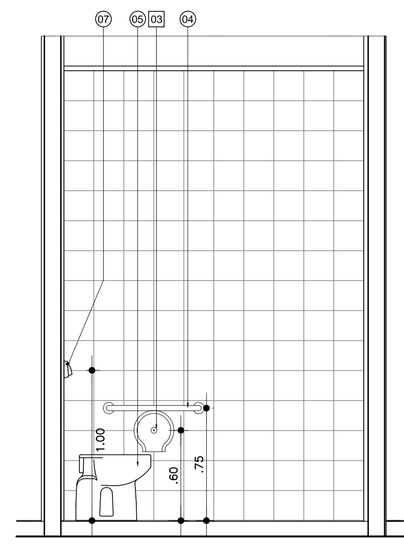
VISTA 12 ESC.: 1:25
