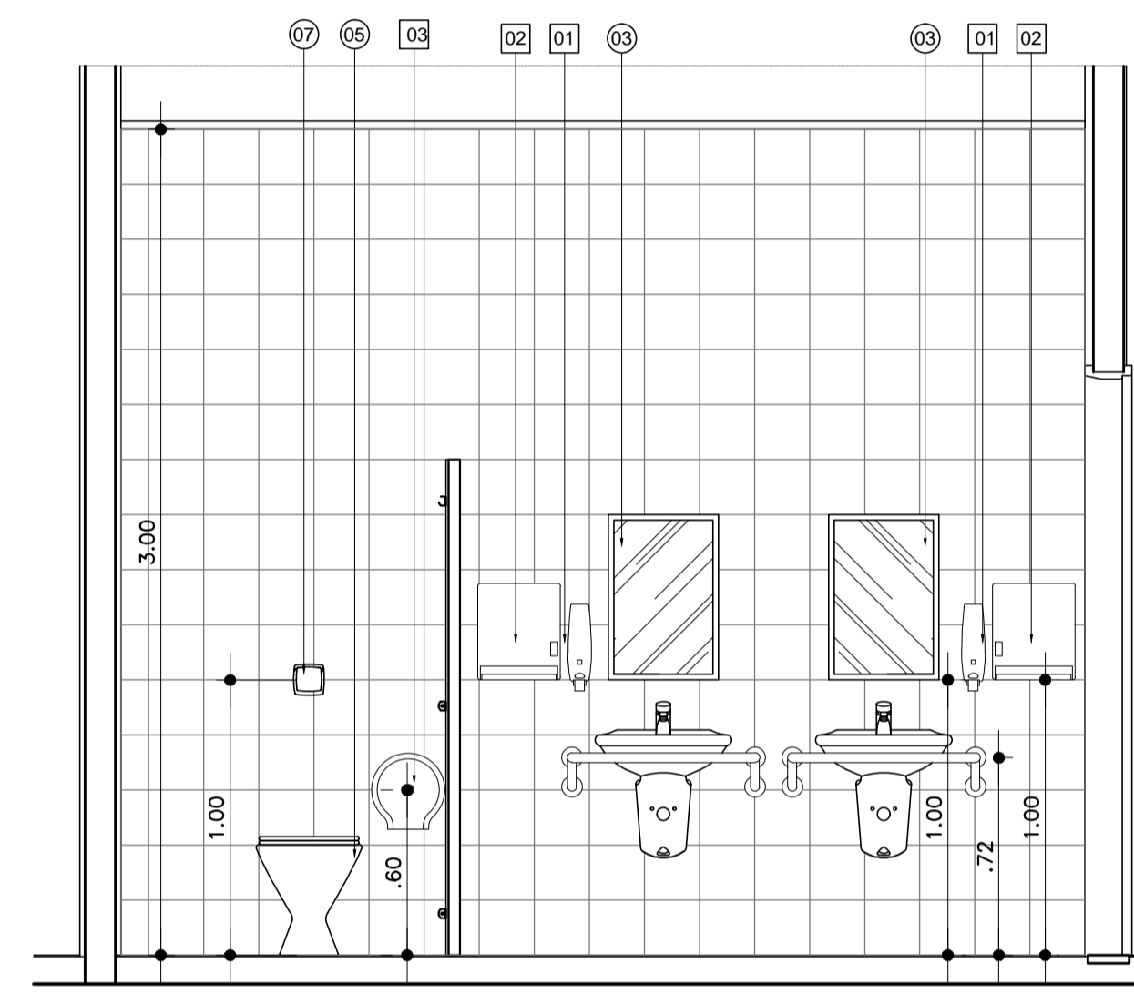
VISTA 17 ESC.: 1:25
