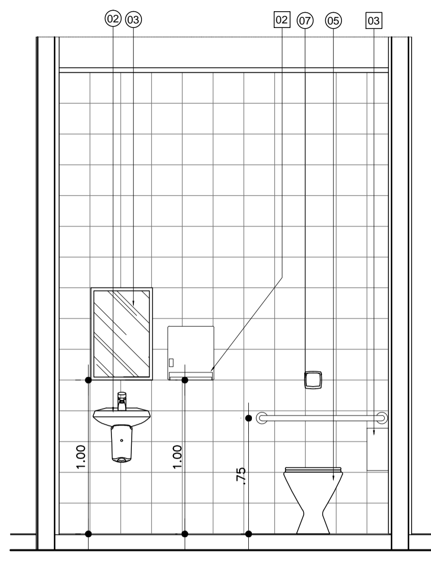
VISTA 11 ESC.: 1:25
