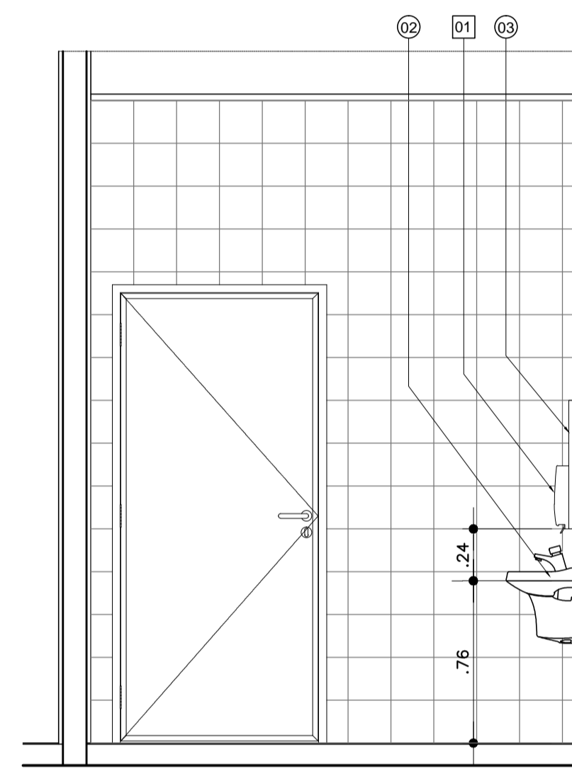
VISTA 14 ESC.: 1:25
