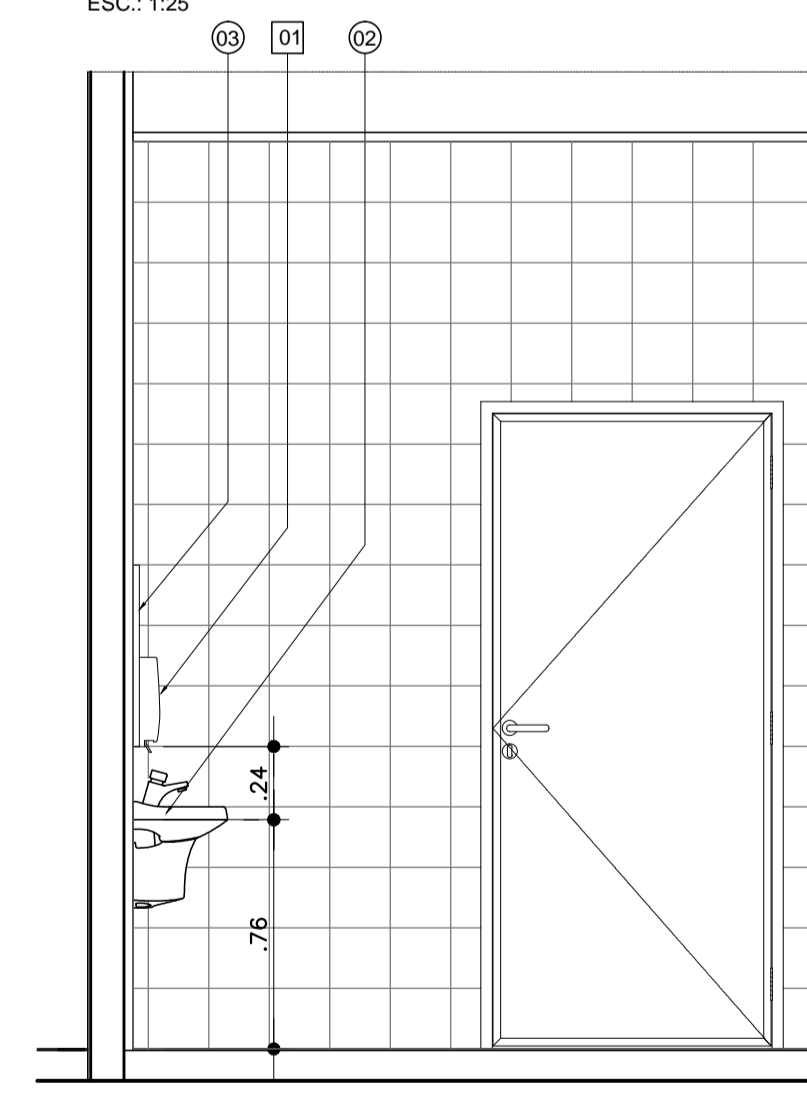
VISTA 18 ESC.: 1:25 AM 04 - AMPLIAÇÃO WC - PAVIMENTO TÉRREO
