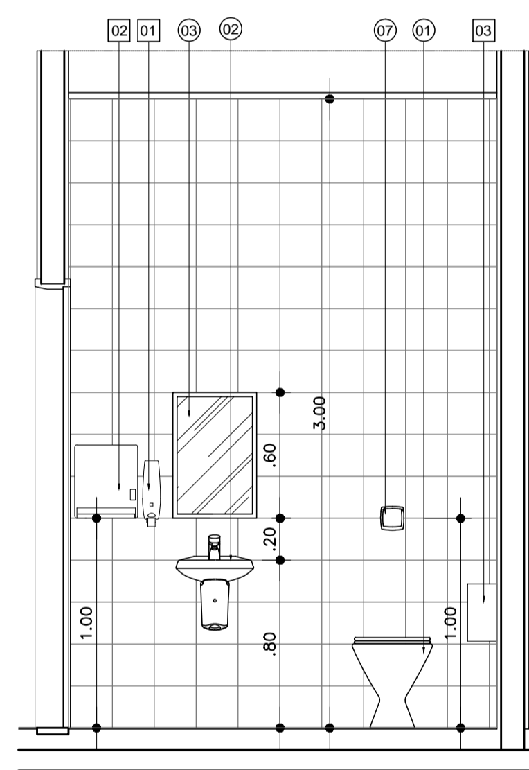
VISTA 03 ESC.: 1:25
