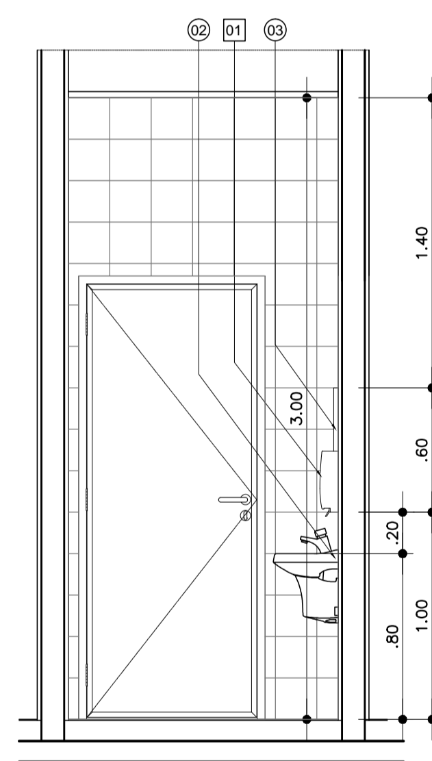
VISTA 02 ESC.: 1:25
