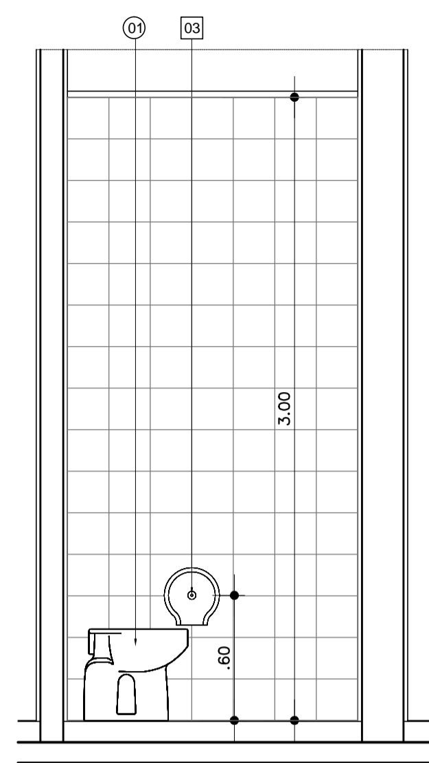
VISTA 02 ESC.: 1:25
