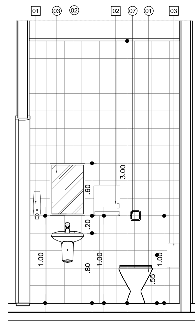
VISTA 01 ESC.: 1:25
