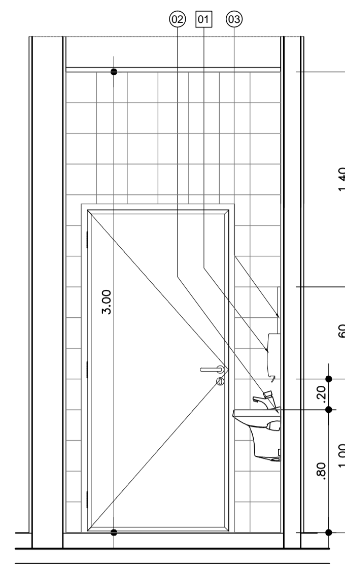
VISTA 04 ESC.: 1:25
