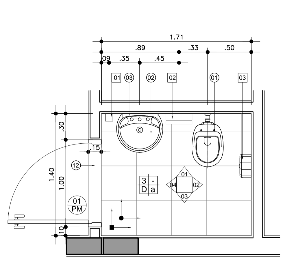
PLANTA ESC.: 1:25 AM 08 - AMPLIAÇÃO SANITÁRIO - PAVIMENTO TÉRREO
