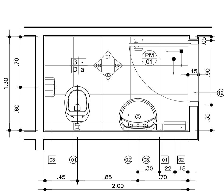
PLANTA ESC.: 1:25 AM 10 - AMPLIAÇÃO SANITÁRIO - PAVIMENTO TÉRREO
