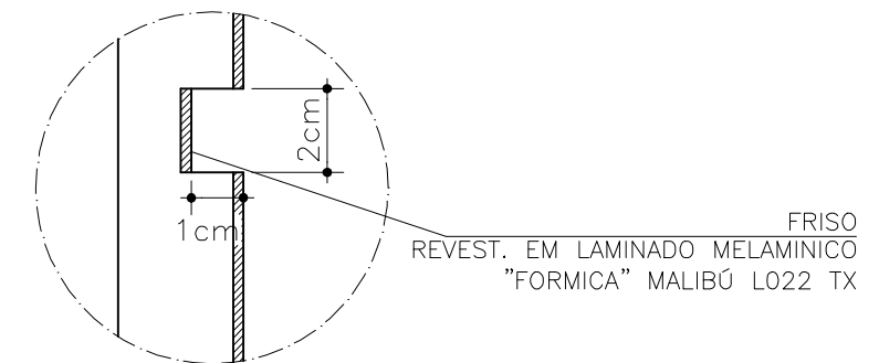
DET. FRISO ESC. 1:2,5
