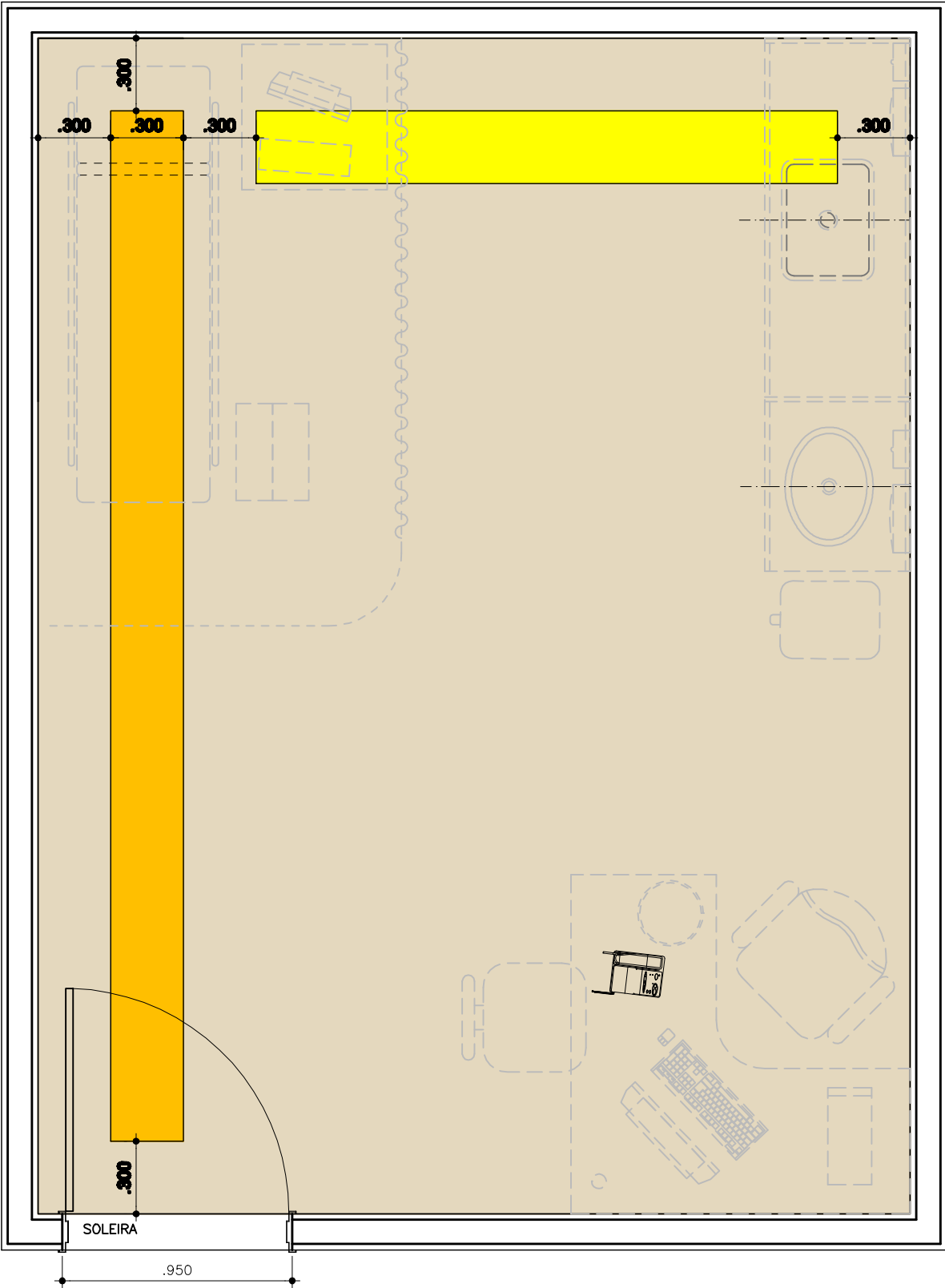
PLANTA DE PAGINAÇÃO DE PISO ESCALA 1/25
