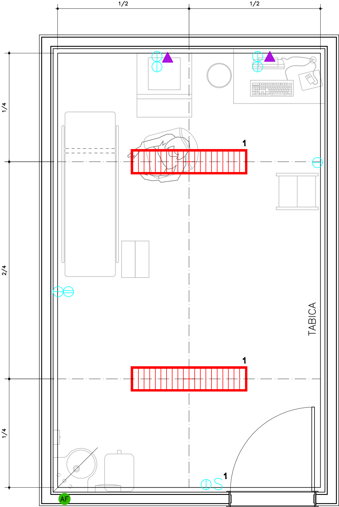
PLANTA PONTOS DE INSTALAÇÕES ESCALA 1/25
