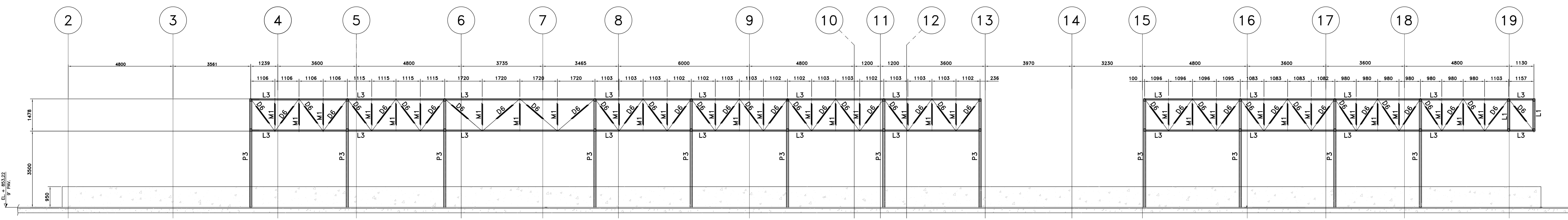
CORTE F - F ESC. 1:50
