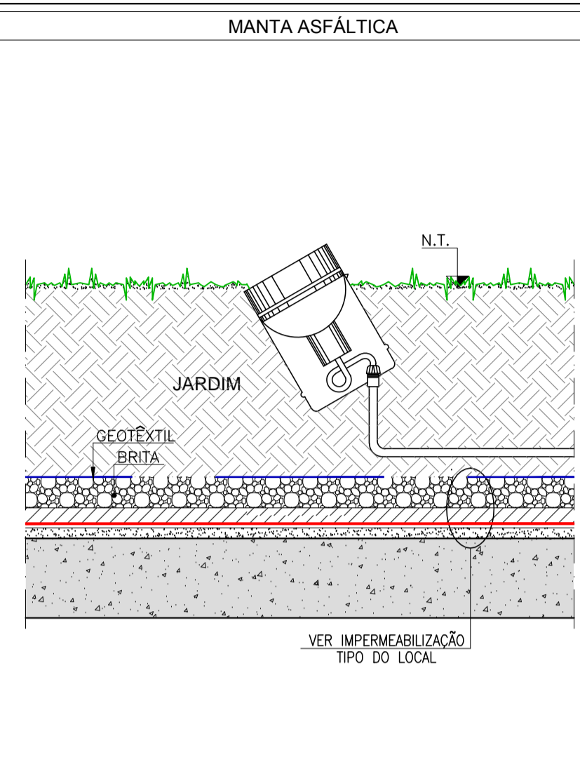
DETALHE " 24 " PROJETO JARDIM SEM ESCALA
