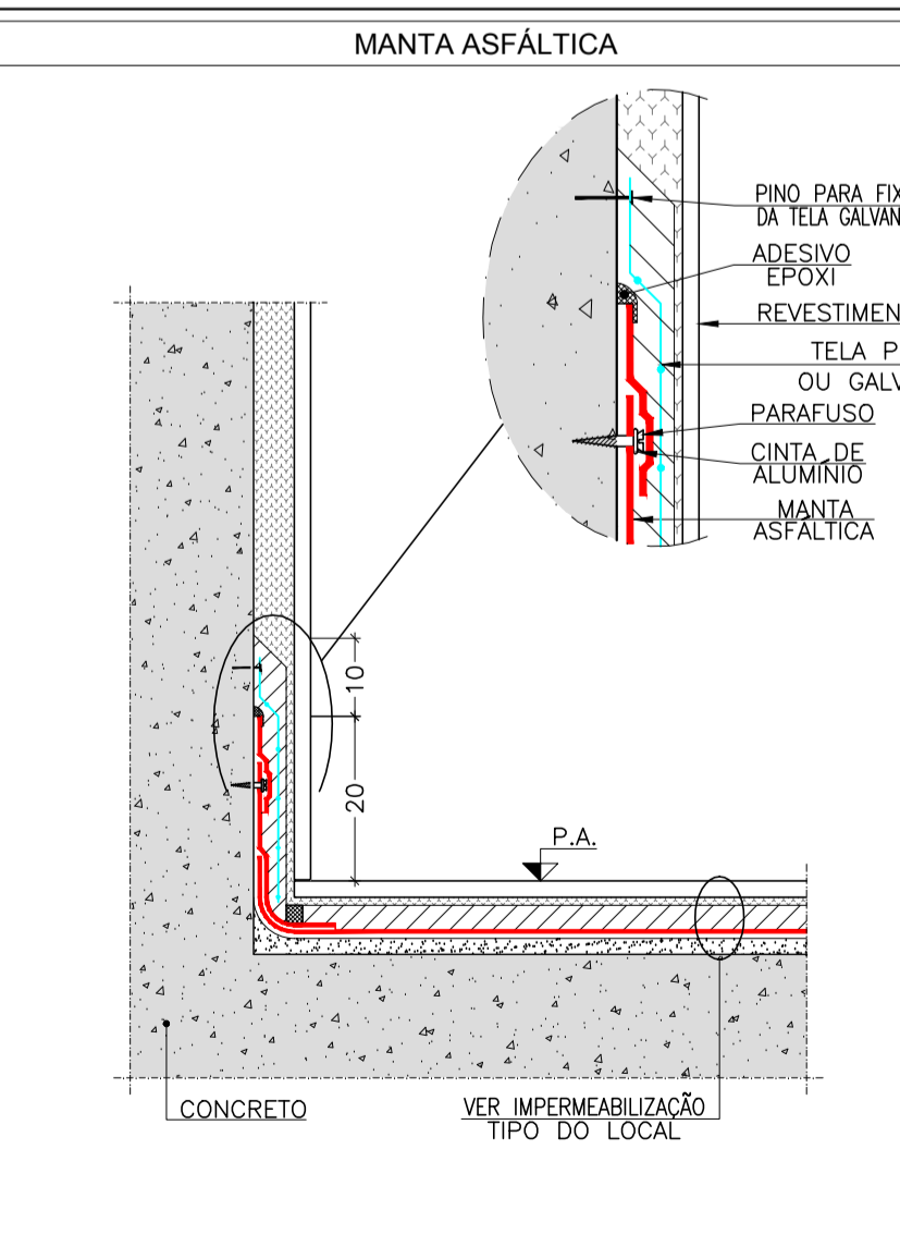
DETALHE " 32 " RODAPÉ EM CONCRETO COM CINTAMENTO SEM ESCALA
