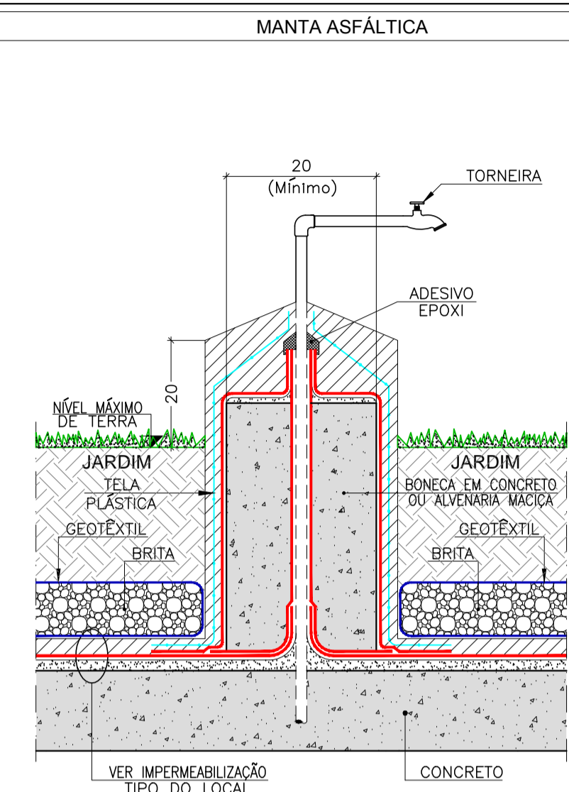
DETALHE " 25 " TORNEIRA JARDIM (CONCRETO) SEM ESCALA
