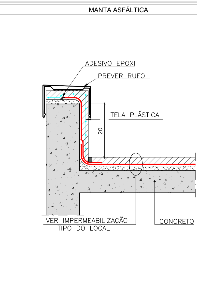
DETALHE " 33 " PLATIBANDA LAJE DE COBERTURA SEM ESCALA
