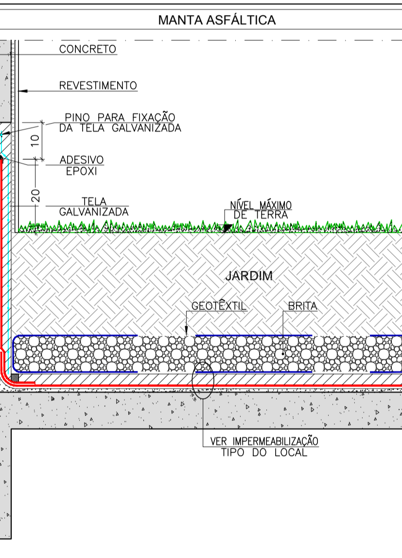
DETALHE " 28 " RODAPÉ COM ENCAIXE EM CONCRETO JARDIM SEM ESCALA
