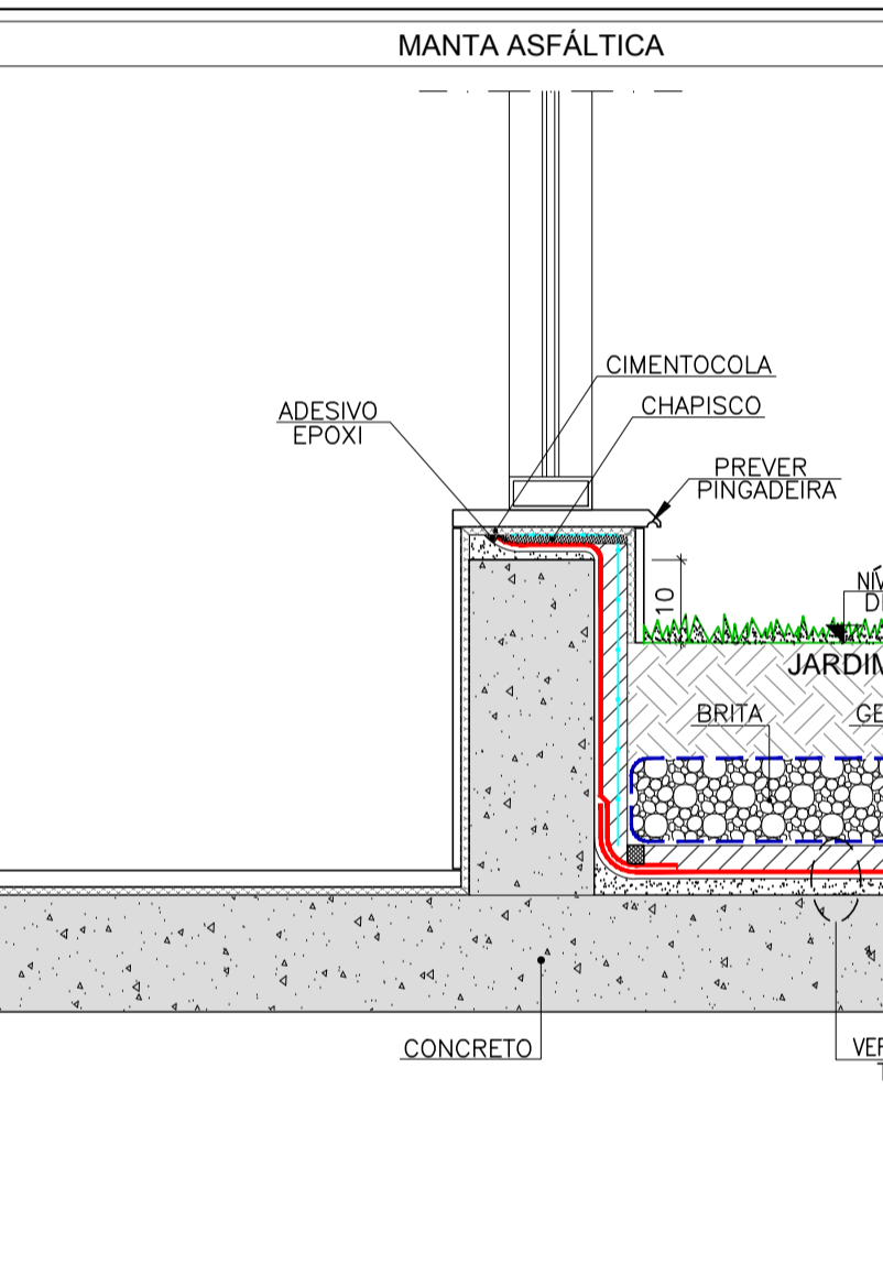
DETALHE " 29 " SOLEIRA JARDIM SEM ESCALA
