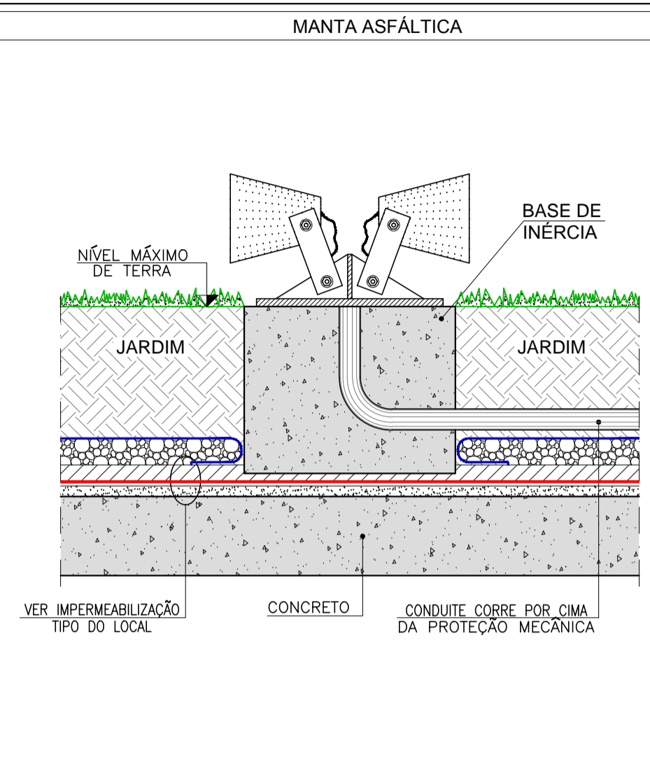
DETALHE " 23 " LUMINÁRIA JARDIM SEM ESCALA
