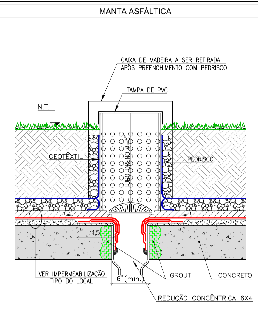
DETALHE " 26 " CAPTAÇÃO EM ÁREAS COM JARDIM / DRENO PVC SEM ESCALA
