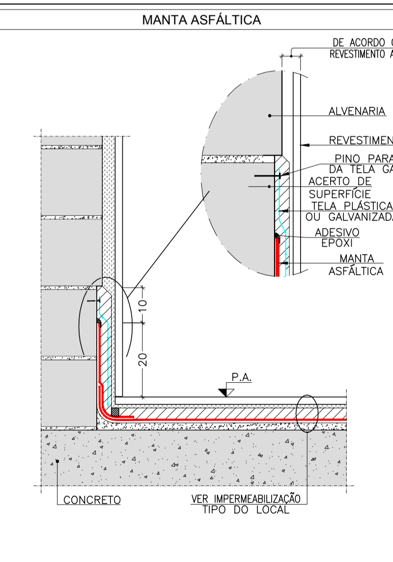
DETALHE " 31 " RODAPÉ EM ALVENARIA COM ENCAIXE SEM ESCALA
