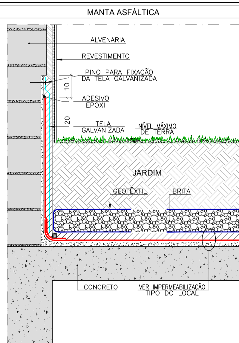
DETALHE " 27 " RODAPÉ ALVENARIA JARDIM SEM ESCALA
