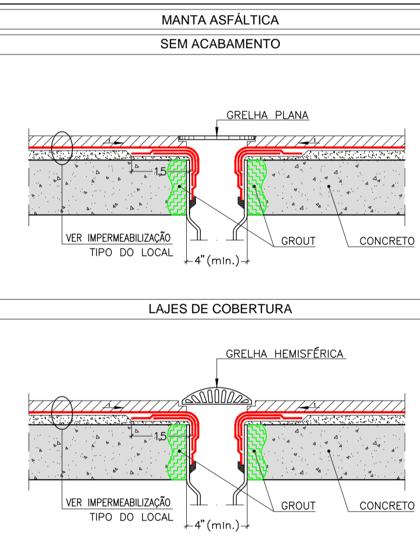
DETALHE " 30 " RALO SEM ESCALA
