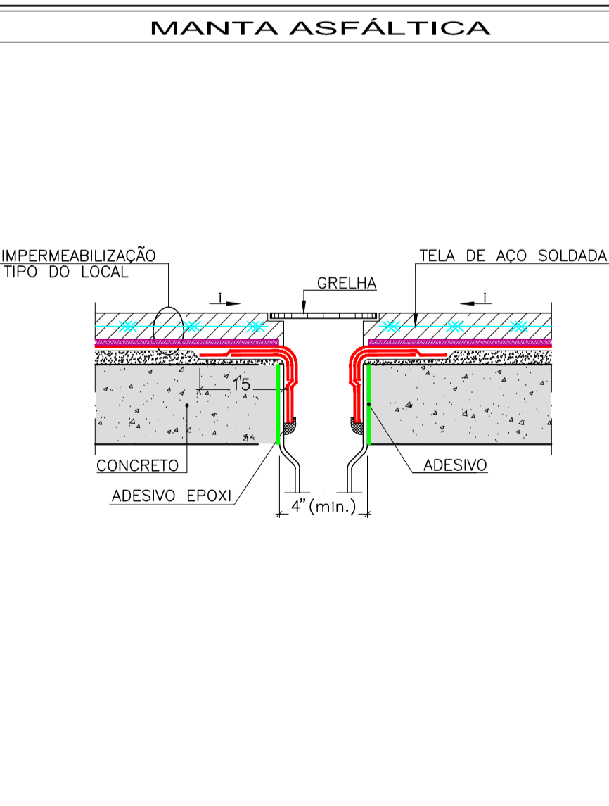
DETALHE " 34 " RALO (CIRCULAÇÃO DE VEÍCULOS) SEM ESCALA
