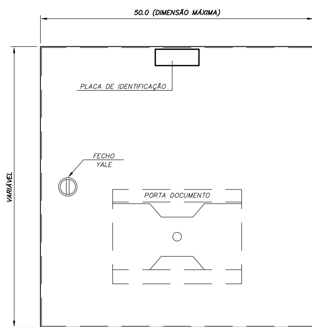
VISTA FRONTAL EXTERNA
