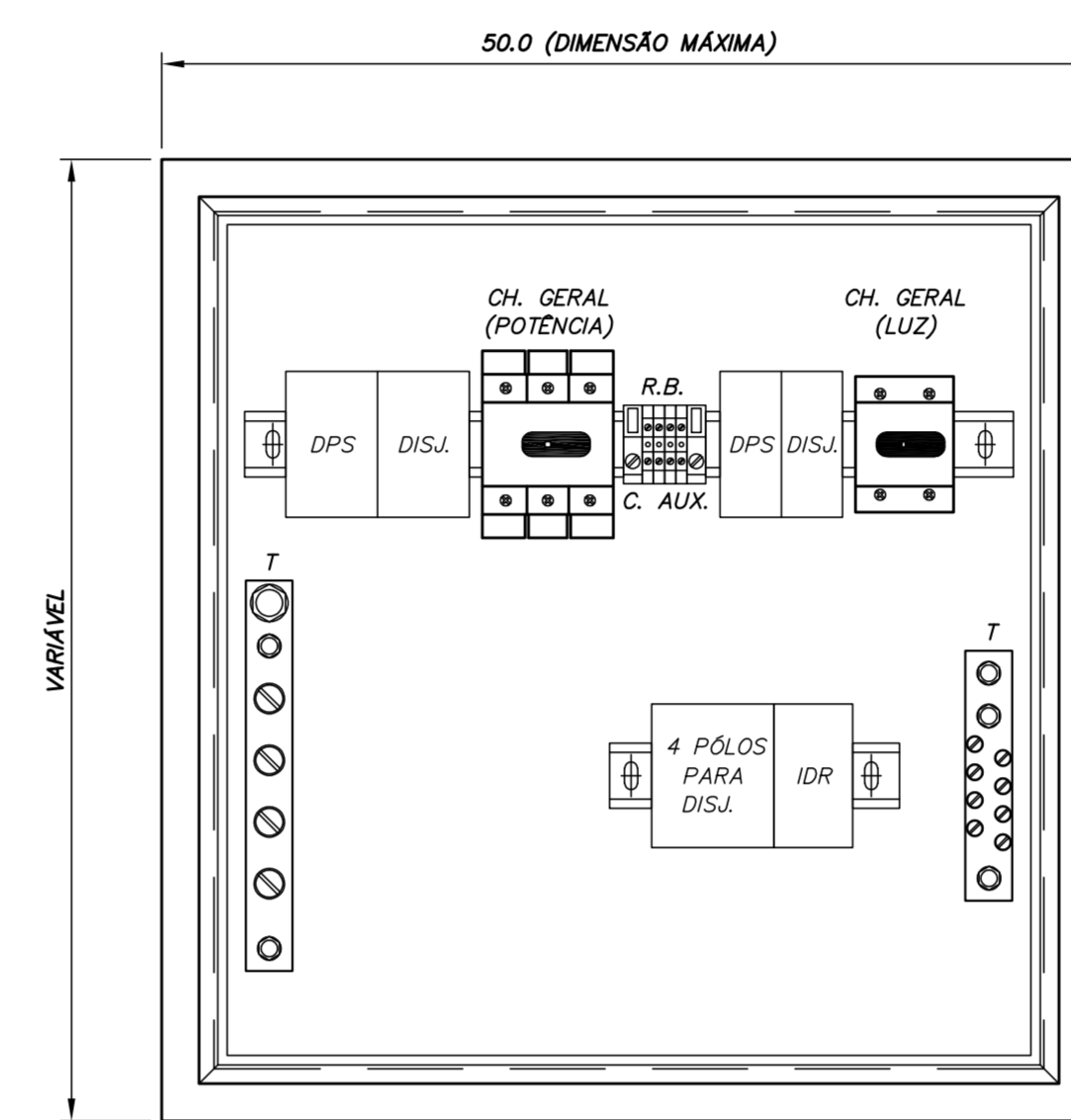
VISTA FRONTAL INTERNA
