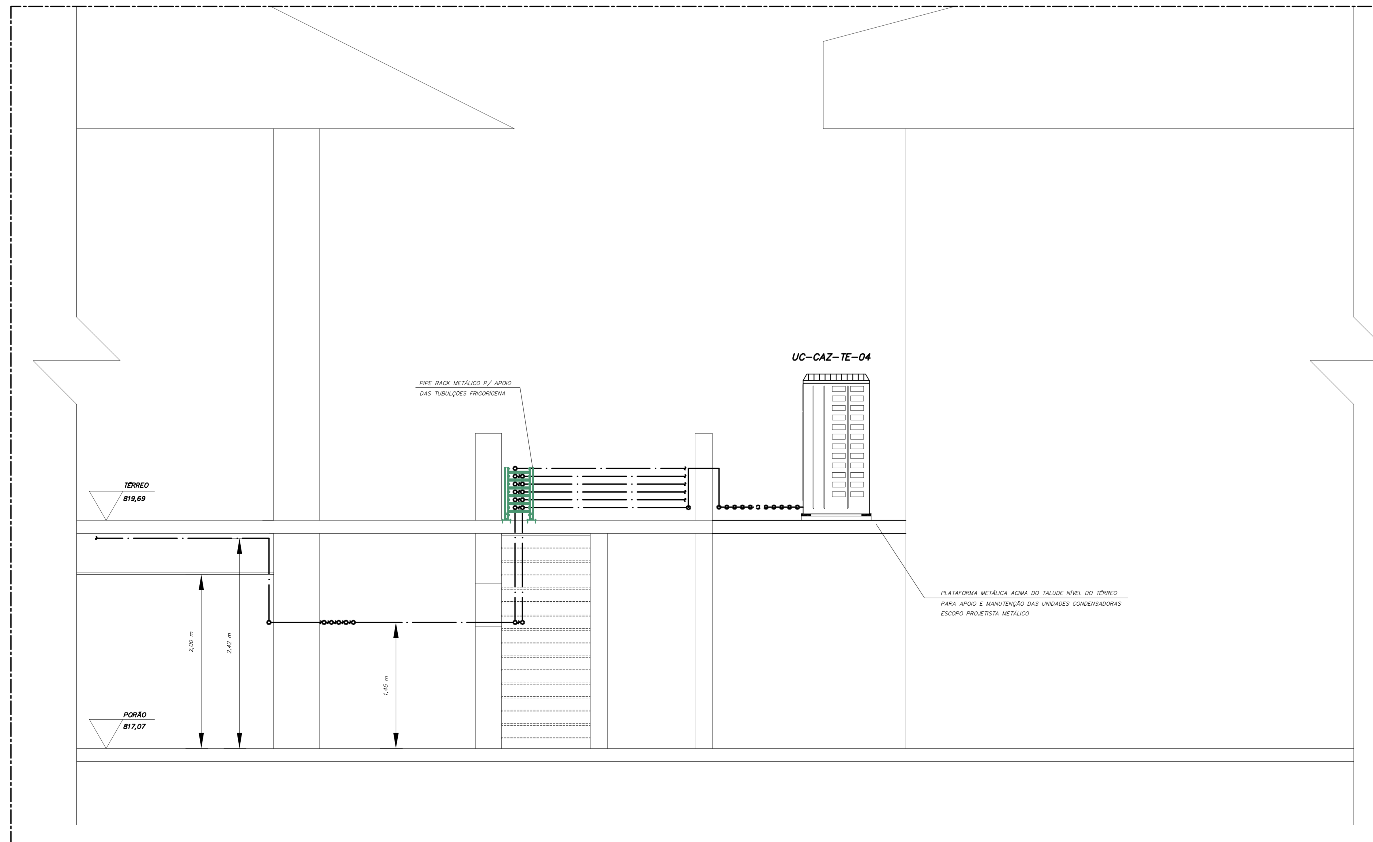
CORTE C-C
