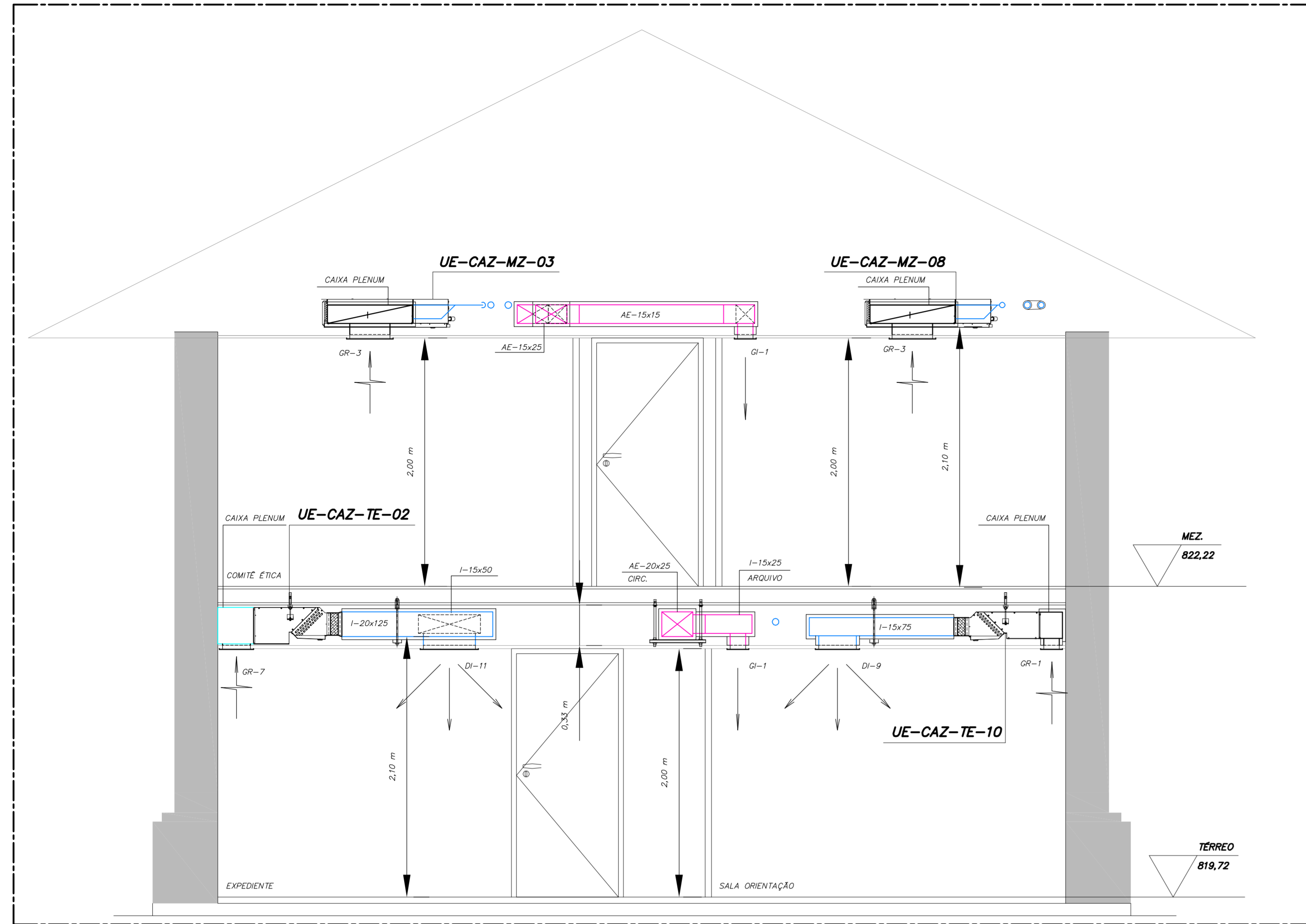
CORTE A-A
