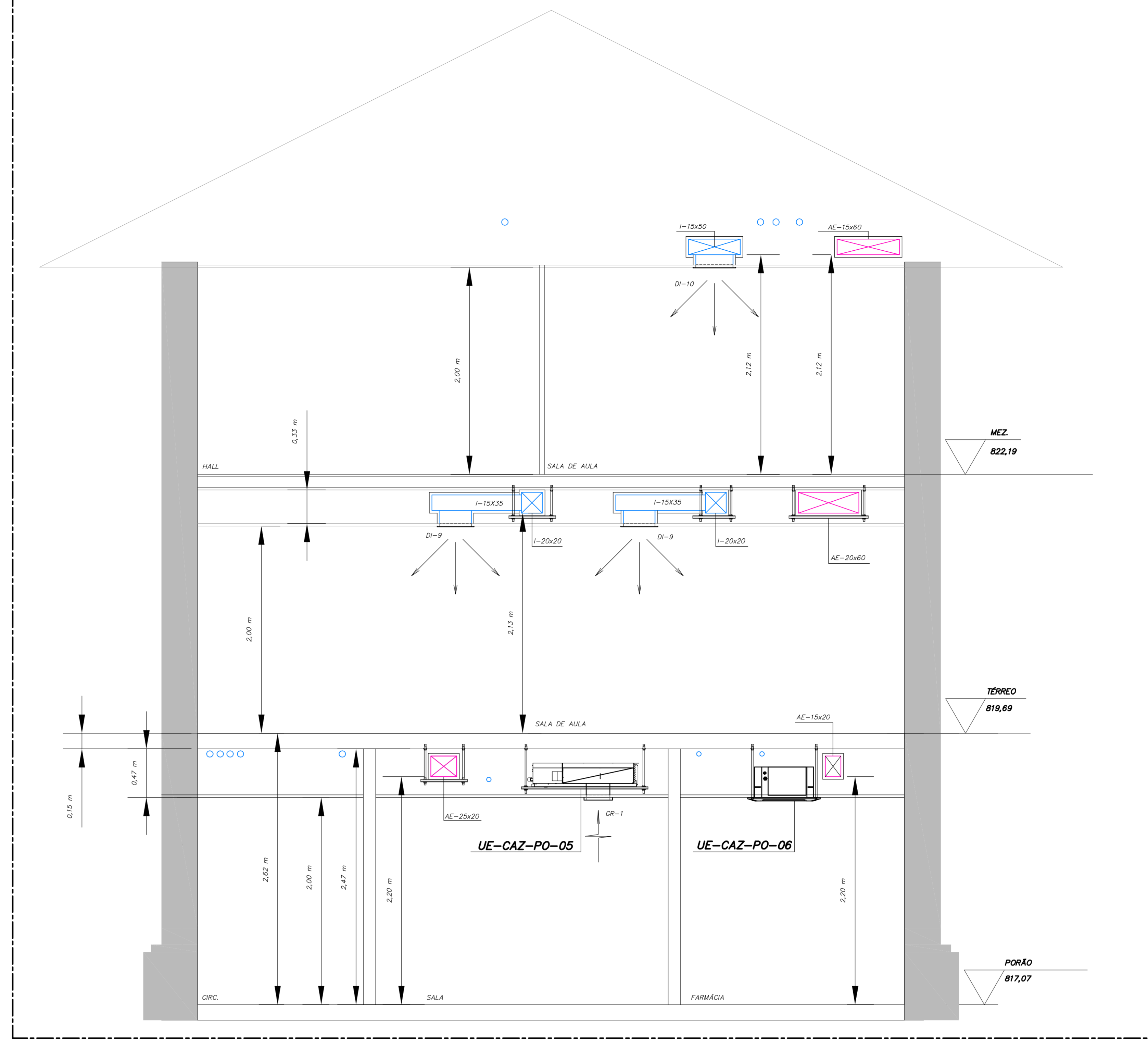
CORTE B-B
