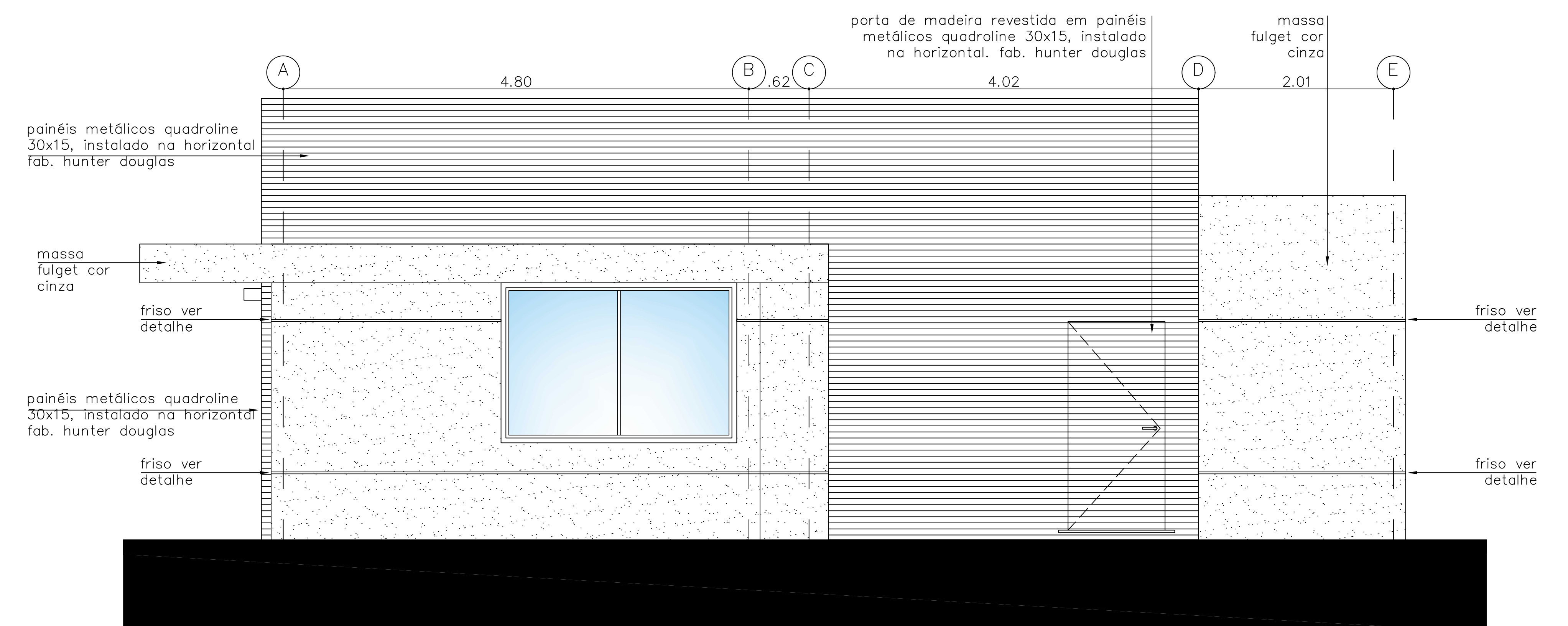
ELEVAÇÃO 04 ESCALA 1:50
