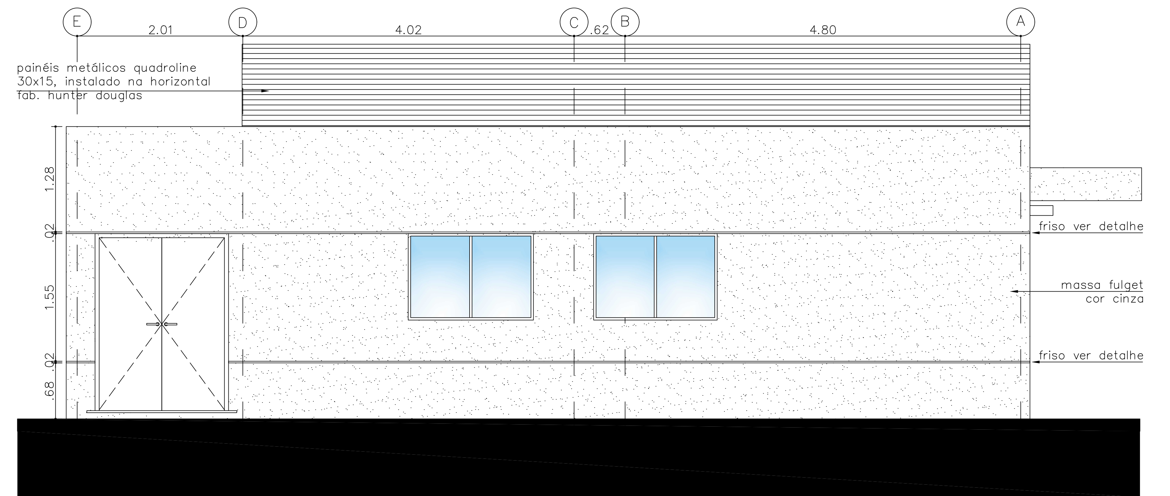
ELEVAÇÃO 02 ESCALA 1:50
