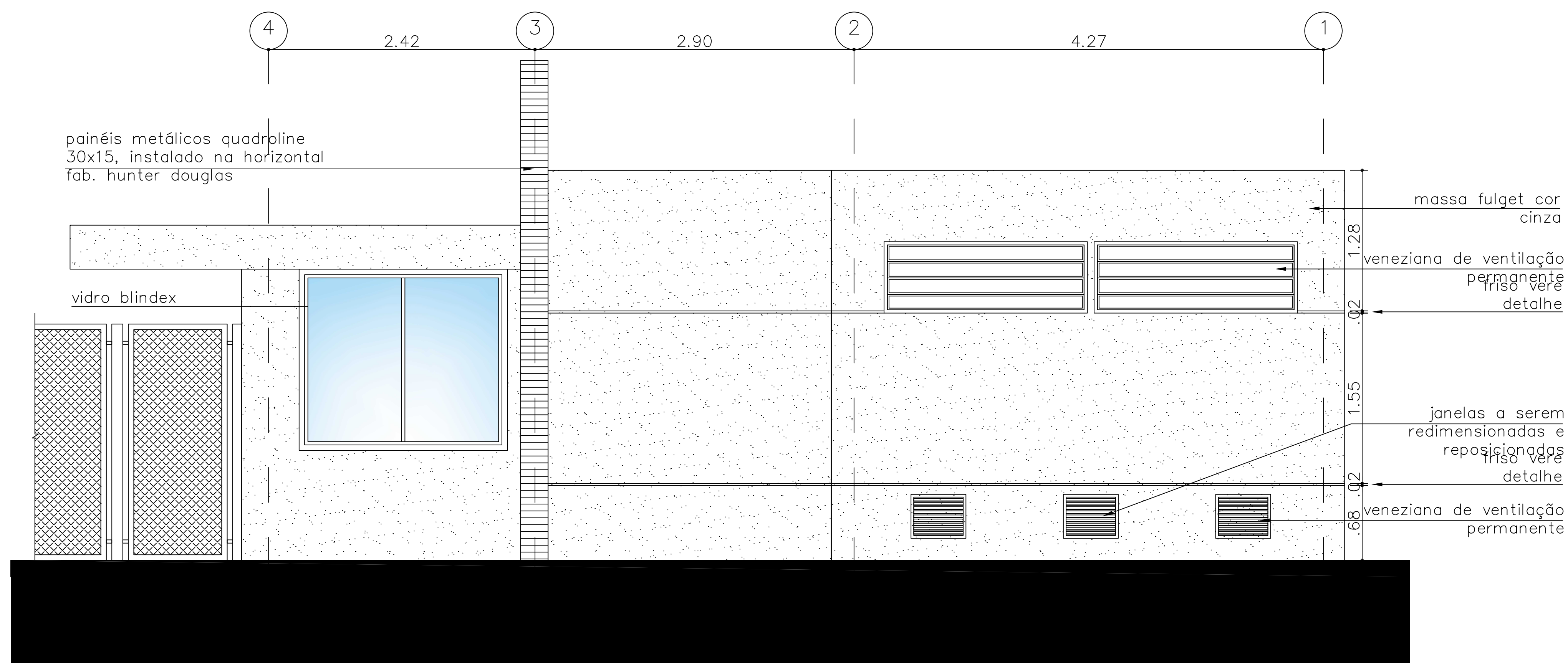
ELEVAÇÃO 01 ESCALA 1:50
