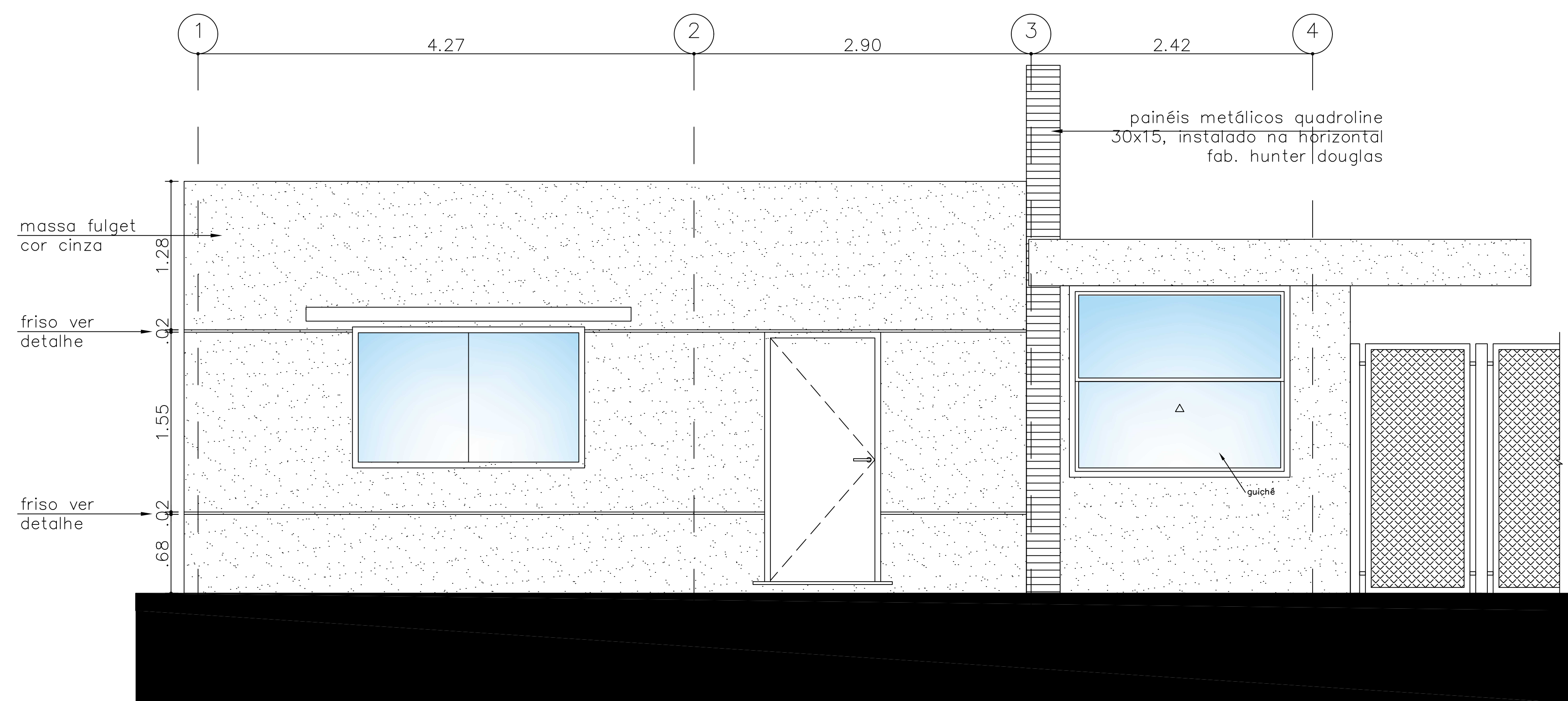
ELEVAÇÃO 03 ESCALA 1:50
