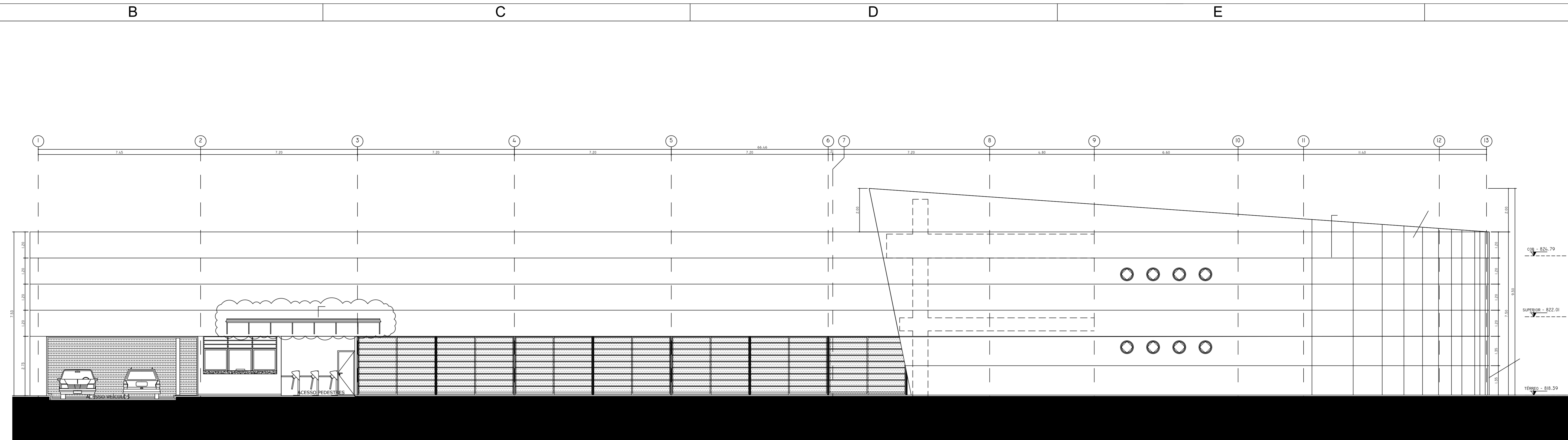
ELEVACÃO 01 ESCALA 1/50
