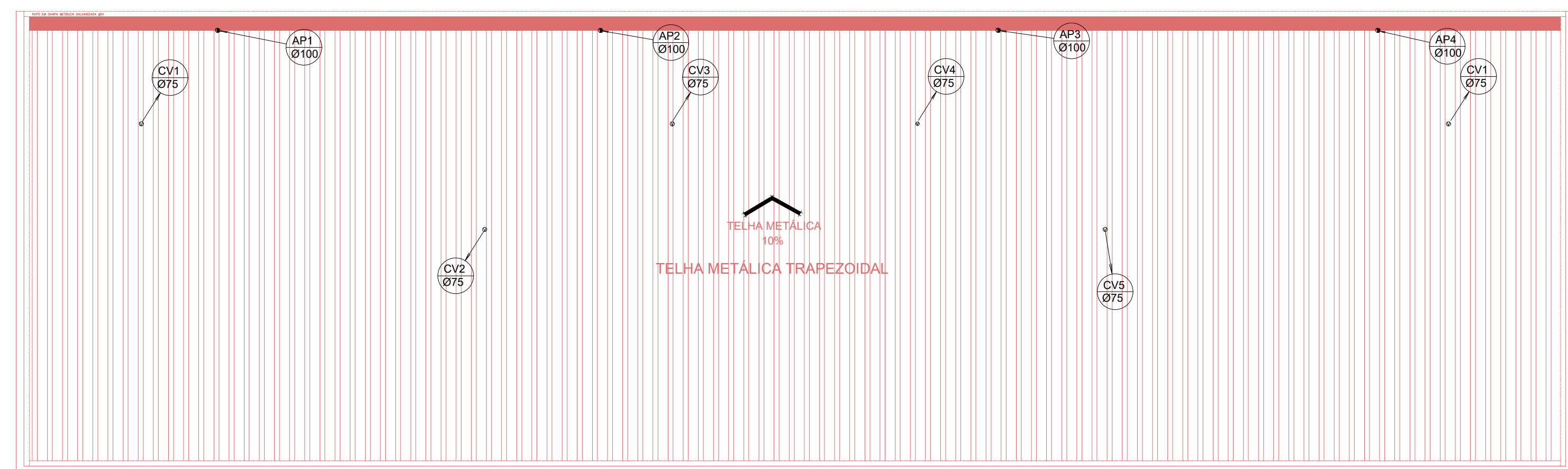
PLANTA DE COBERTURA - VESTIÁRIOS ESCALA 1:75
