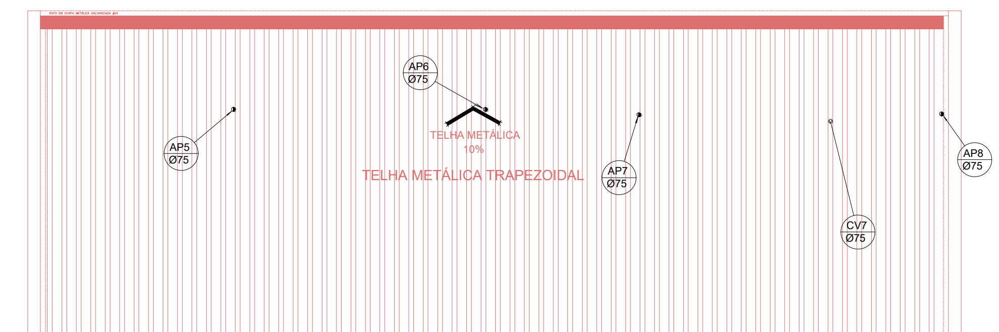
PLANTA DE COBERTURA - PORTARIA ESCALA 1:75
