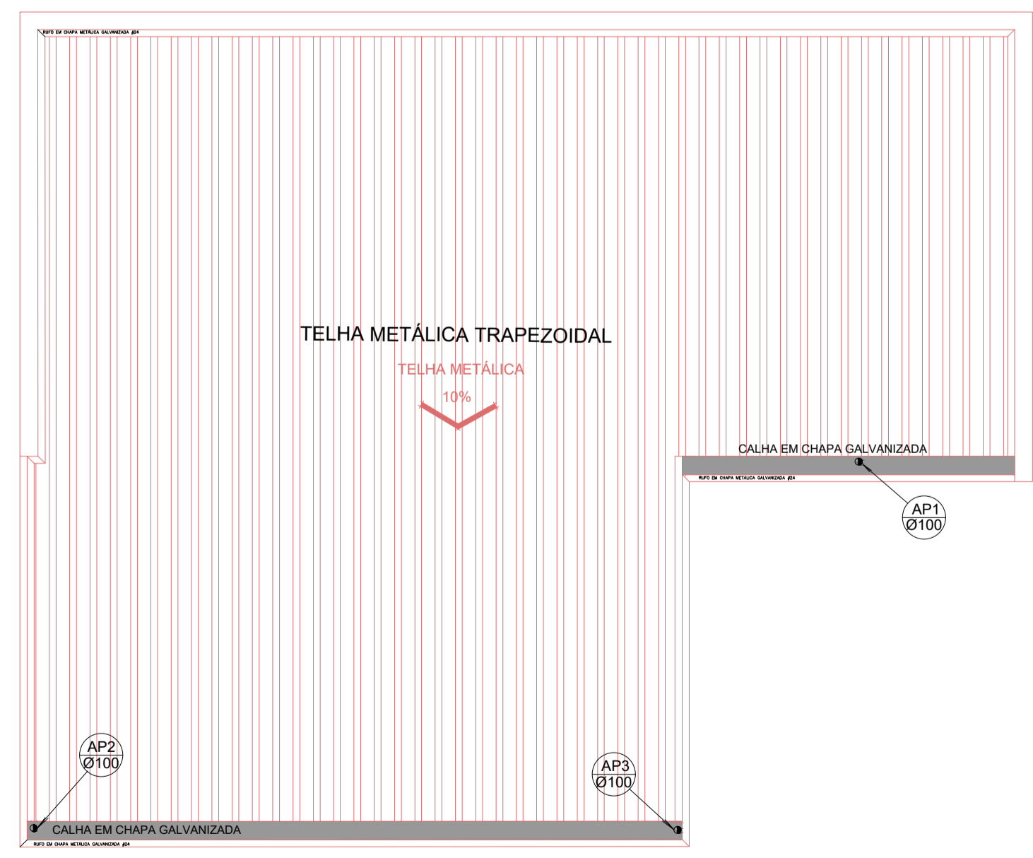
PLANTA DE COBERTURA - MORGUE ESCALA 1:75
