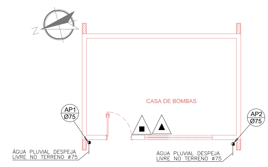
PLANTA BAIXA - CASA DE BOMBAS ESCALA 1:75
