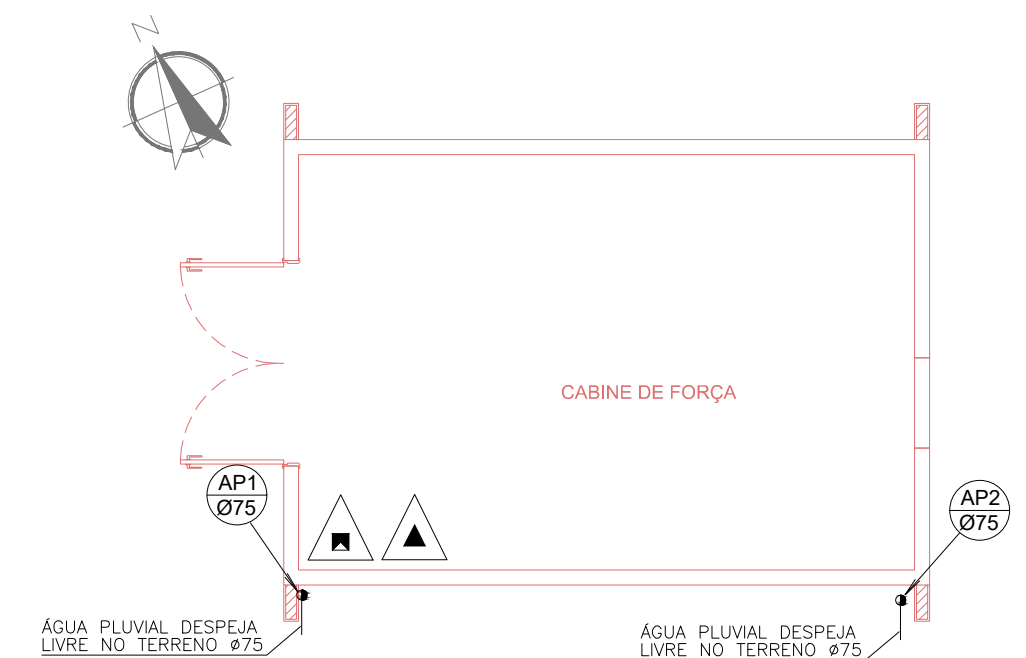
CABINE DE FORÇA PLANTA BAIXA ESCALA 1:75
