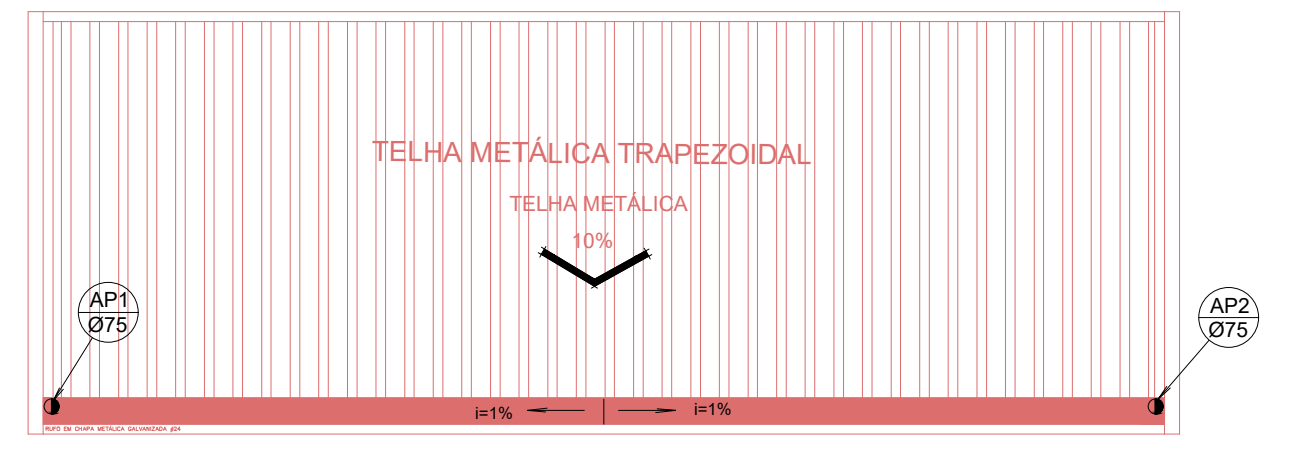
PLANTA COBERTURA
