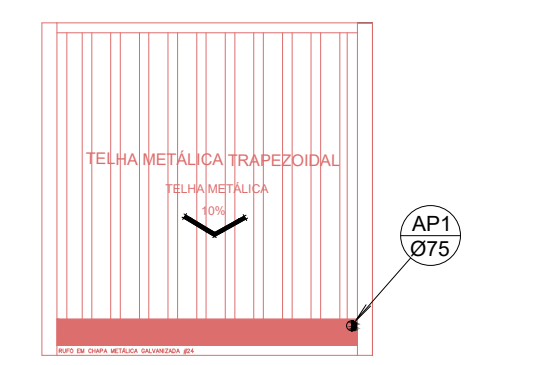
PLANTA COBERTURA ESCALA 1:75
