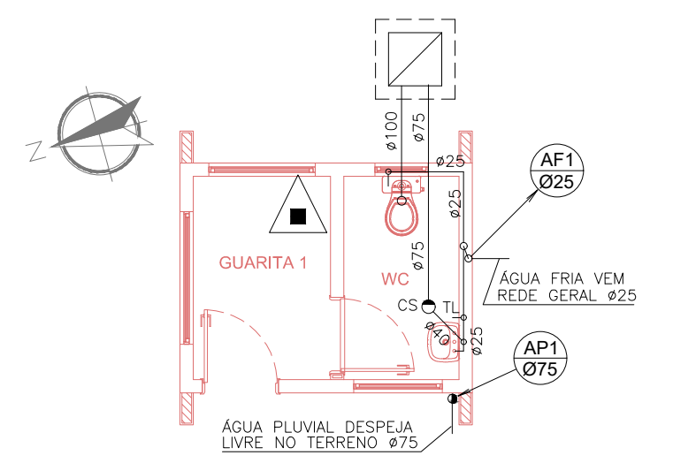
PLANTA BAIXA - GUARITA 1 ESCALA 1:75
