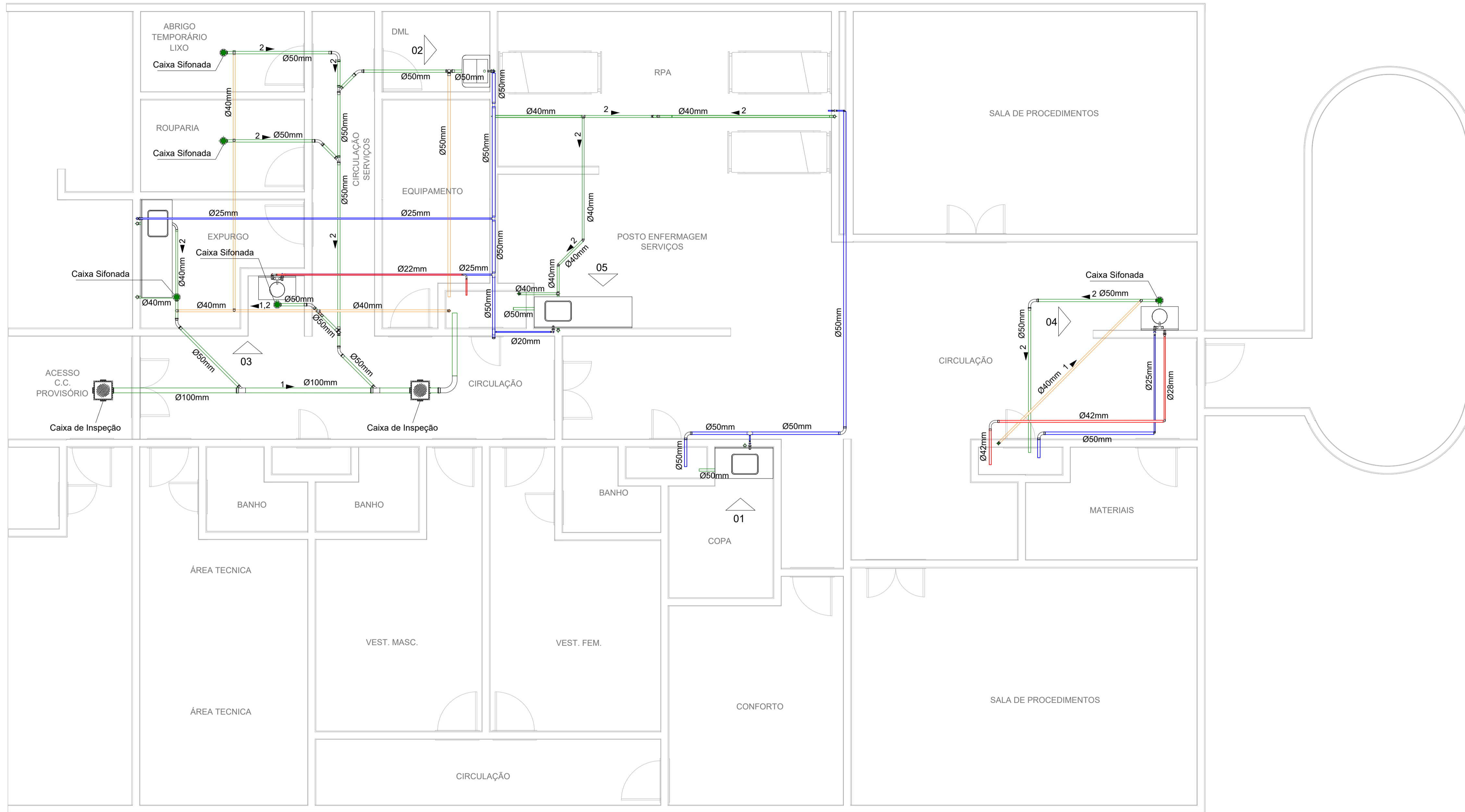
1 Planta Baixa Geral 1 : 50
