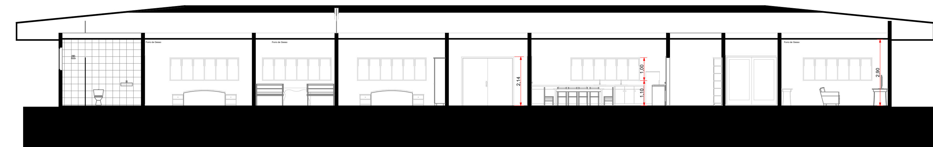
CORTE B-B 1:200
