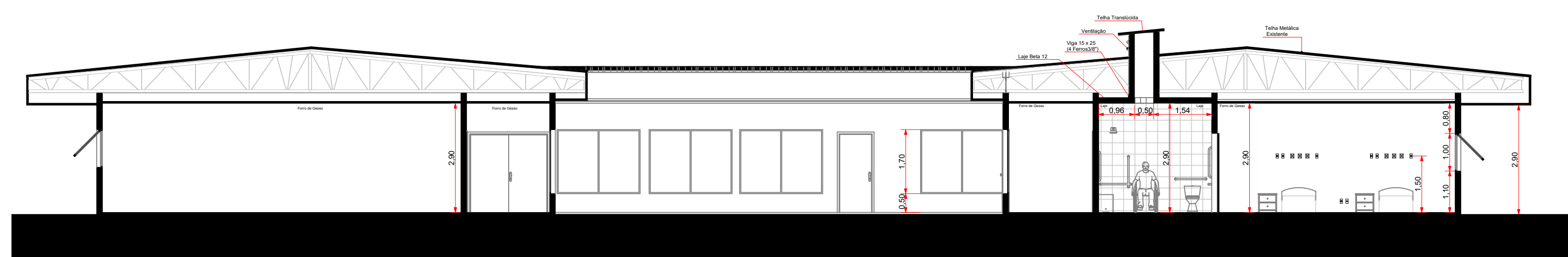
CORTE A-A 1:200
