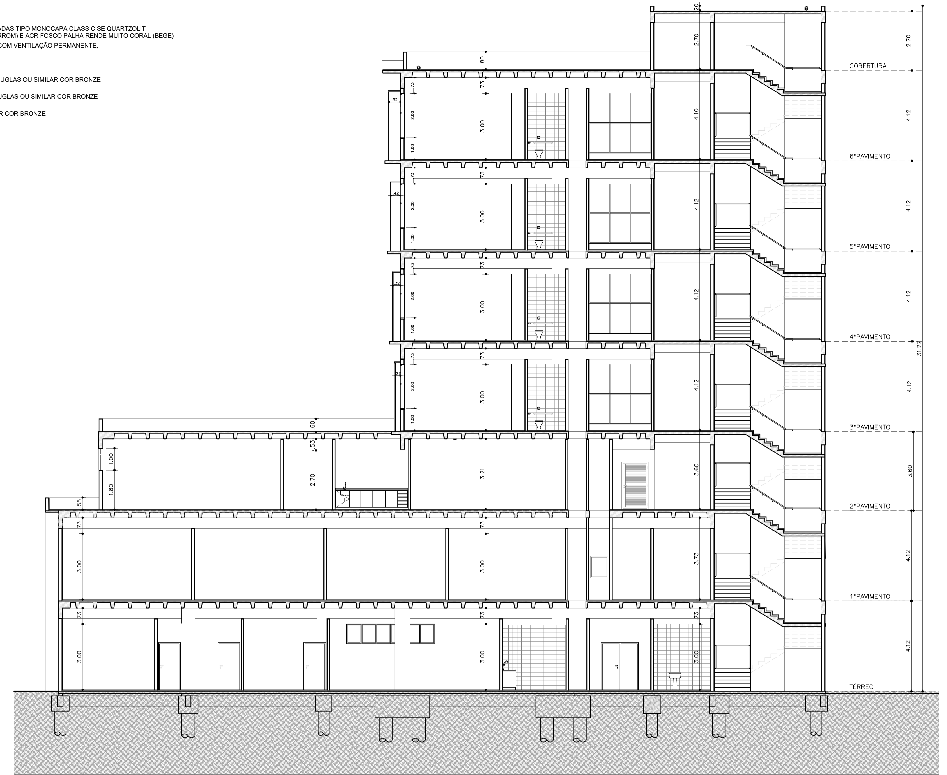
CORTE TRANSVERSAL
