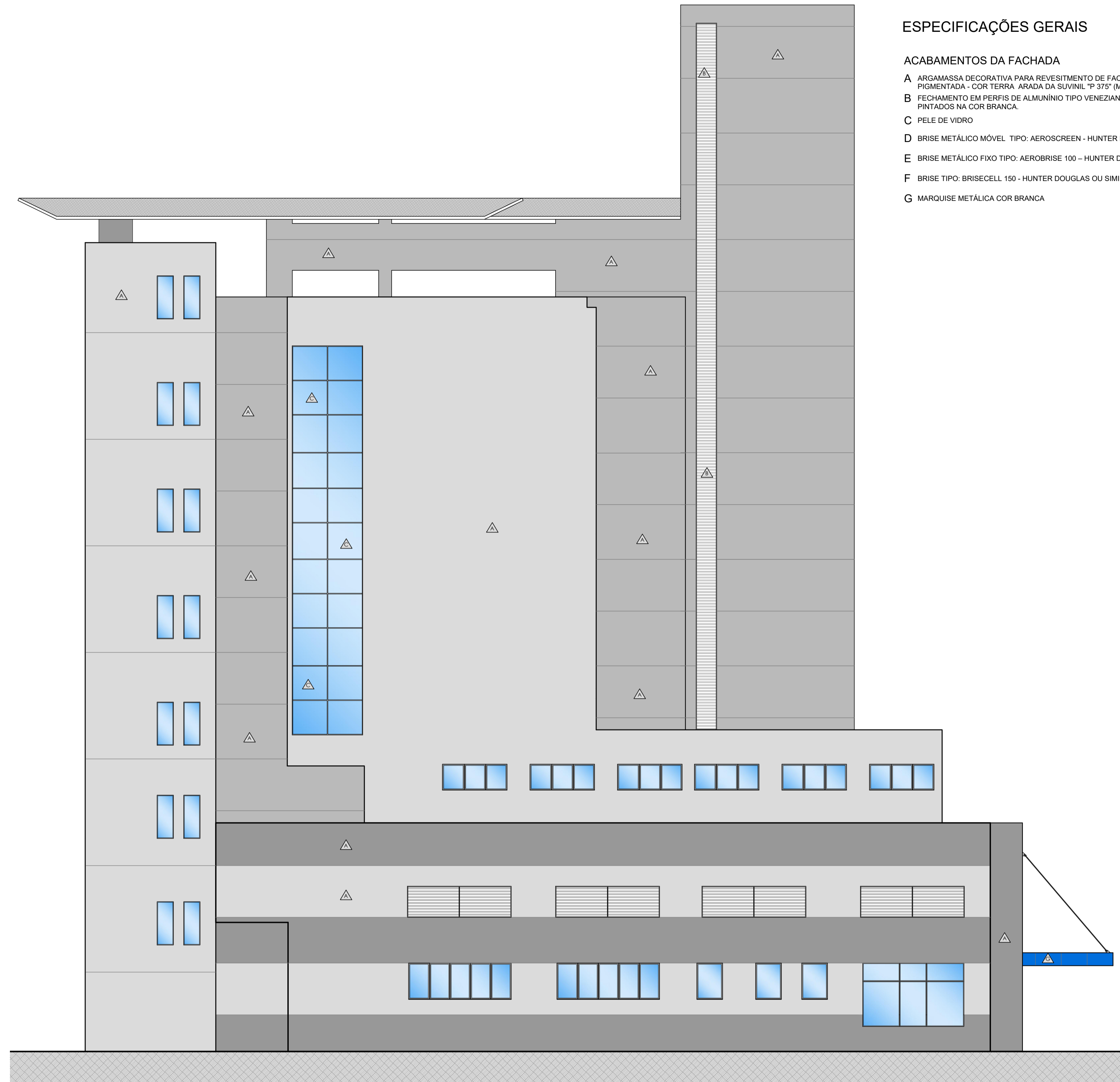
ELEVAÇÃO LATERAL
