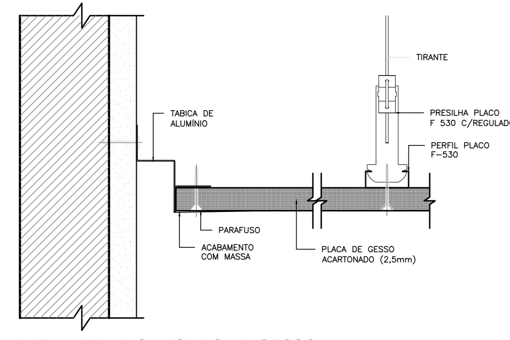
DETALHE TABICA FORRO DE GESSO ESC 1:5 MEDIDAS CM
