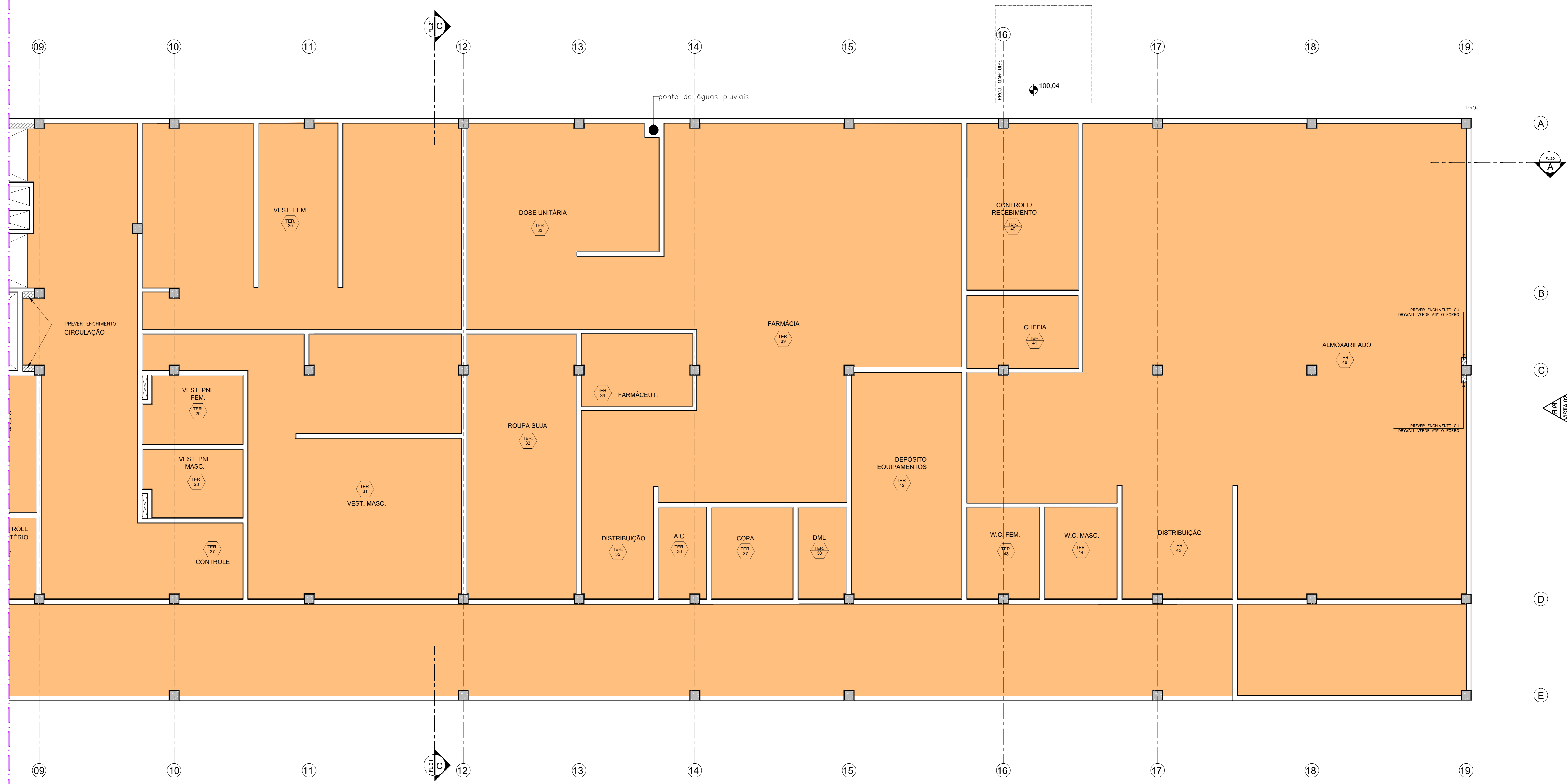
1A BLOCO 2 - PLANTA FORRO PAVIMENTO TÉRREO ESC 1:50
