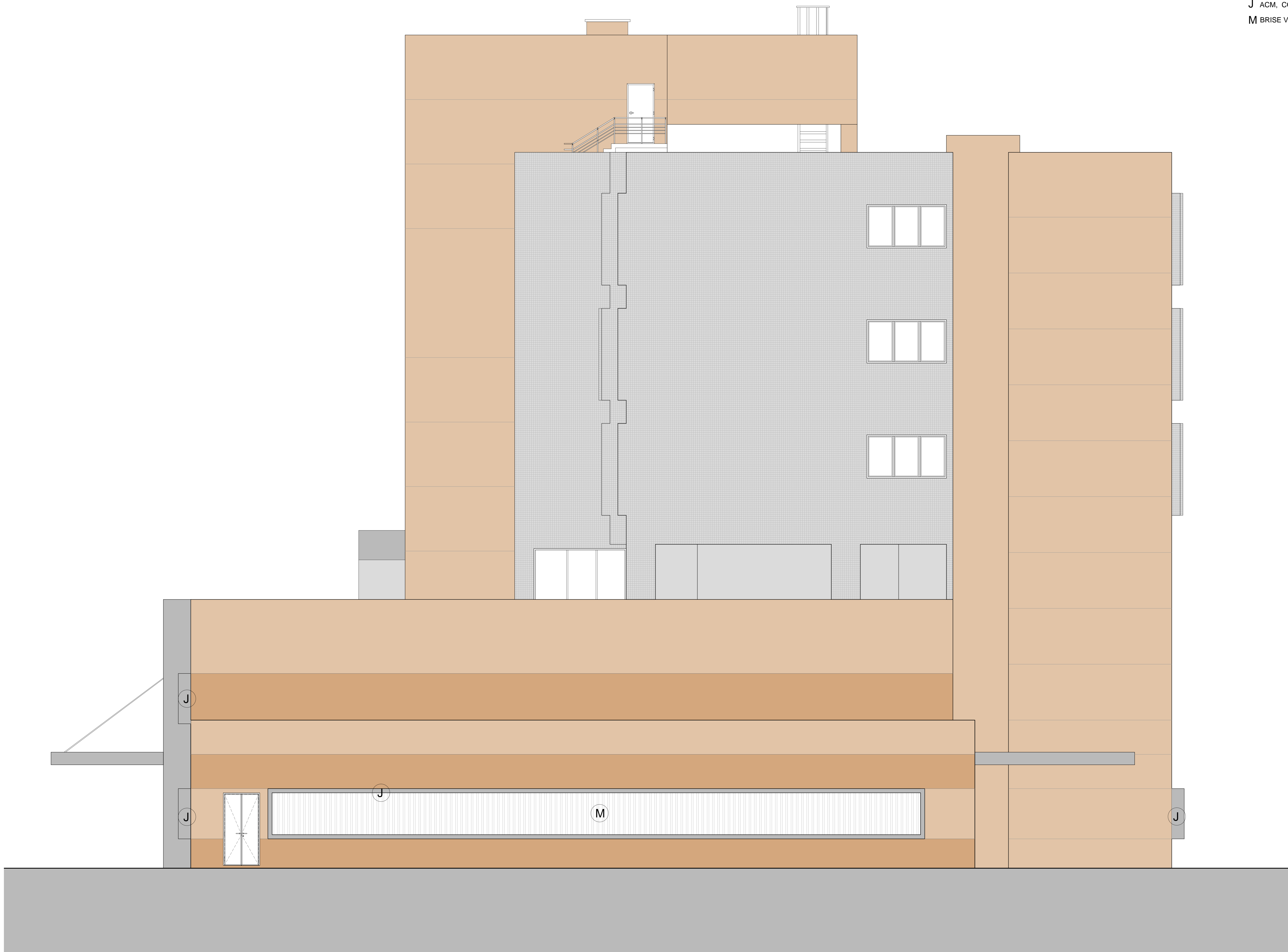
BLOCO 1 - ELEVAÇÃO 03 ESC 1:50
