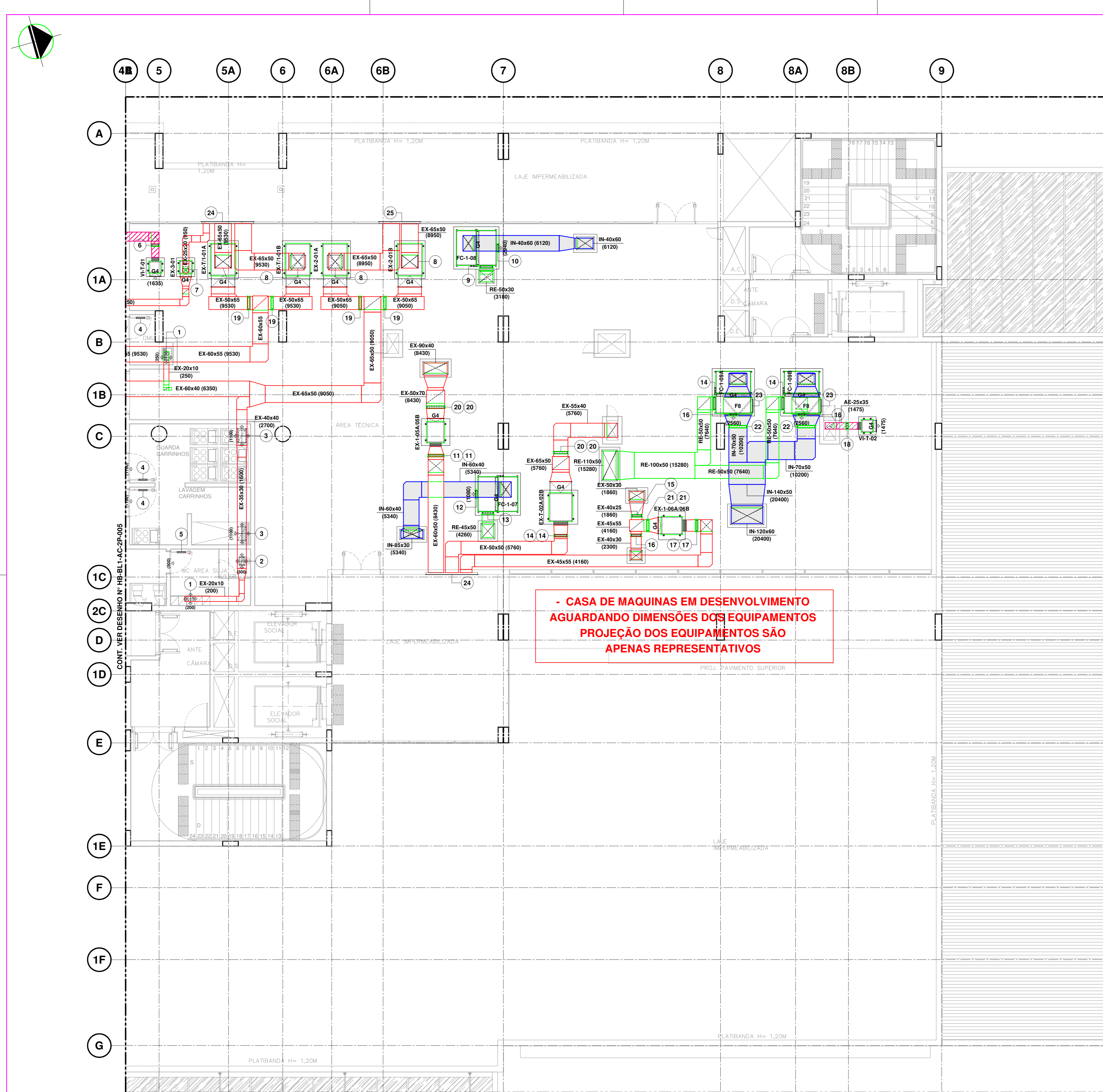
PLANTA PARCIAL DO 2º PAVIMENTO - PARTE 02/02 ESCALA 1:75
