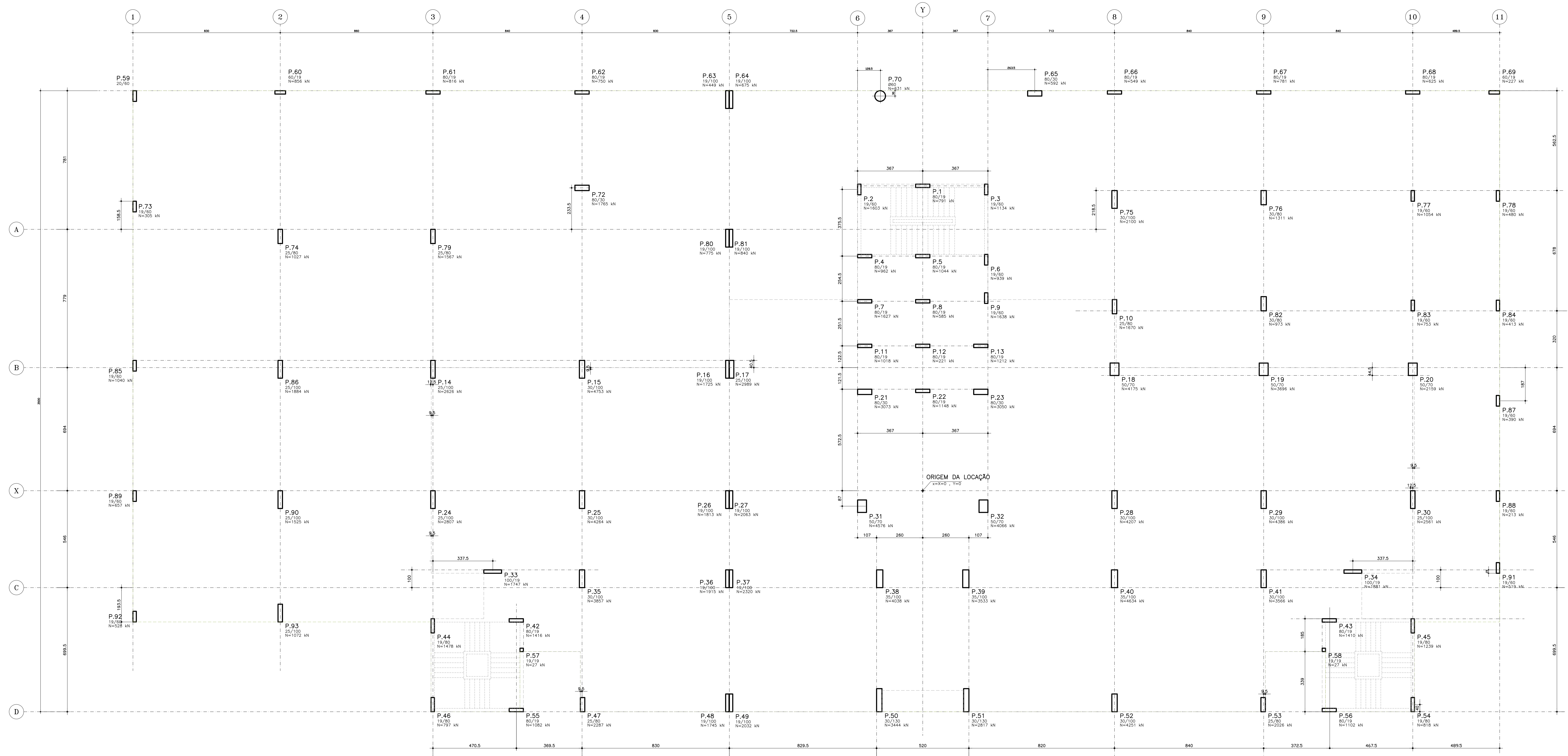
BLOCO 1 – LOCAÇÃO DOS PILARES E CARGAS NAS FUNDAÇÕES ESCALA 1/75
