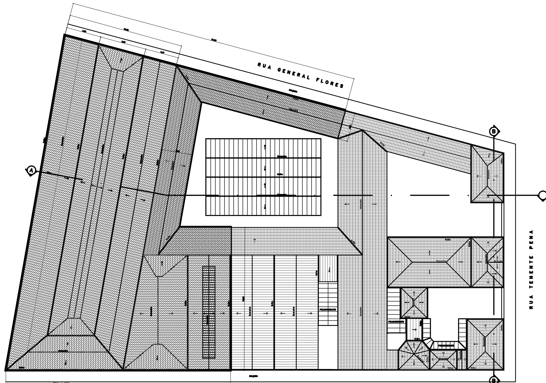
ESQ. 1:200 RUA DOS ITALIANOS PLANTA DA COBERTURA- ÁREA A SER REFORMADA
