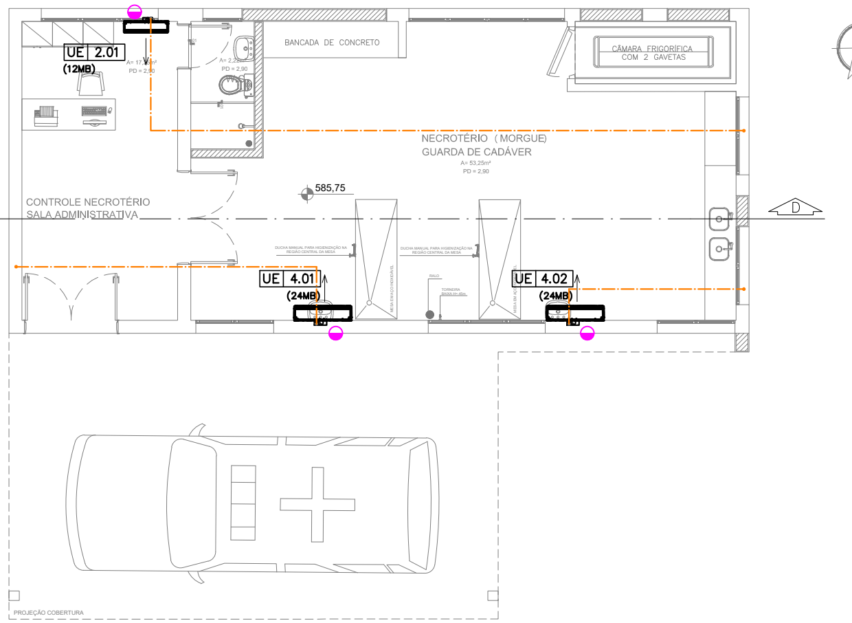
PLANTA BAIXA MORGUE ESCALA 1:75
