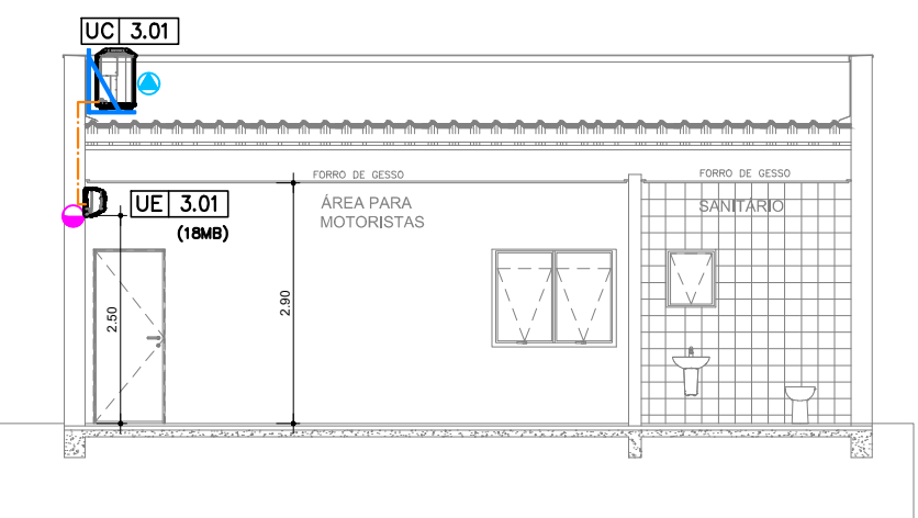
CORTE CC - AMBULÂNCIAS ESC.: 1:75
