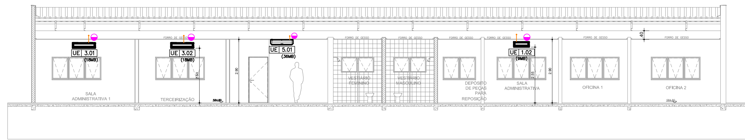
CORTE AA - TERCEIRIZAÇÃO/MANUTENÇÃO ESC.: 1:75
