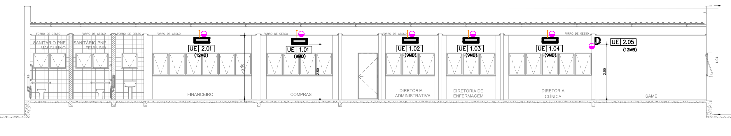
CORTE AA - ADMINISTRATIVO ESC.: 1:75
