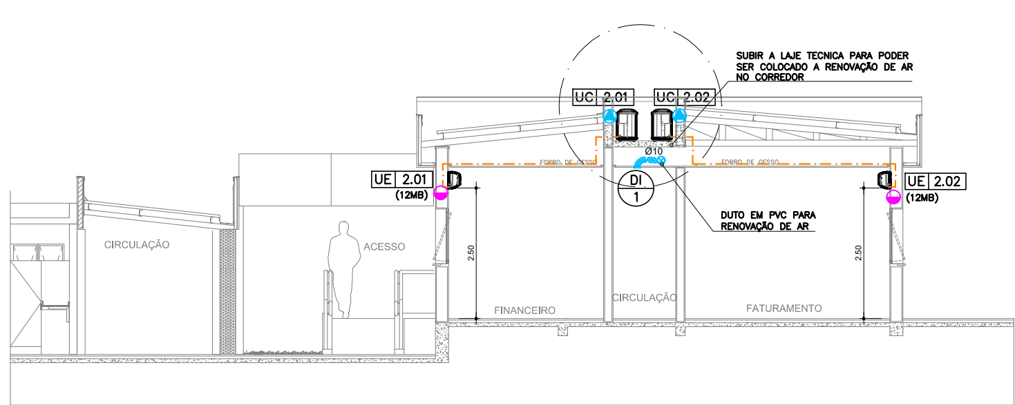
CORTE BB - ADMINISTRATIVO ESC.: 1:75
