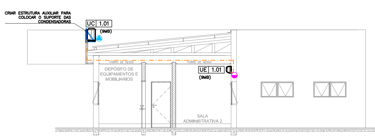
CORTE FF - TERCEIRIZAÇÃO/MANUTENÇÃO ESCALA 1:75
