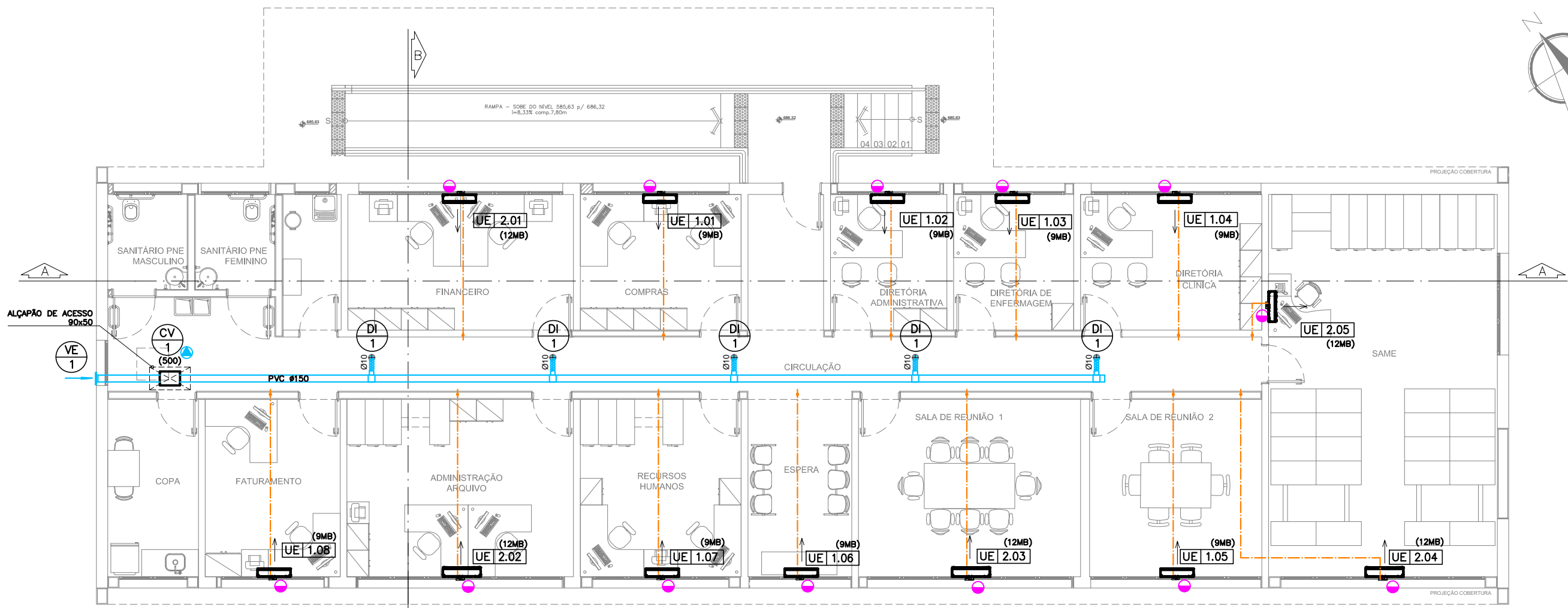
PLANTA BAIXA - ADMINISTRATIVO ESC.: 1:75
