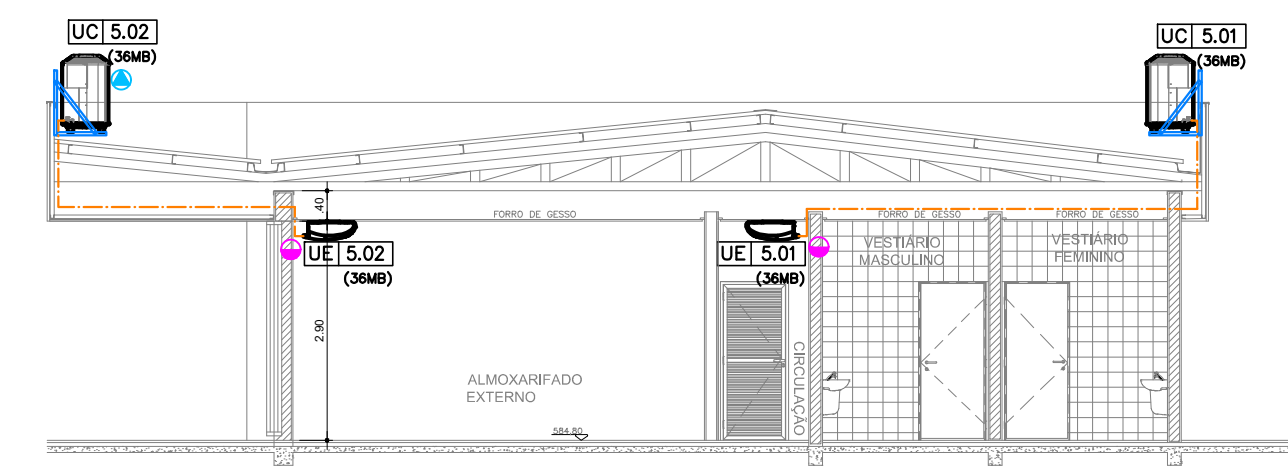
CORTE BB - TERCEIRIZAÇÃO/MANUTENÇÃO ESCALA 1:75
