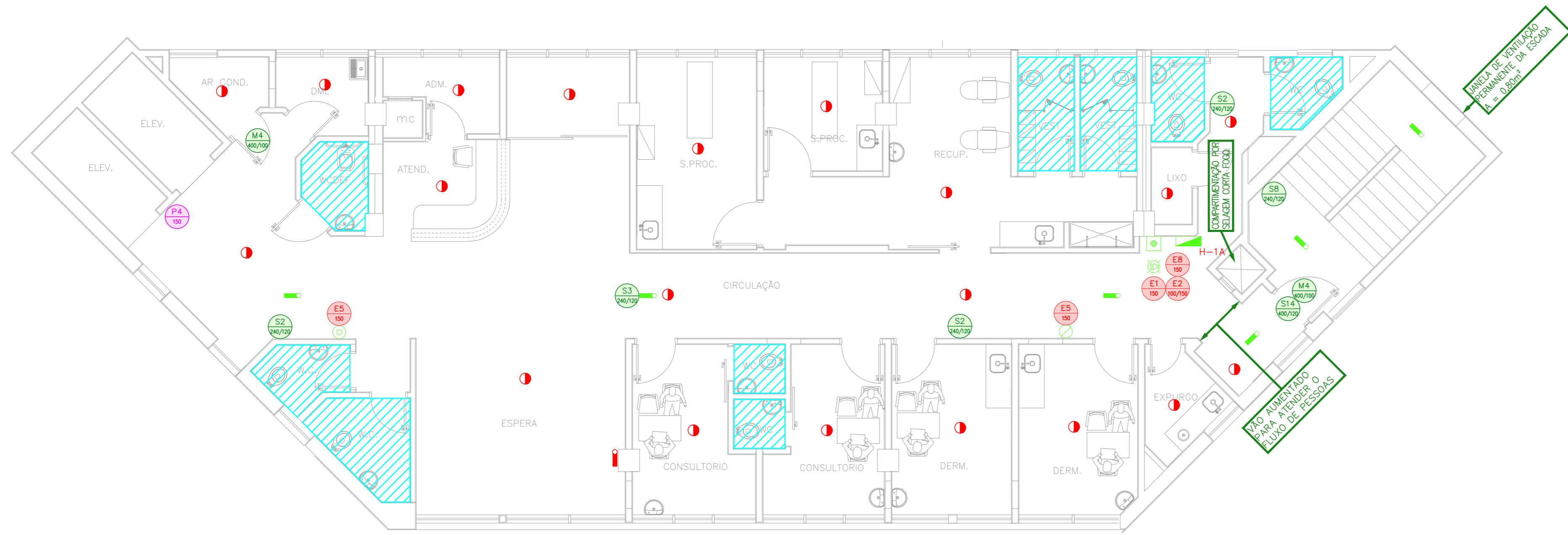
1 HOSPITAL IPIRANGA - AMBULATÓRIO PROJETO BÁSICO DOS SISTEMAS DE INCÊNDIO PLANTA BAIXA - 5ª PAVIMENTO ESCALA: 1:75 METRO
