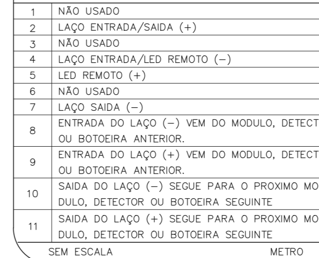
HIDRANTE SIMPLES AÇIONAMENTO AUTOMÁTICO
