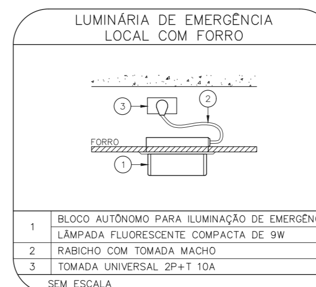
LUMINÁRIA DE EMERGÊNCIA LOCAL COM FORRO
