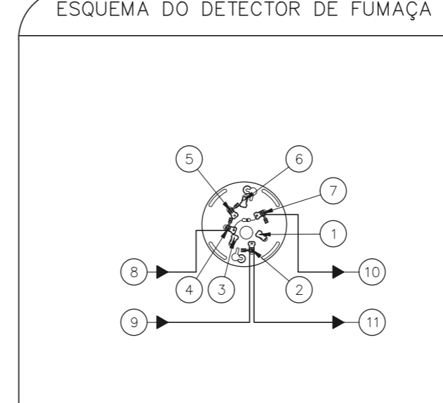
ESQUEMA DO DETECTOR DE FUMAÇA
