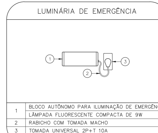
LUMINÁRIA DE EMERGÊNCIA
