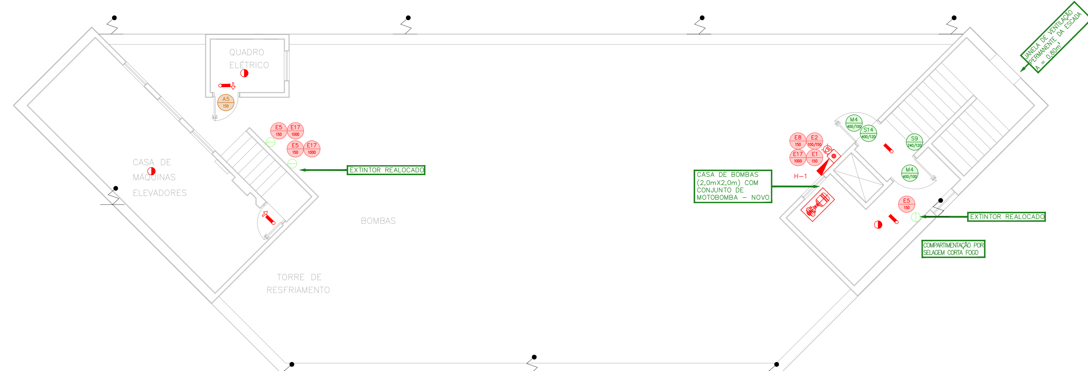
2 HOSPITAL IPIRANGA - AMBULATÓRIO PROJETO BÁSICO DOS SISTEMAS DE INCÊNDIO PLANTA BAIXA - CASA DE MÁQUINAS ESCALA: 1:75 METRO
