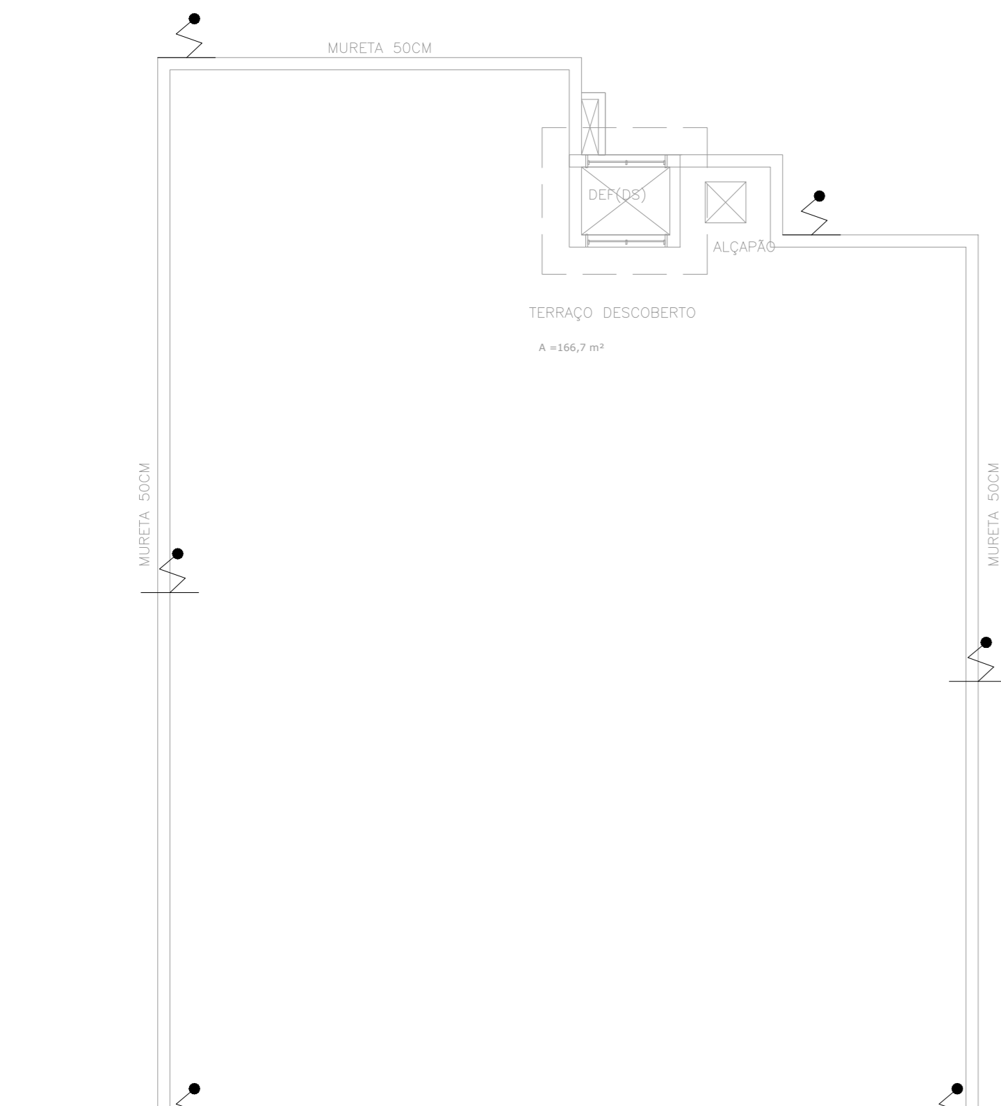
3 HOSPITAL IPIRANGA - AMBULATÓRIO PROJETO BÁSICO DOS SISTEMAS DE INCÊNDIO PLANTA BAIXA - COBERTURA ESCALA: 1:75 METRO
