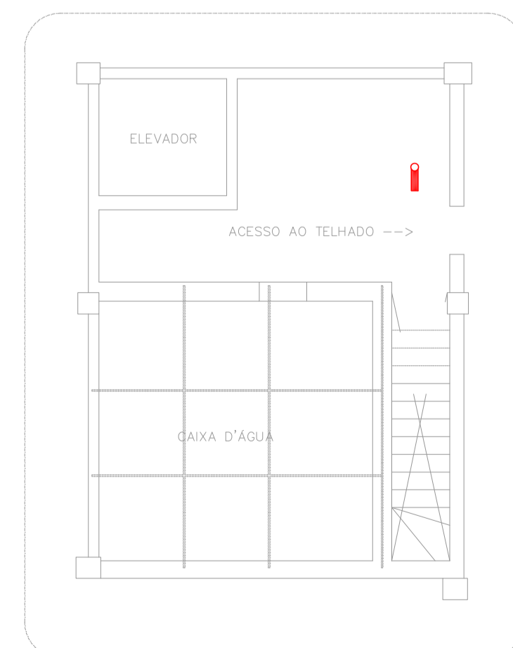
2 CRATOD BOM RETIRO PROJETO BASEADO NOS SISTEMAS DE INCÊNDIO PLANTA BAIXA - RESERVATÓRIO E CASA DE MÁQUINAS ESCALA 1:75 METRO
