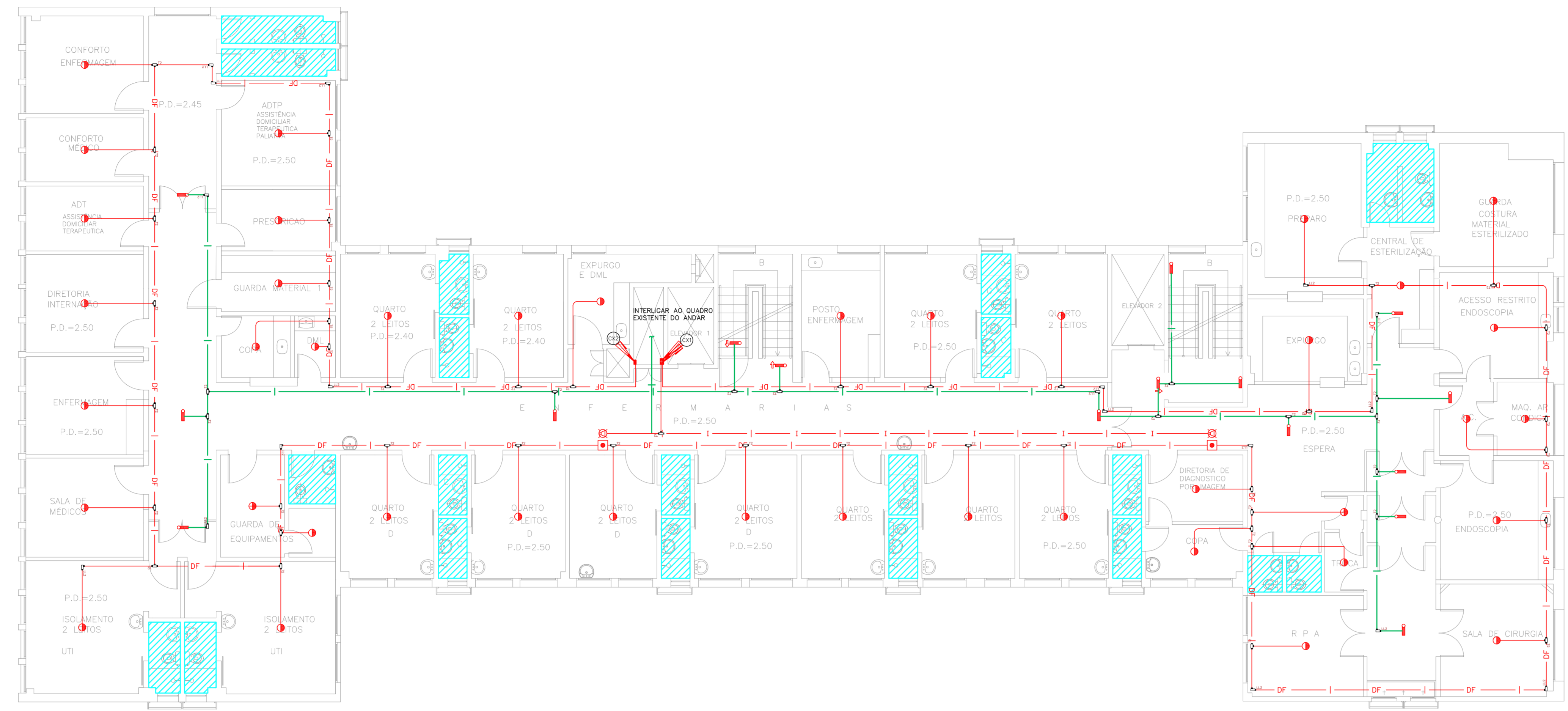
1 CRT/DST - AIDS PROJETO BÁSICO DOS SISTEMAS DE INCÊNDIO PLANTA BAIXA - 3º PAVIMENTO ESCALA 1:100 METRO
