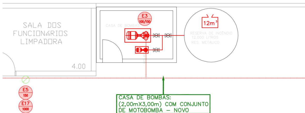
Figura 6 – PAVIMENTO INFERIOR – Alvenaria casa de bombas
