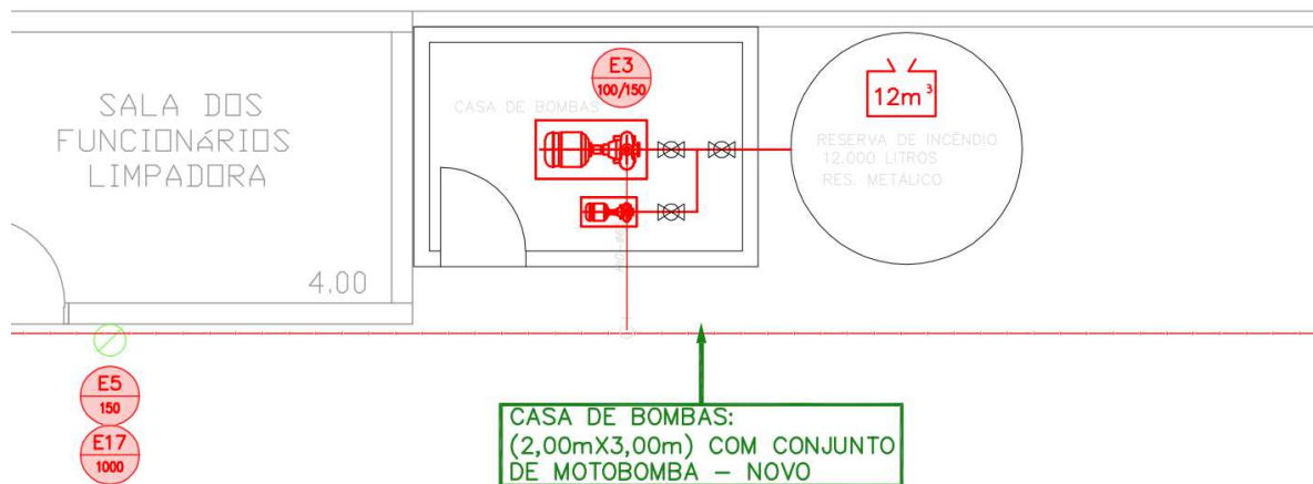
Figura 7 – RESERVA DE INCÊNDIO E CASA DE BOMBAS - Layout
