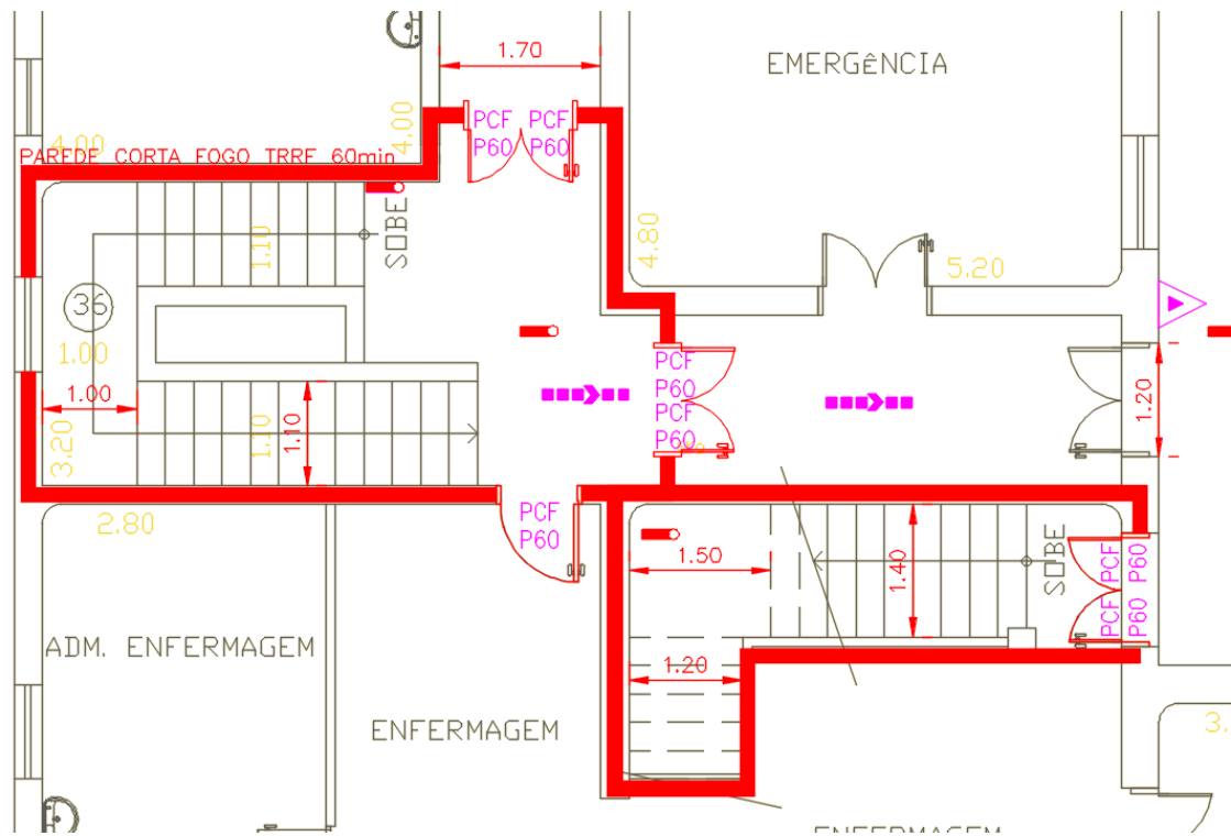
Figura 3 – PAVIMENTO TÉRREO – Instalação de portas corta-fogo
