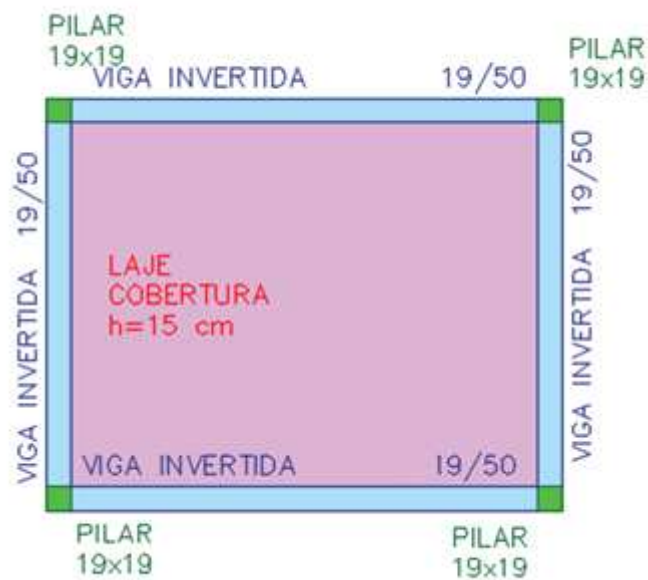
Figura 06 - CASA DE BOMBAS - PLANTA ESTRUTURAL DA COBERTURA
