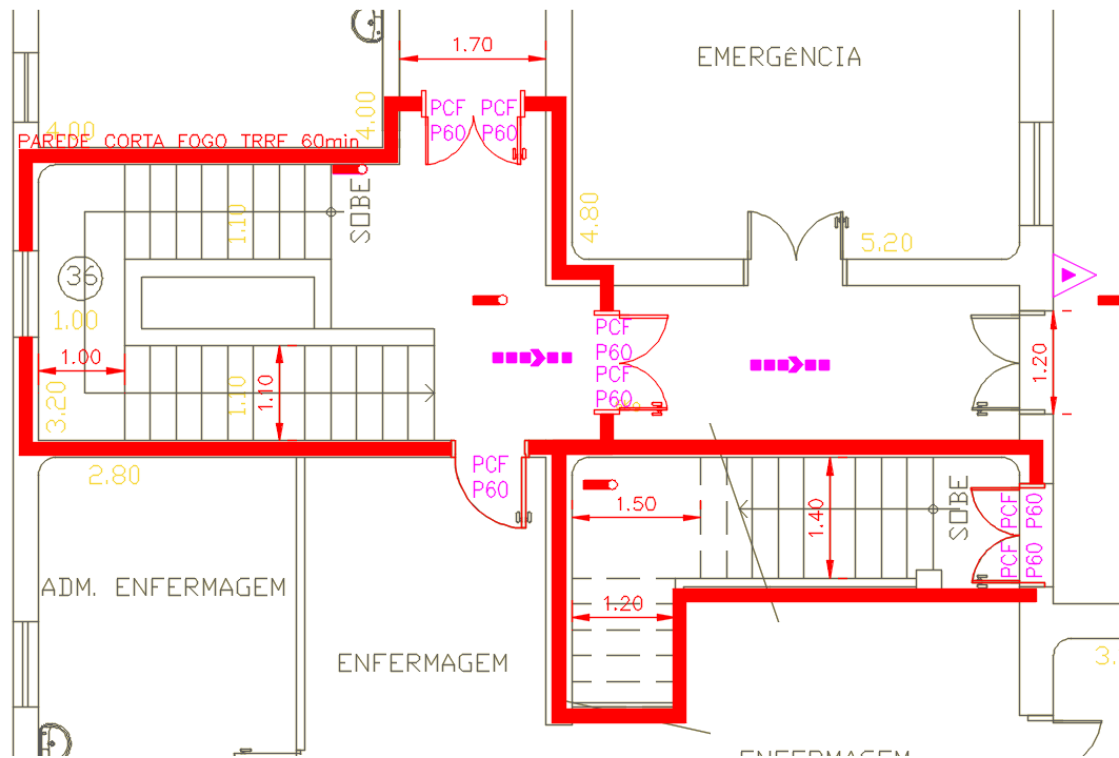
Figura 5 – PAVIMENTO TÉRREO – Instalação de portas corta-fogo
