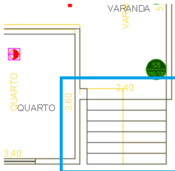
Figura 35 – PAVILHÃO 11 – Ampliação da escada existente – Escada existente (amarelo) x nova escada
