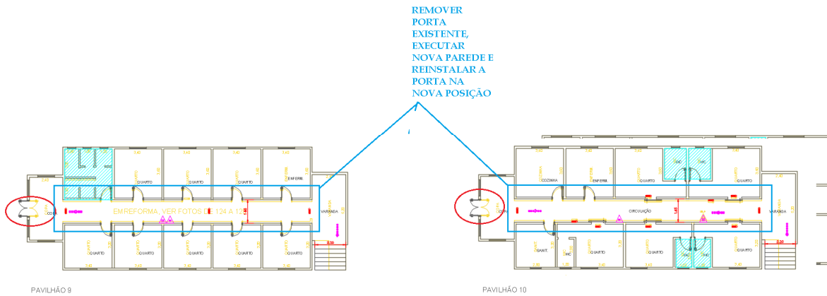
Figura 12 – PAVILHÃO 09 e 10 – Reposicionamento/instalação e inversão portas
