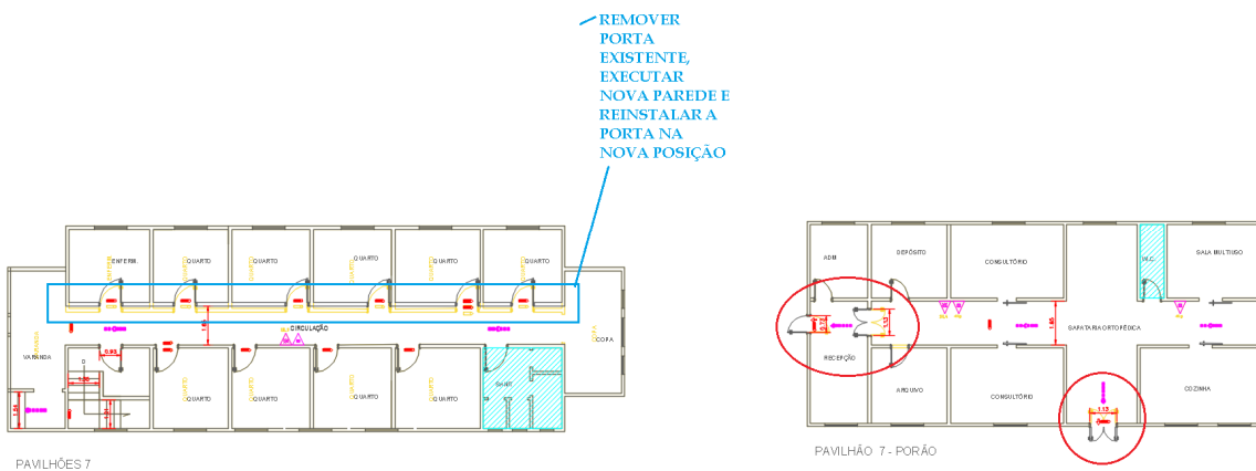
Figura 10 – PAVILHÃO 07 – Reposicionamento/instalação e inversão portas
