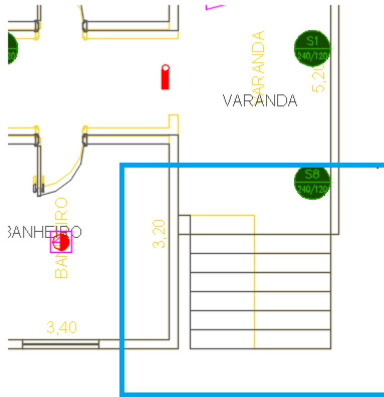
Figura 29 – PAVILHÃO 2 – Ampliação da escada existente – Escada existente (amarelo) x nova escada
