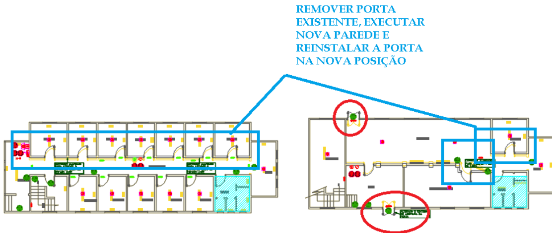
Figura 8 – PAVILHÃO 03 – Reposicionamento/instalação e inversão portas
