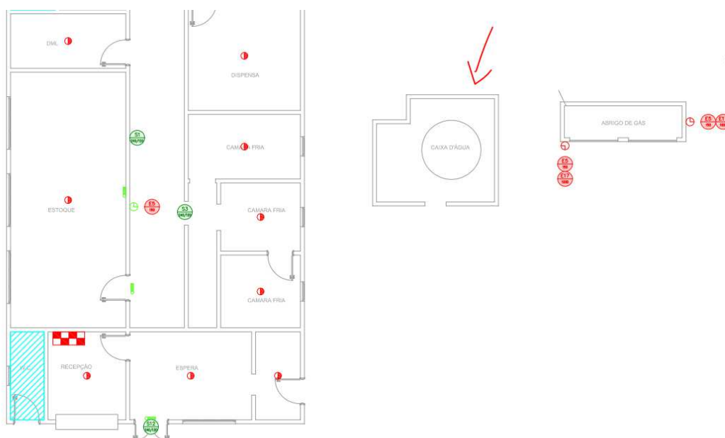
Figura 36 – HFRA/REFEITÓRIO - NOVO RESERVATÓRIO - Layout
