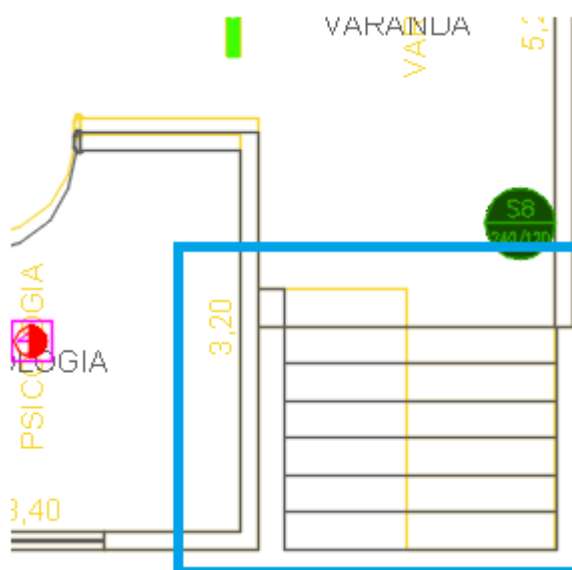
Figura 32 – PAVILHÃO 8 – Ampliação da escada existente – Escada existente (amarelo) x nova escada
