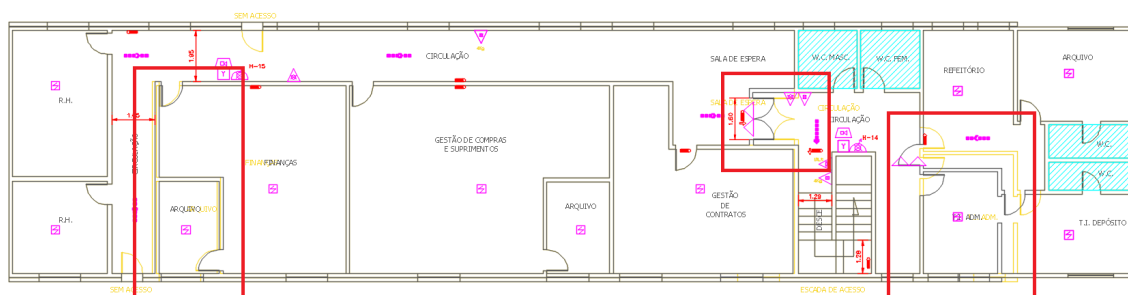
Figura 17 – MEZANINO –Demolição/reconstrução paredes
