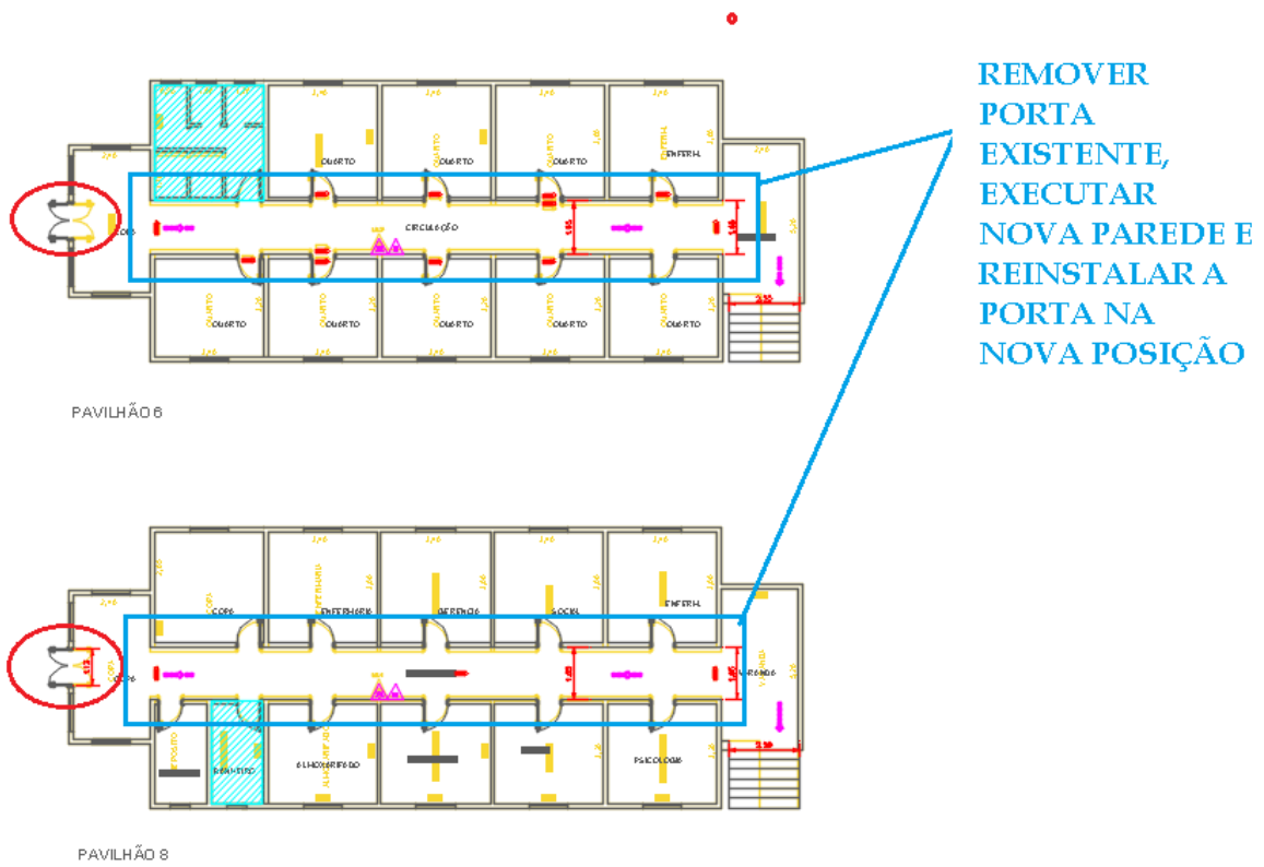
Figura 11 – PAVILHÃO 06 e 08 – Reposicionamento/instalação e inversão portas
