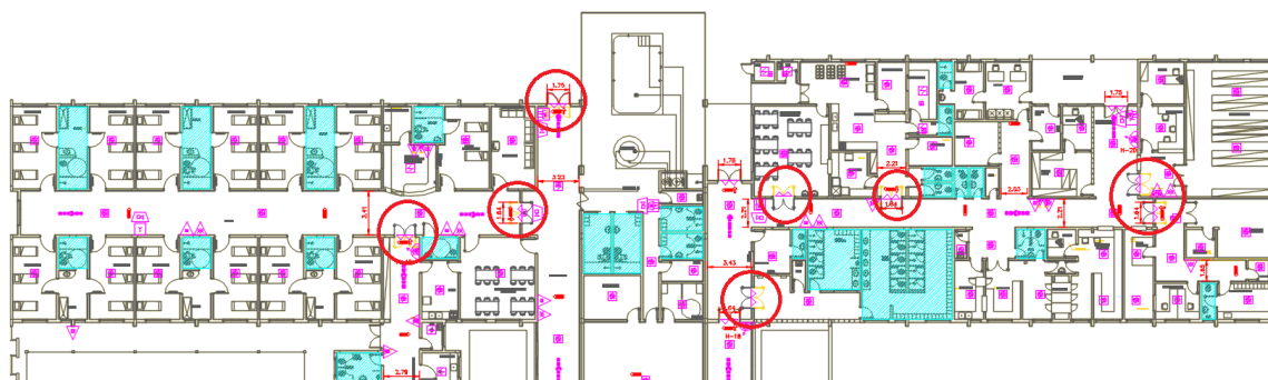
Figura 1 – PAVIMENTO TÉRREO- PRÉDIO PRINCIPAL – Inversão sentido de porta
