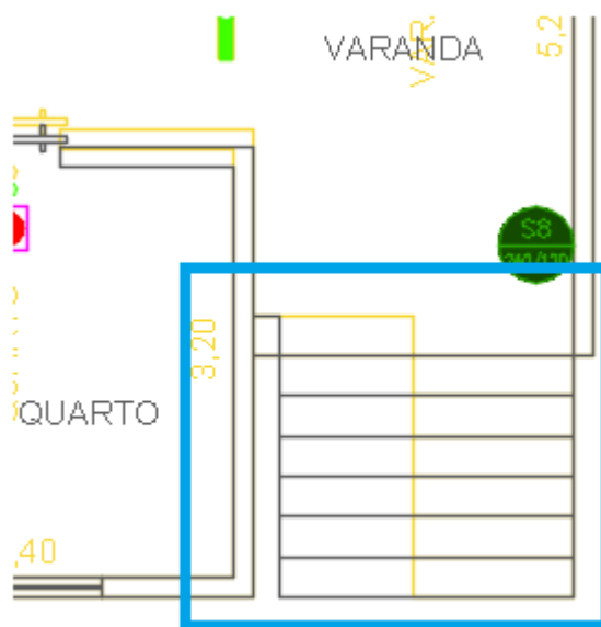
Figura 34 – PAVILHÃO 10 – Ampliação da escada existente – Escada existente (amarelo) x nova escada
