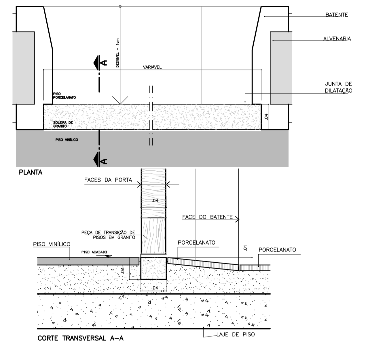
DETALHE TRANSIÇÃO DE PISOS EM RAMPA - SOLEIRA DE GRANITO ESC. 1:3
