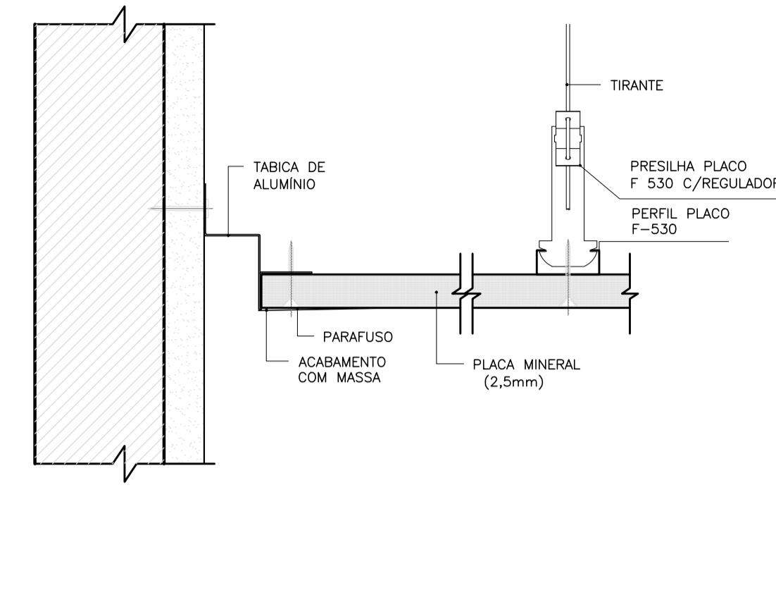
DETALHE TABICA FORRO MINERAL ESC. 1:2
