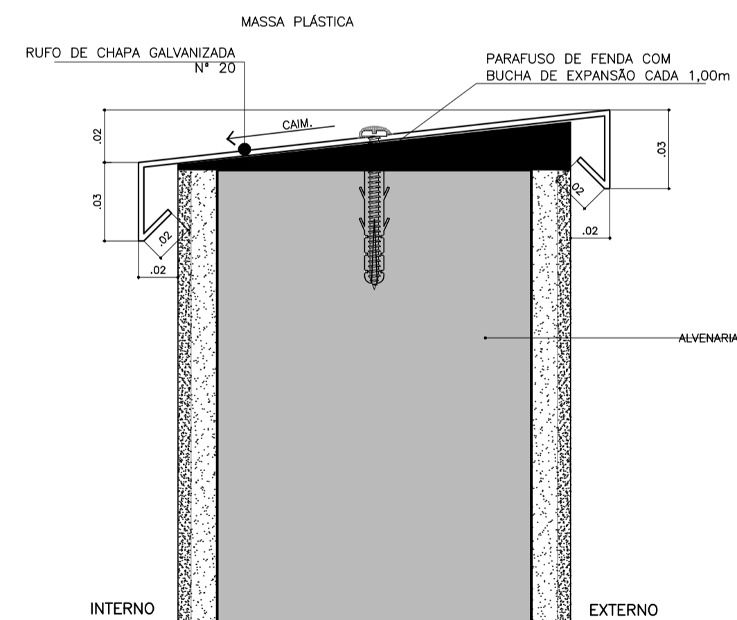
DETALHE CAPEAMENTO METÁLICO P/ PLATIBANDA ESC. 1:2
