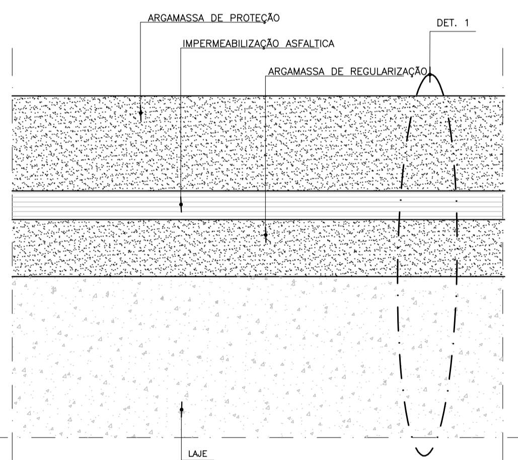
CORTE ESCALA 1:2
