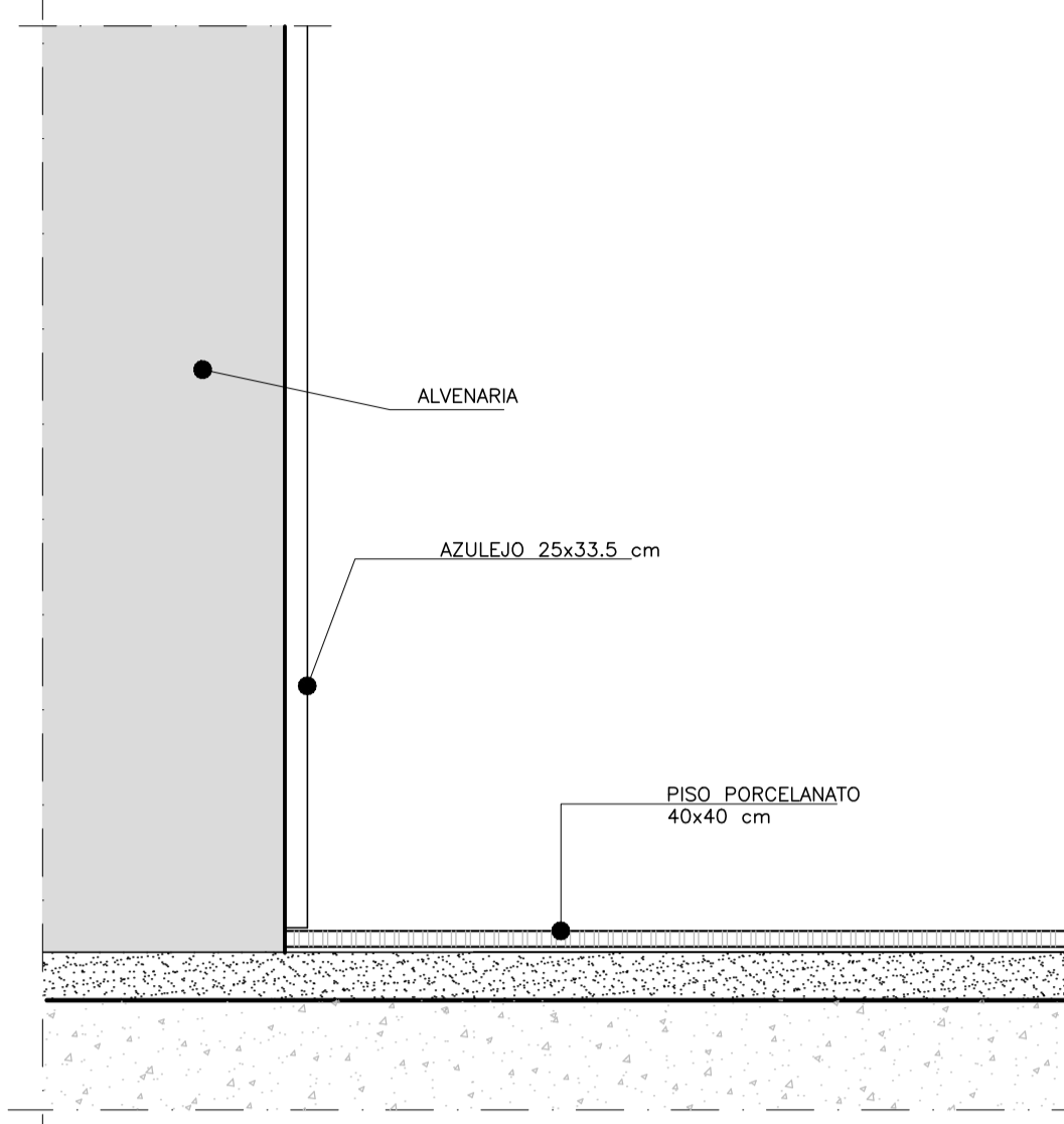
DETALHE RODAPÉ AZULEJO / PISO CERÂMICO ESC. 1:2
