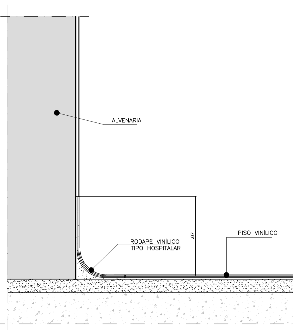
DETALHE RODAPÉ VINILICO ESC. 1:2
