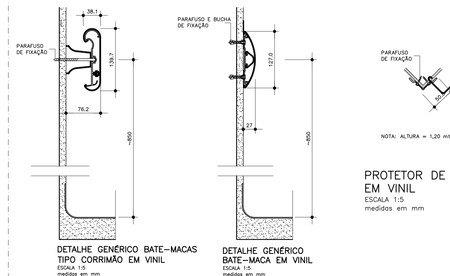
DETALHE BATE-MACAS ESC. 1:5
