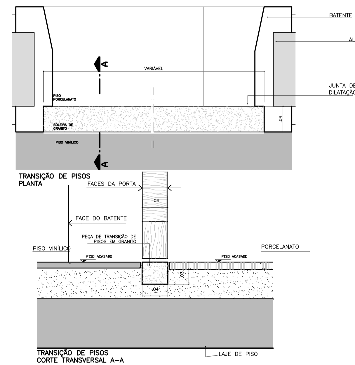
DETALHE TRANSIÇÃO DE PISOS ESC. 1:3
