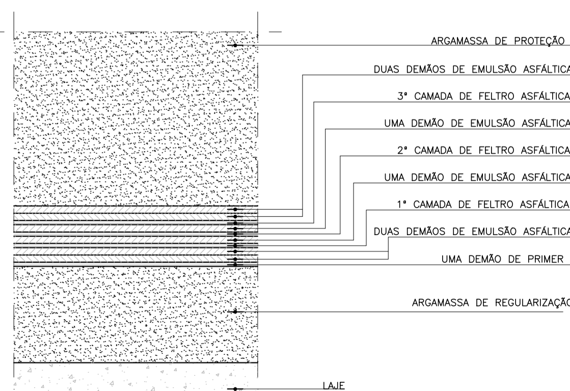
DET.1 5/ ESCALA
