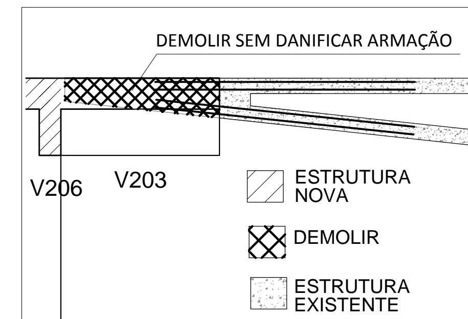
DETALHE 1 ESC: 1:25
