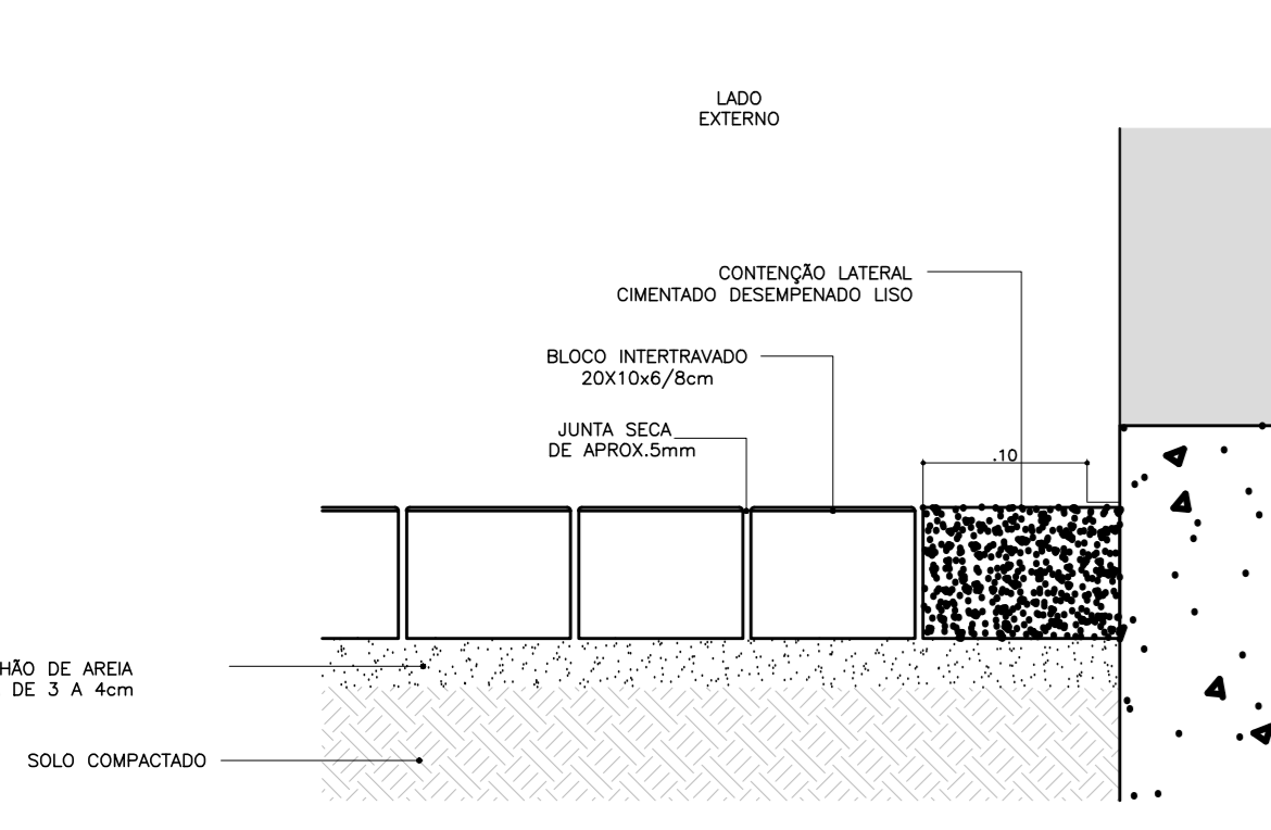
BLOCO INTERTRAVADO CORTE TRANSVERSAL ESCALA 1:5
