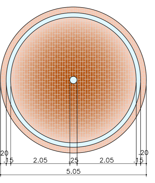
DETALHE FONTE ESC.1:75
