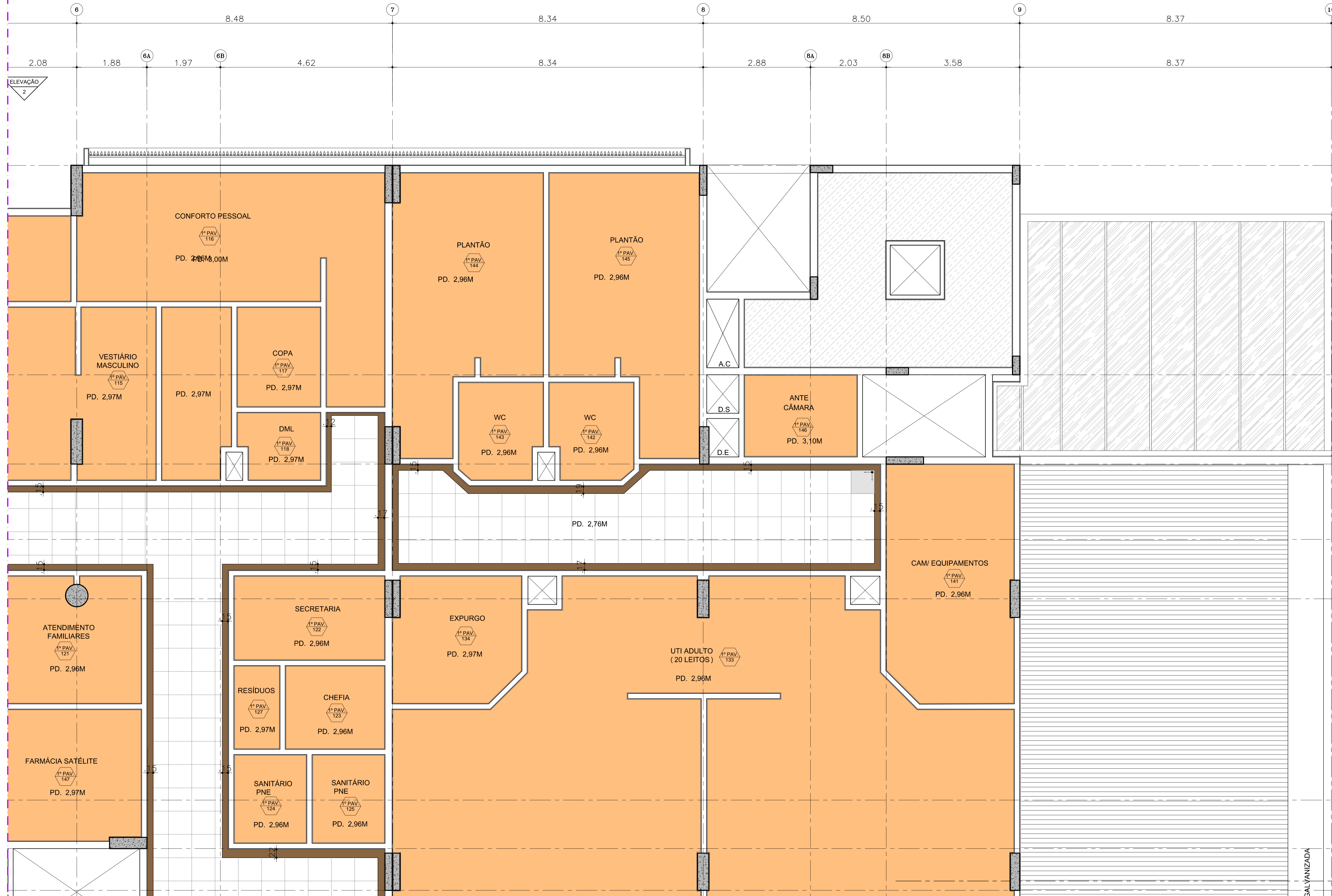
1A PLANTA FORRO BLOCO 1 - 1º PAVIMENTO ESC 1:50
