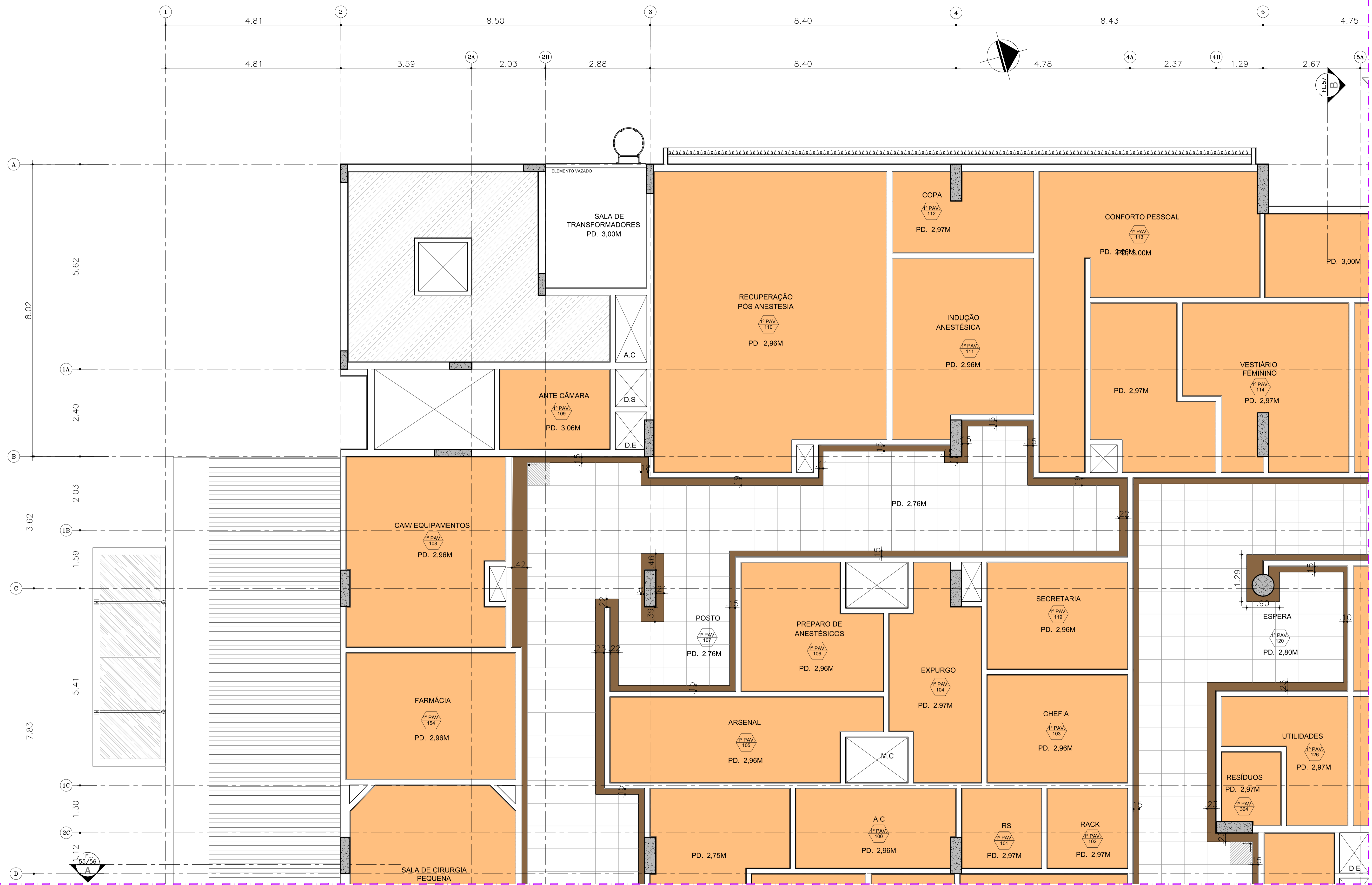
PLANTA FORRO BLOCO 1 - 1º PAVIMENTO ESC 1:50
