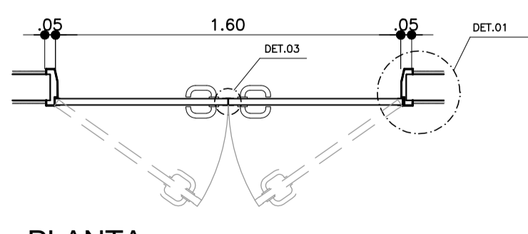
PLANTA ESC. 1:25
