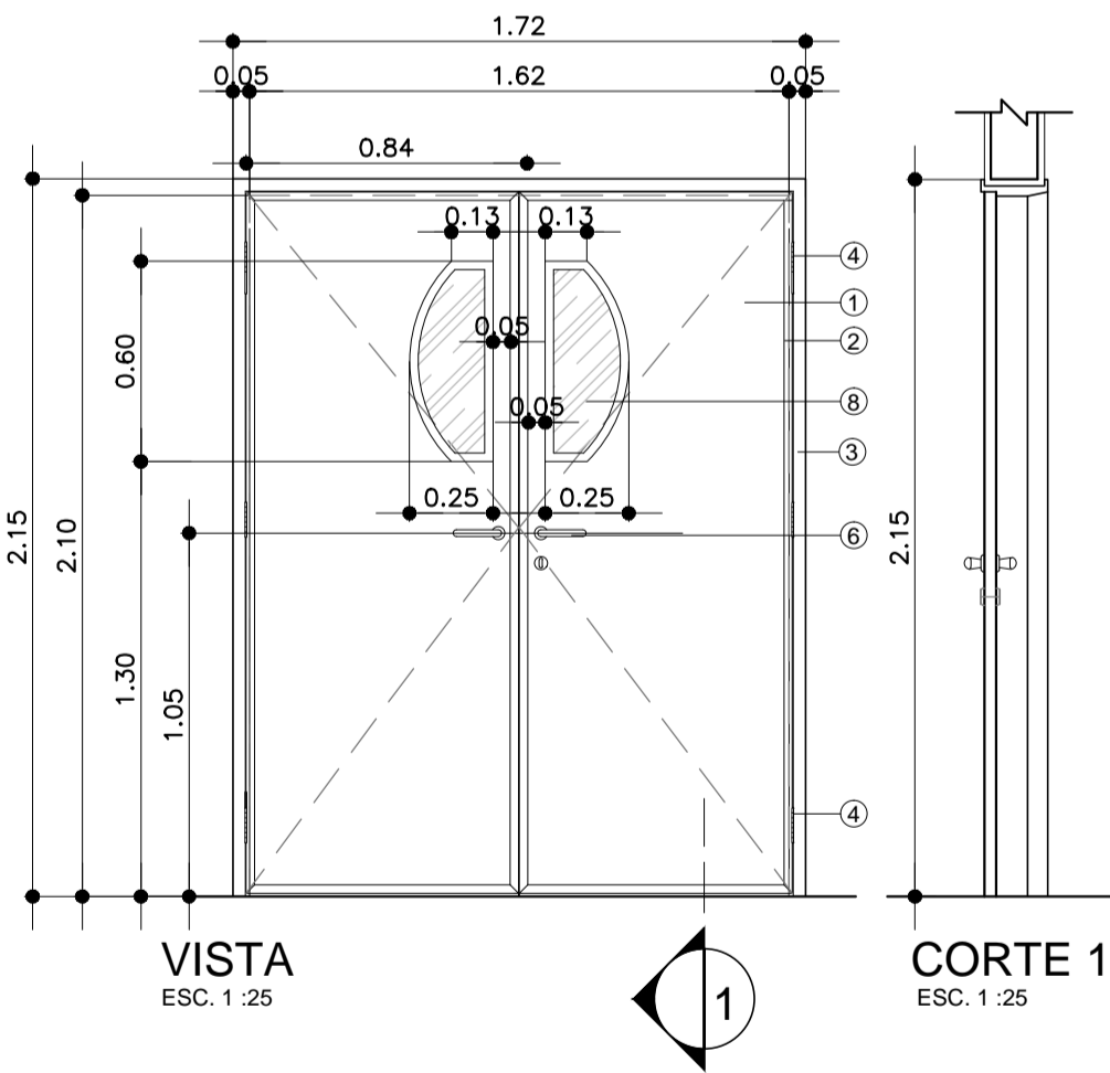
PM 06 PORTA DUPLA VAL-VEM COM VISOR QUANTIDADE: 2 UNIDADES
