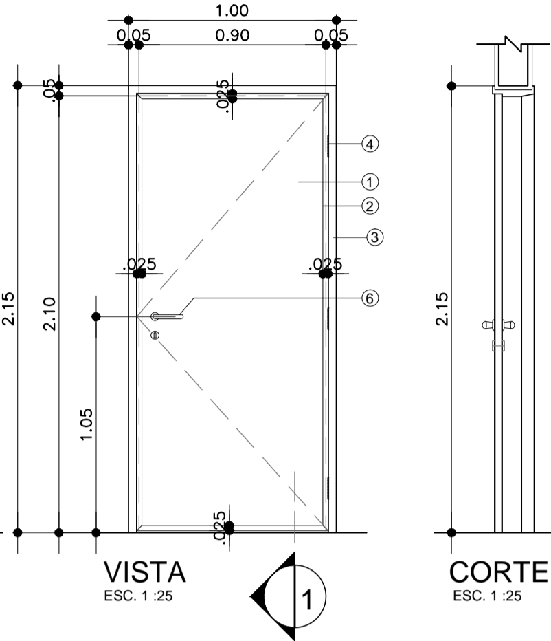
CORTE 1 ESC. 1:25
