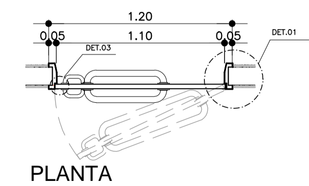
PLANTA ESC. 1:25
