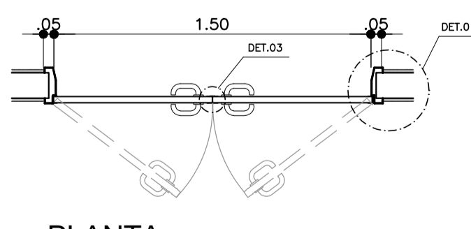
PLANTA ESC. 1:25
