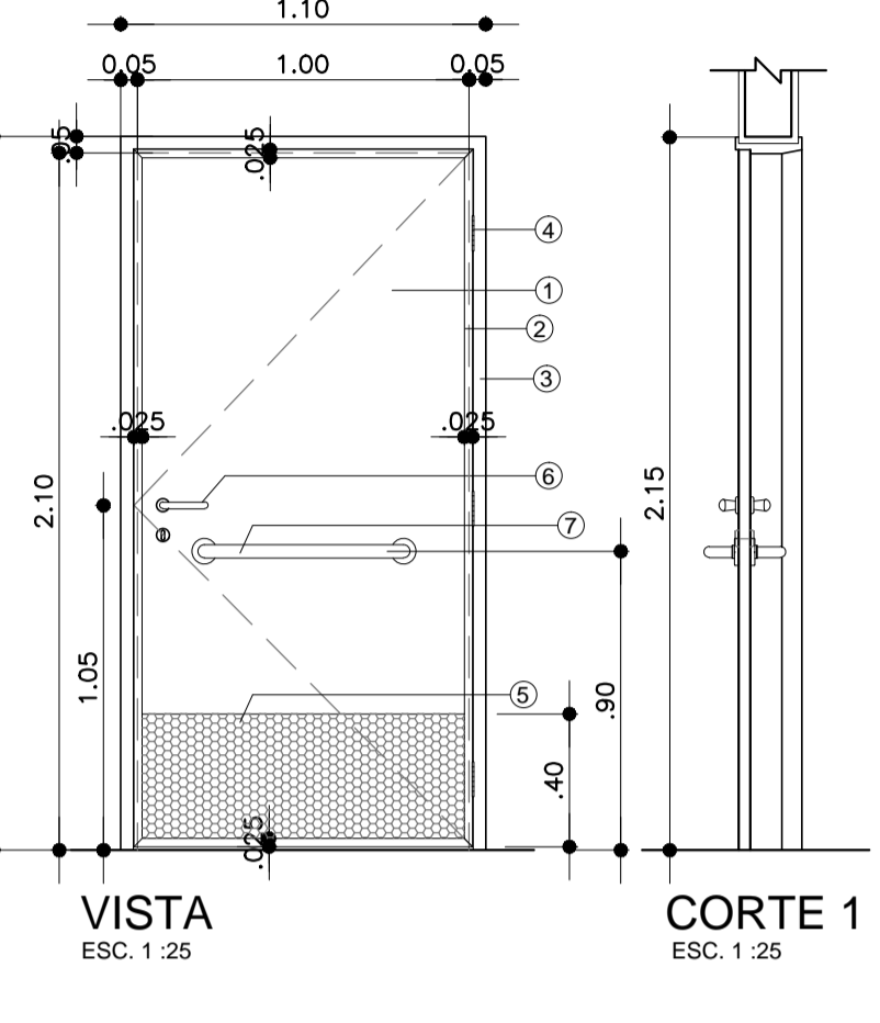
PM 11 PORTA DE MADEIRA QUANTIDADE: 02 UNIDADES
