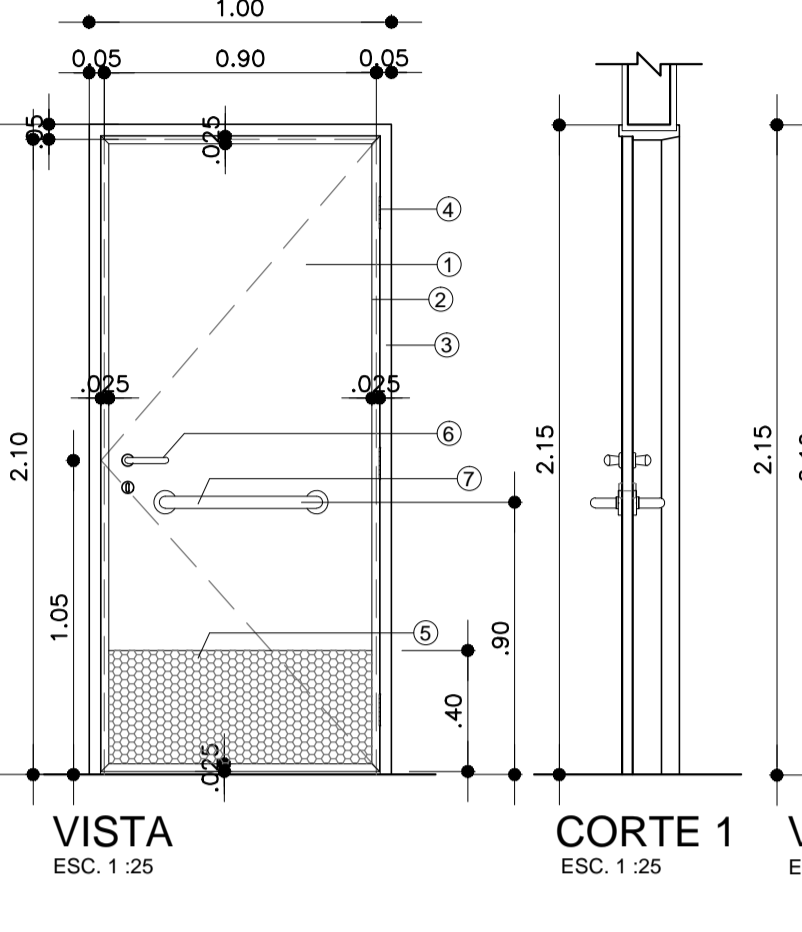
PM 04 PORTA DE MADEIRA QUANTIDADE: 04 UNIDADES
