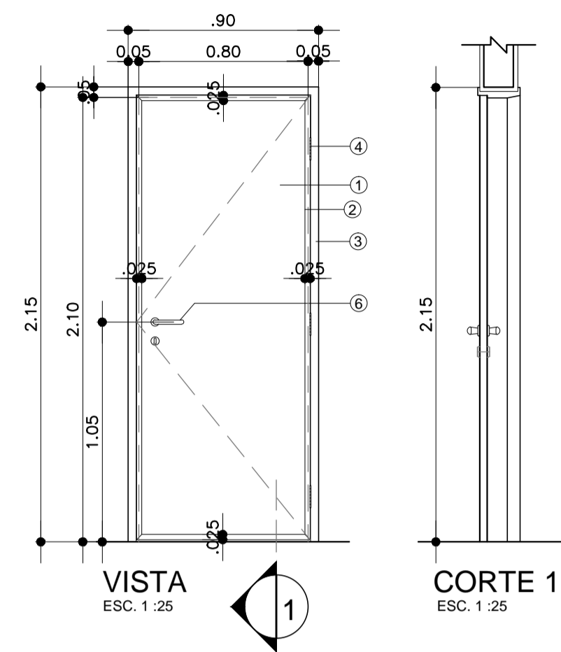
PM 02 PORTA DE MADEIRA QUANTIDADE: 04 UNIDADES
