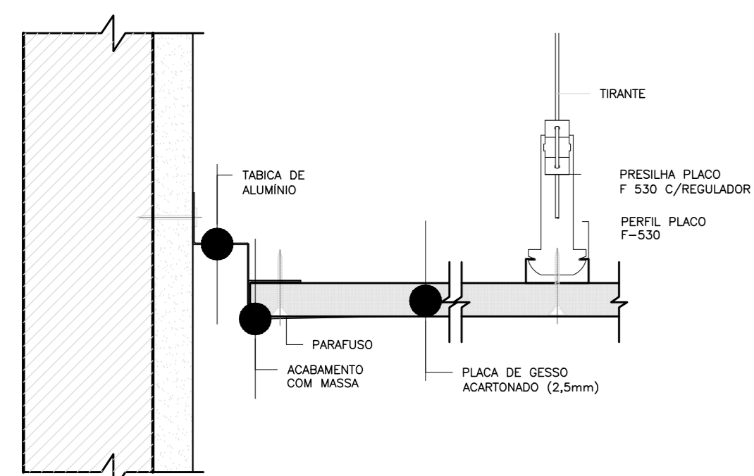
DETALHE TABICA FORRO DE GESSO ESC 1:5 M020404
