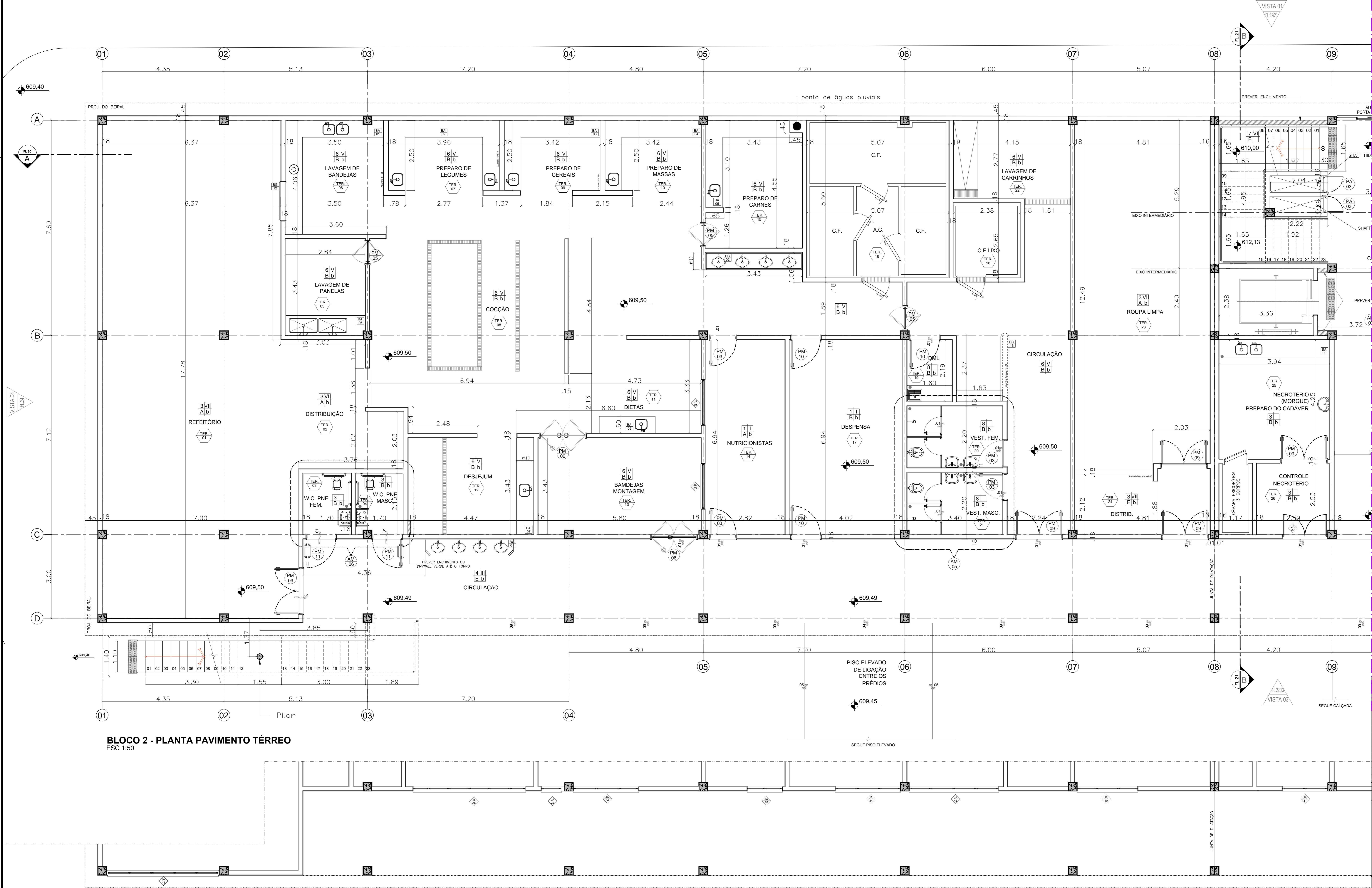
BLOCO 2 - PLANTA CAIXILHOS ESC 1:50
